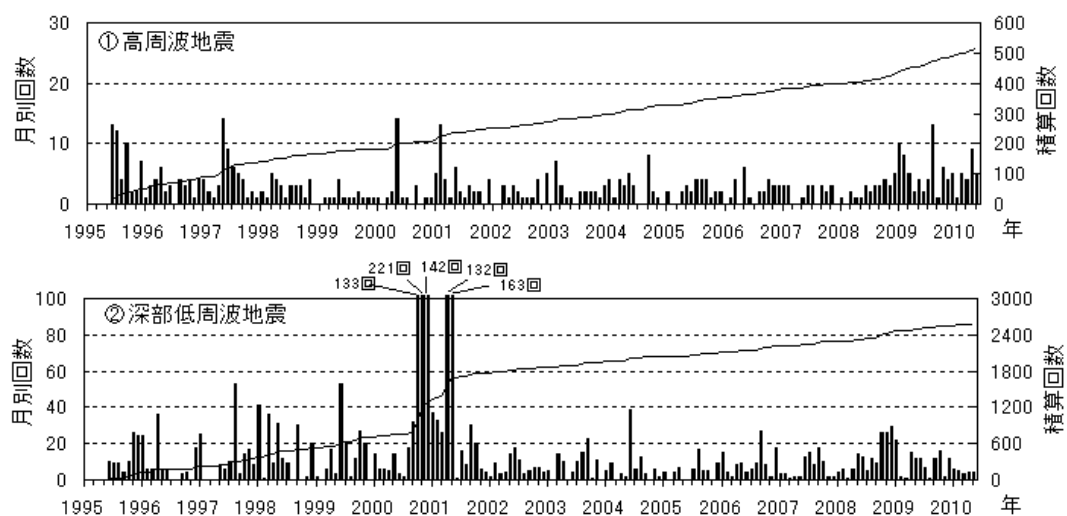
図 2※ 富士山 月別地震回数(1995 年 6 月～2010 年 5 月)
