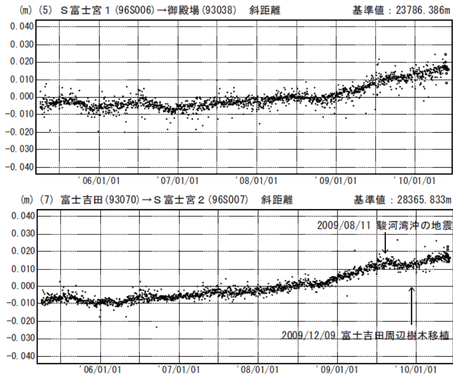
図 4 ※ 富士山 国土地理院による GPS 観測結果 1) （2005 年 4 月 1 日～2010 年 6 月 1 日）
