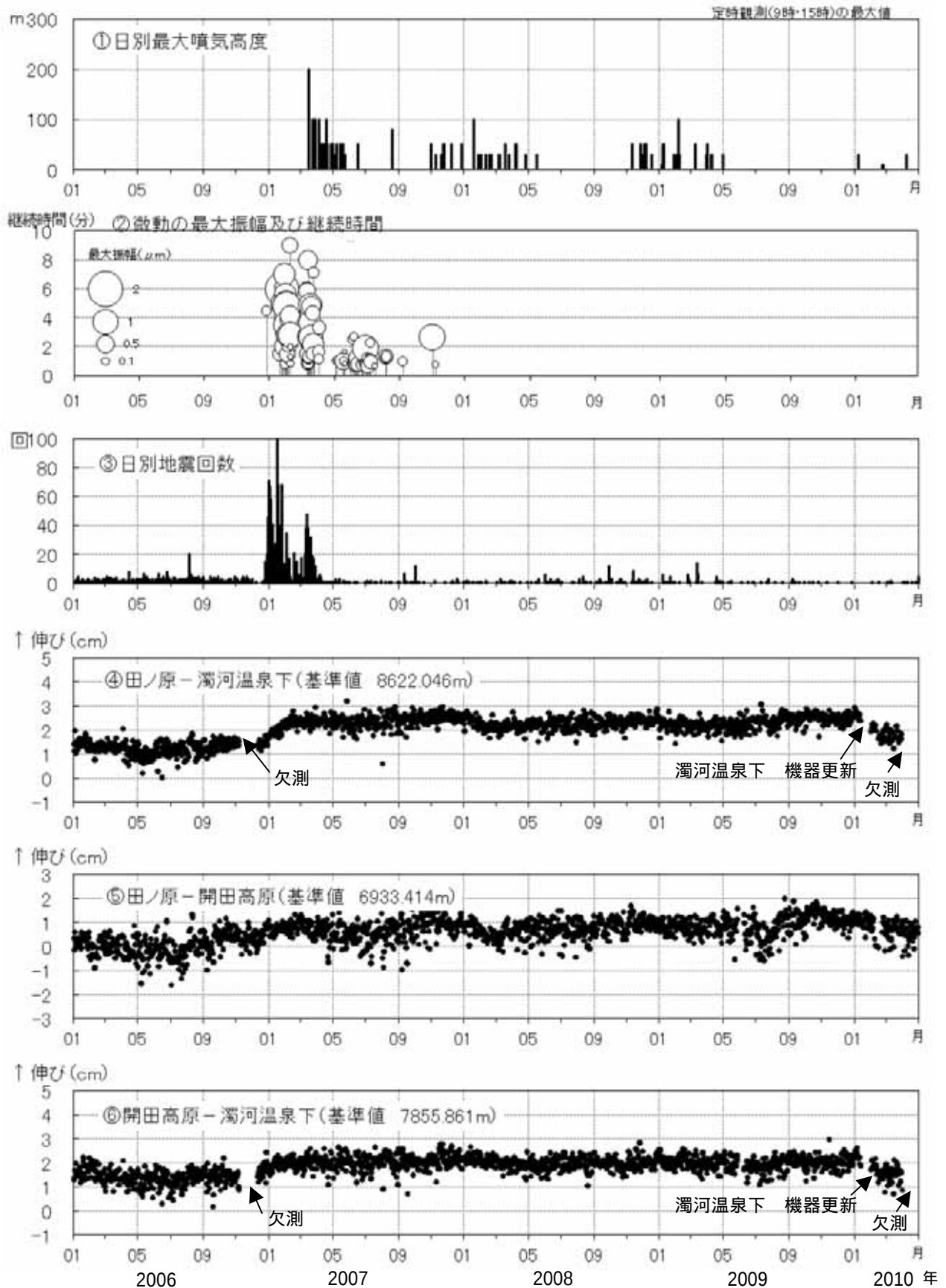
図4 御嶽山 最近の火山活動の推移(2006年1月1日~2010年4月30日)
