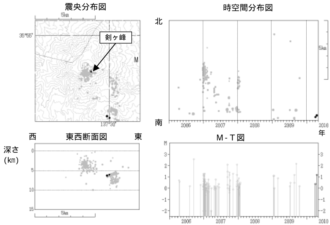
図5 御嶽山 震源分布図（2006年1月1日～2010年4月30日）
