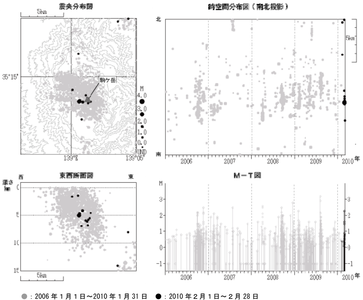
図 3※ 箱根山 震源分布図（2006 年 1 月 1 日～2010 年 2 月 28 日） M（マグニチュード）は地震の規模を表します。 図中の震源要素は一部暫定値が含まれており、後日変更することがあります。
