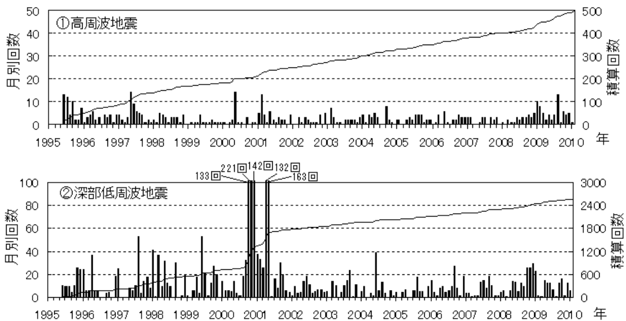
図 2※ 富士山 月別地震回数(1995 年 6 月～2010 年 2 月)
