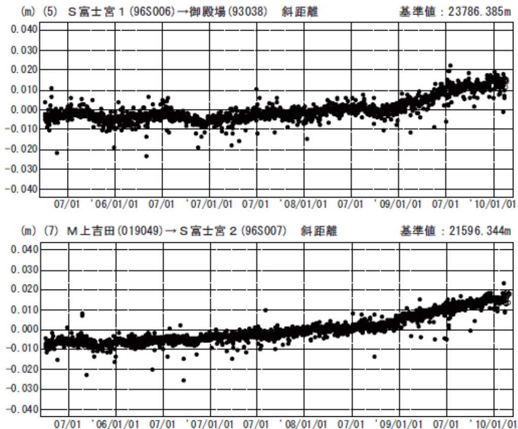
図3※ 富士山 国土地理院によるGPS観測結果 1) (2005年4月1日～2010年2月27日)
