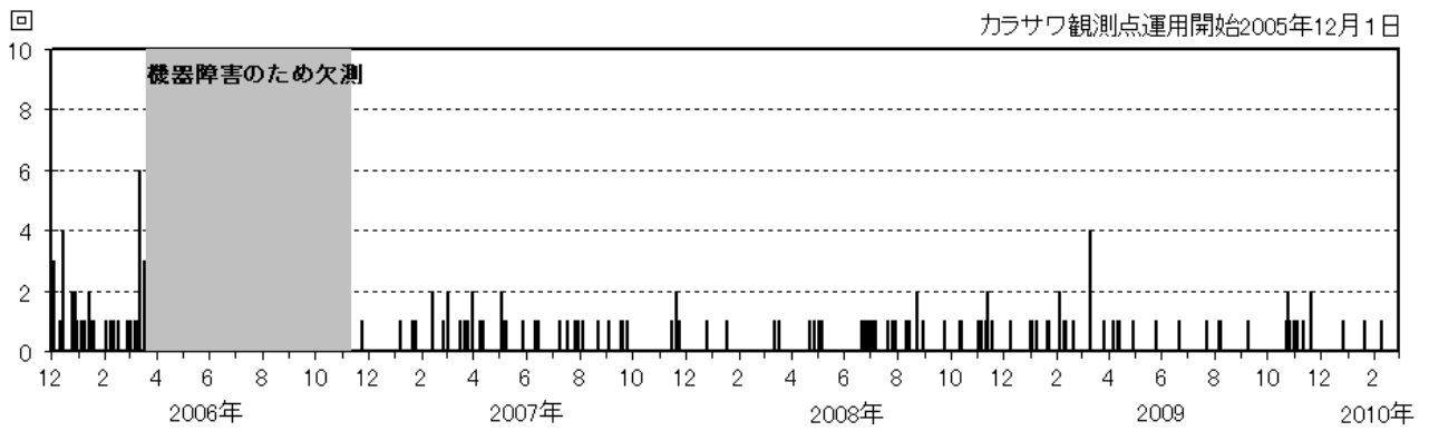
図 2 新潟焼山 日別地震回数（2005 年 12 月 1 日～2010 年 2 月 28 日）
