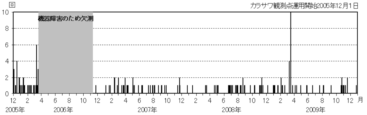
図 2 新潟焼山 日別地震回数（2005 年 12 月 1 日～2009 年 12 月 31 日）
