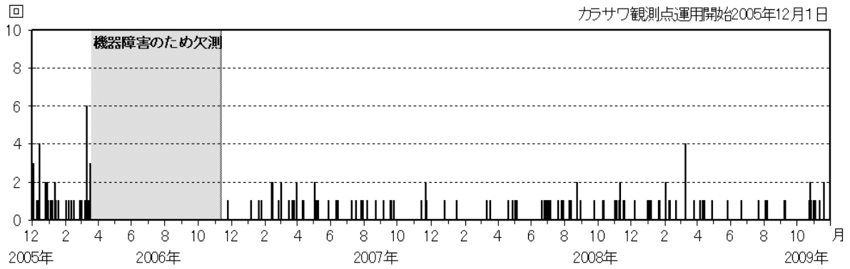
図2 新潟焼山 日別地震回数（2005年12月1日～2009年11月30日）
