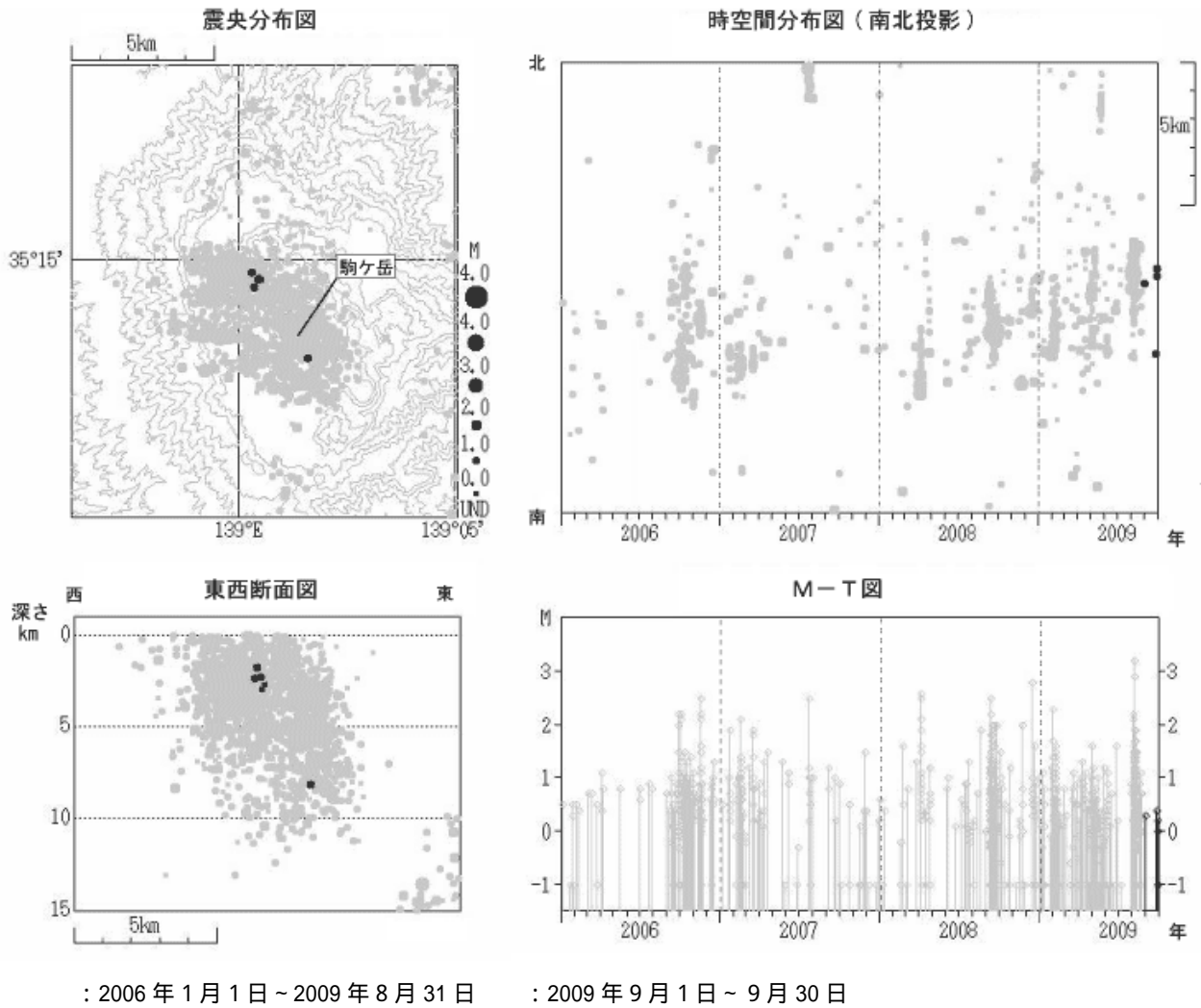
図3 箱根山 震源分布図（2006年1月1日～2009年9月30日） M（マグニチュード）は地震の規模を表します。 図中の震源要素は一部暫定値が含まれており、後日変更することがあります。
