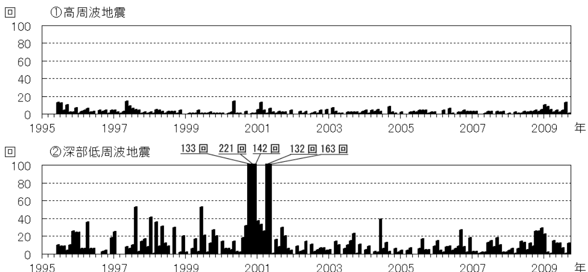
図 2 富士山 月別地震回数(1995 年 6 月～2009 年 9 月)
