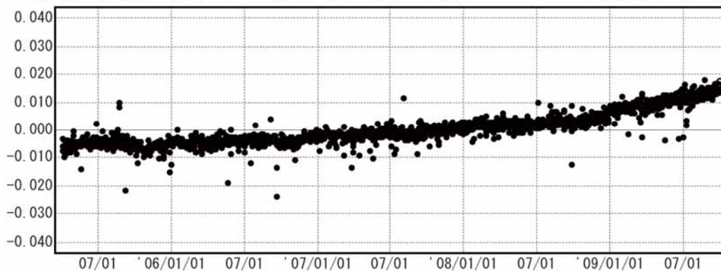
図3 富士山 国土地理院によるGPS観測結果 1) (2005年4月1日～2009年9月30日)
