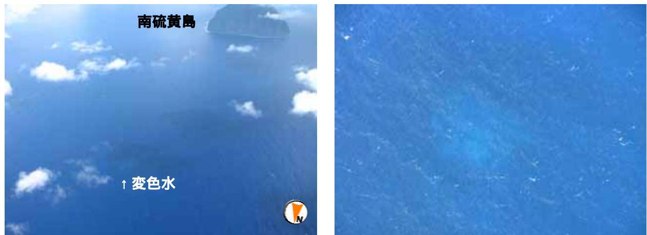
図 1 福德岡ノ場 変色水の状況（7 月 27 日、海上自衛隊の協力による）
