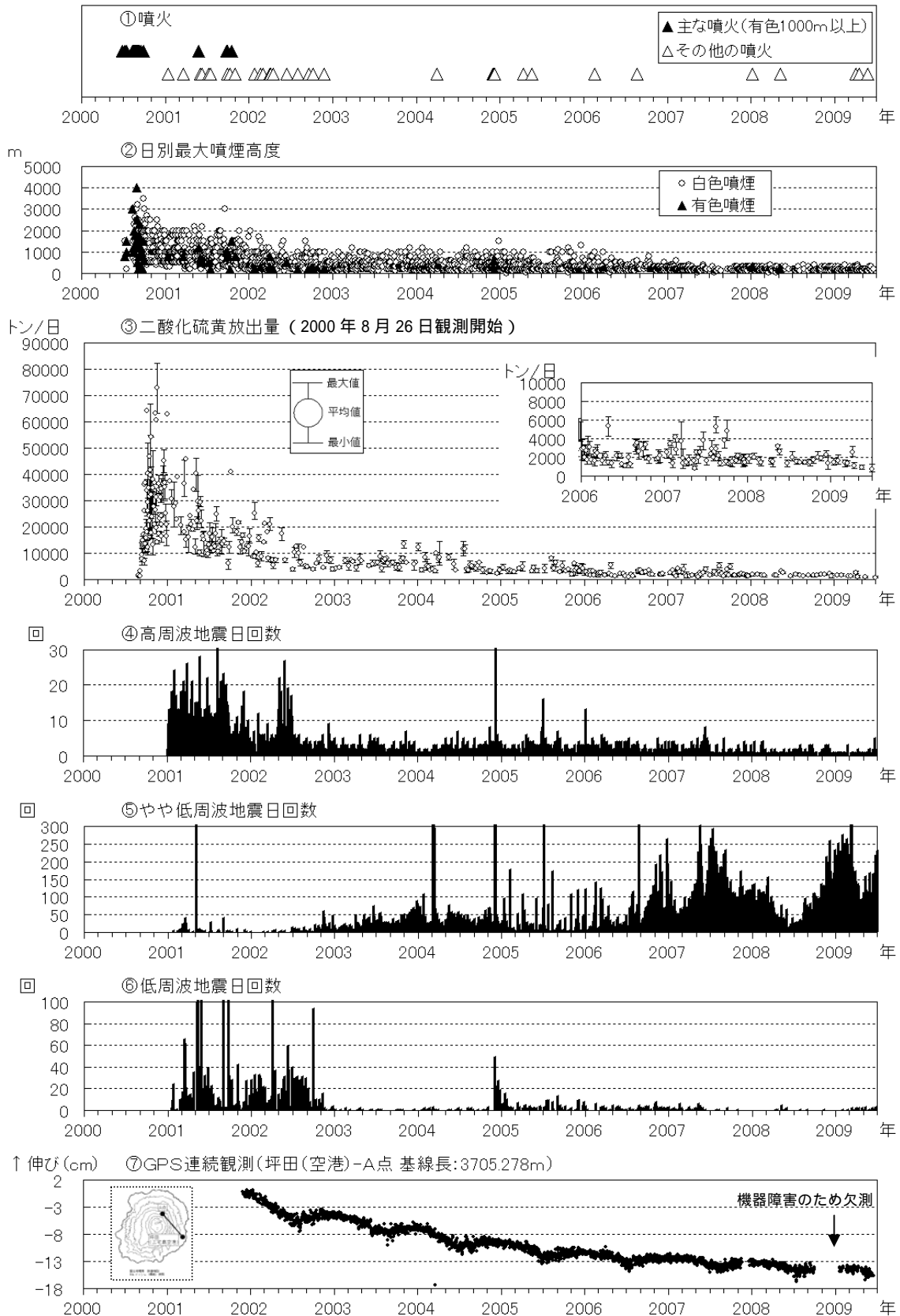
図2 三宅島 最近の火山活動の推移（2000年1月～2009年6月）
