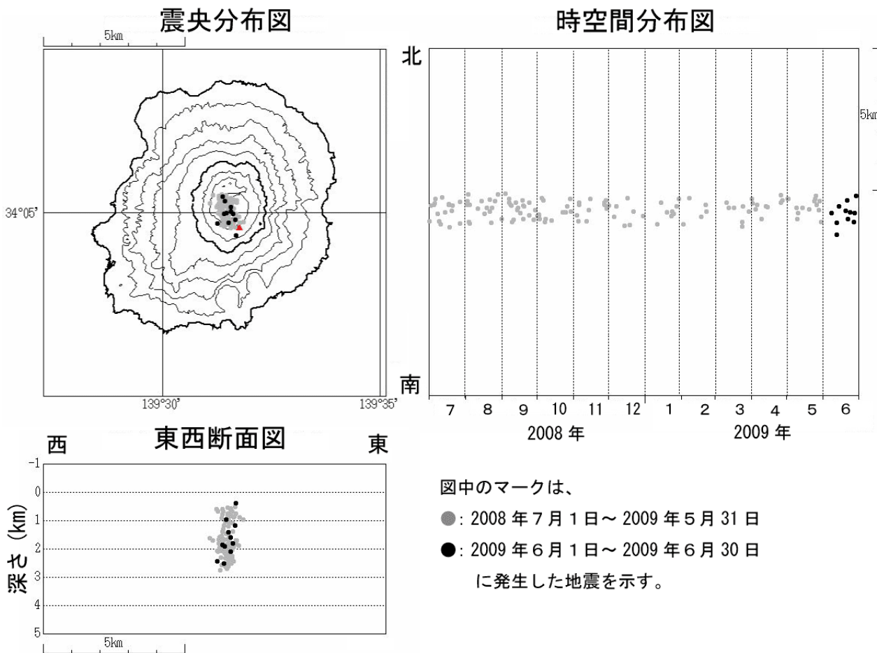
図4 三宅島 震源分布図（2008年7月1日～2009年6月30日）
