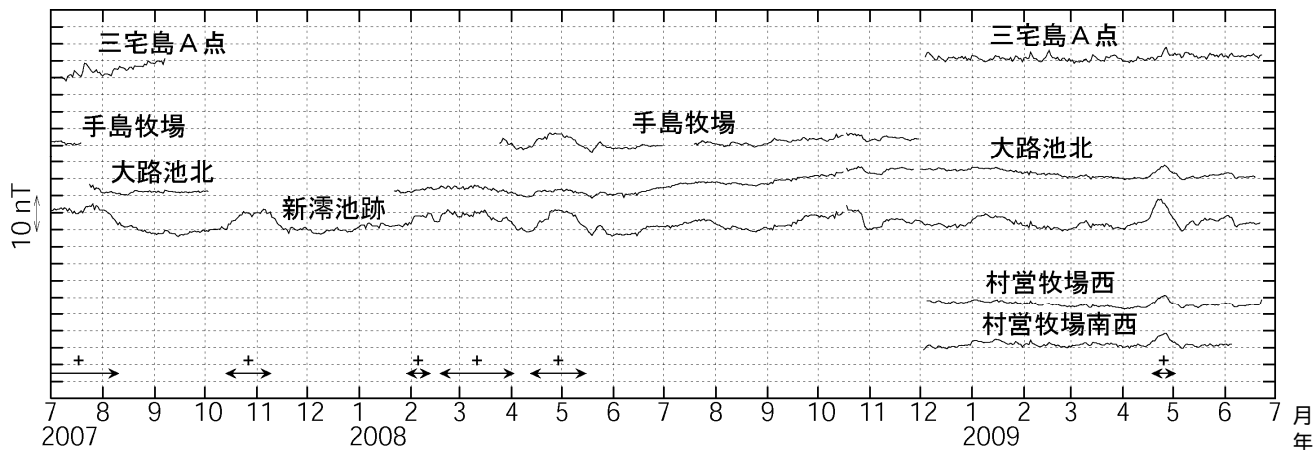
図3 三宅島 全磁力連続観測による全磁力値の変化（2007年7月～2009年6月22日） ←→で示した期間の全磁力値は三宅島周辺の海流の影響を受けていると推測されます。 nT（ナノテスラ）は磁場の強さを表す単位です。 2008年10月下旬の全磁力減少の原因は不明ですが、黒潮の流軸が離れていく場合に同様の傾向がみられます。
