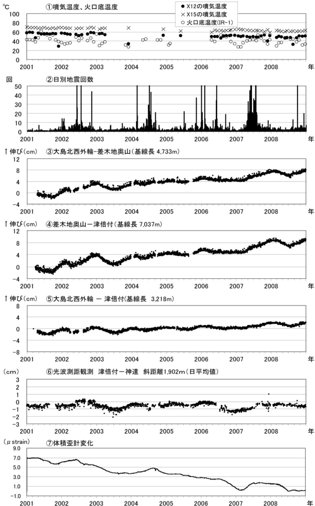
図5 伊豆大島 最近の火山活動経過図(2001年1月~2008年12月)
