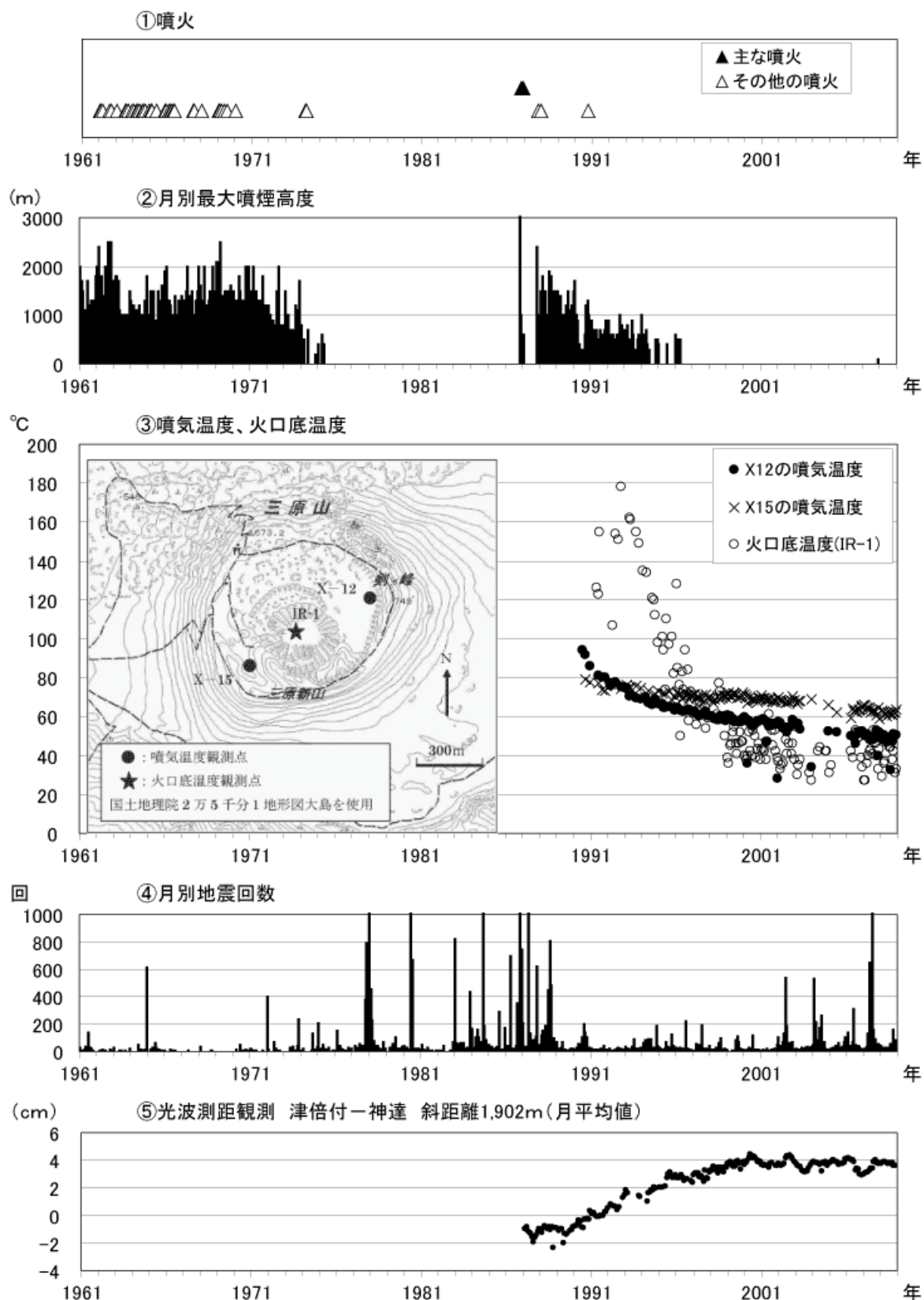
図4 伊豆大島 長期間の火山活動経過図(1961年1月~2008年12月) 1991年12月18日までは火口縁上130m以上、2002年2月28日までは火口縁上300m以上の噴煙高度を観測していました。 火口底温度(IR-1)は赤外放射温度計 1) を用いて離れた場所(図3赤外熱映像観測点と同じ)から測定した値。噴気温度(X-12、X-15)はサーミスタ温度計を用いて直接測定した値。 地震回数には伊豆大島周辺海域で発生した地震も一部含まれています。 光波距離計 2) による月平均値(観測開始は1987年1月)。
