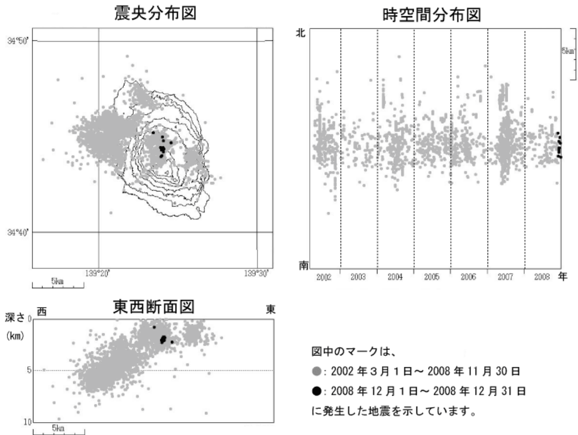
図6 伊豆大島 震源分布図(2002年3月1日～2008年12月31日)
