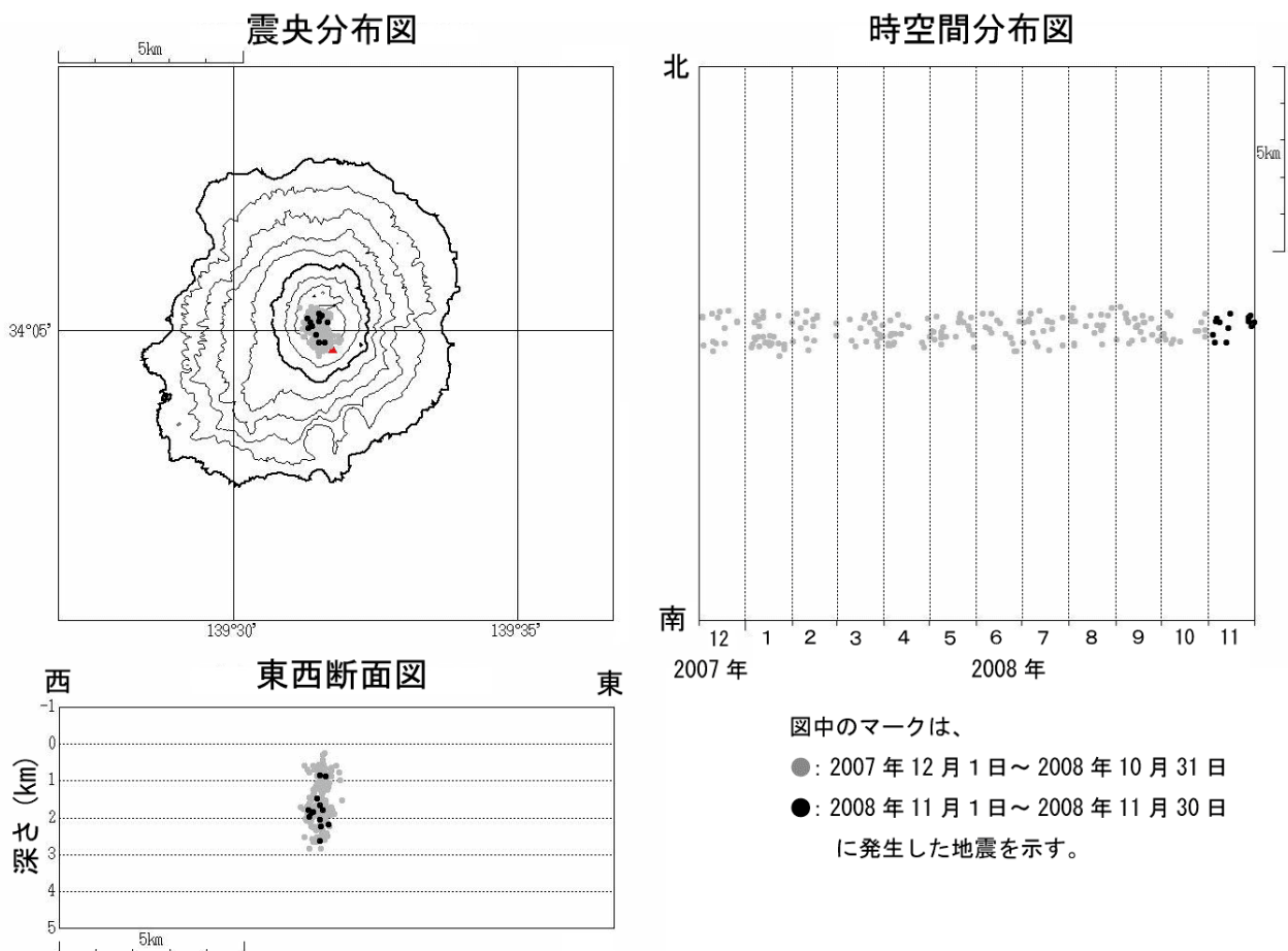
図 4 ※ 三宅島 震源分布図 (2007 年 12 月 1 日～2008 年 11 月 30 日)
