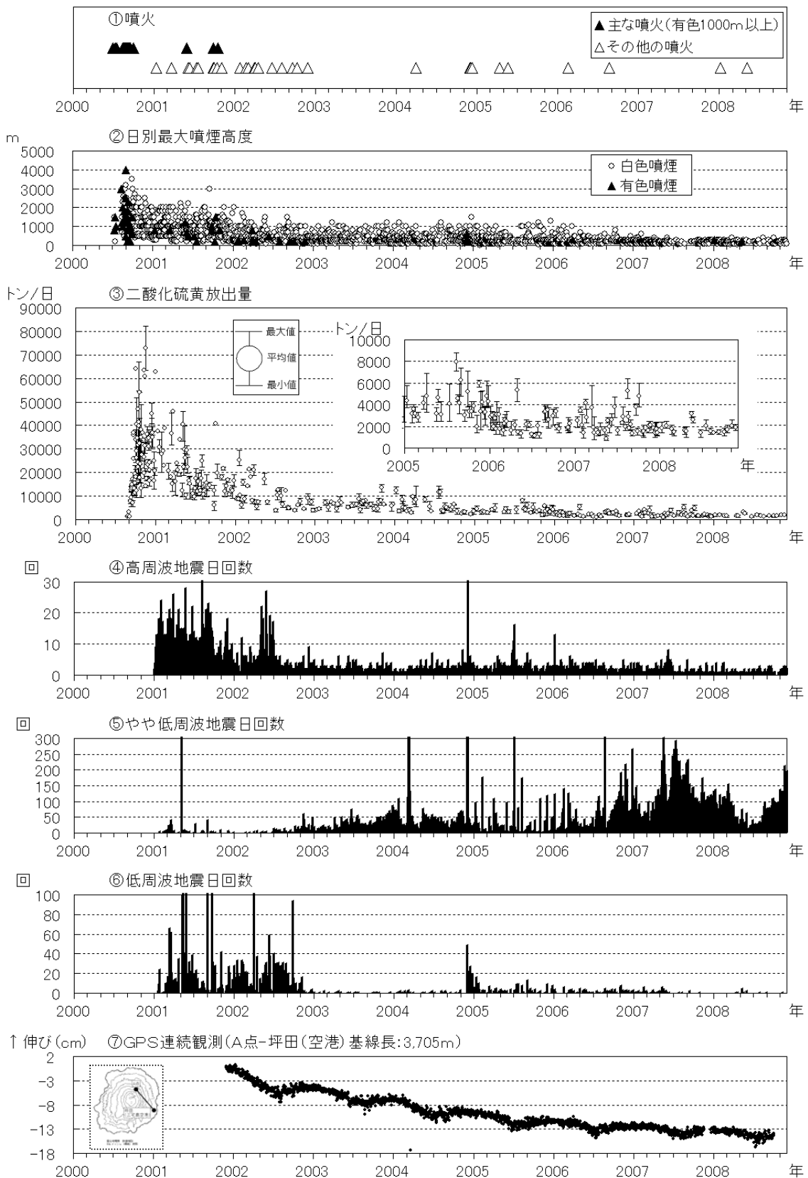
図2 三宅島 最近の火山活動の推移 (2000年1月～2008年11月)
