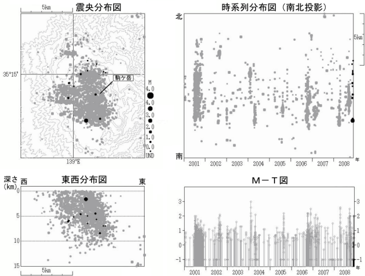
図 3※ 箱根山 震源分布図（2001 年 1 月 1 日～2008 年 11 月 30 日）
