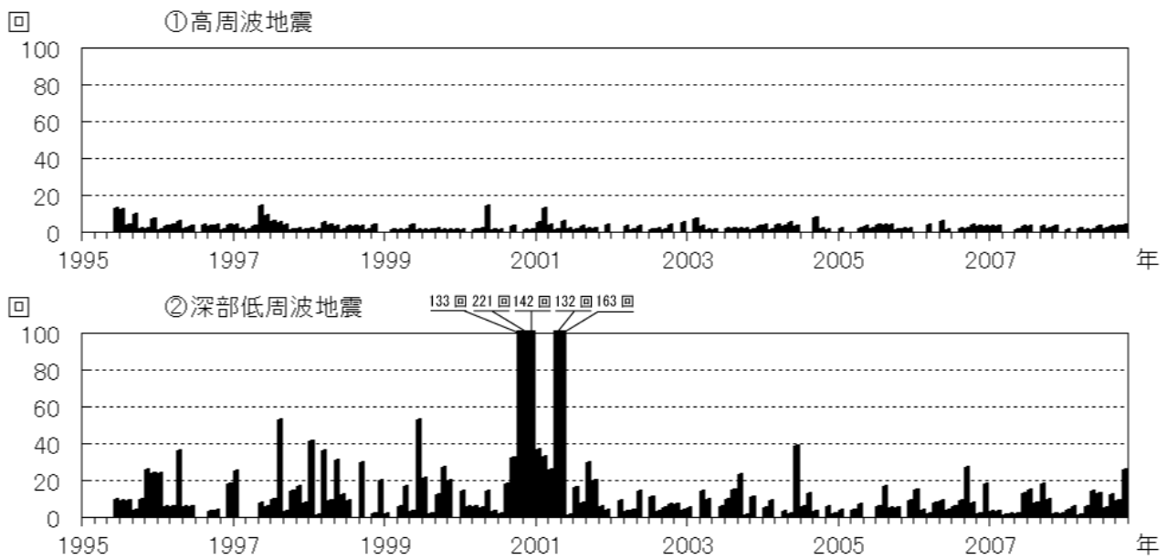
図1 富士山 月別地震回数(1995年6月～2008年10月)
