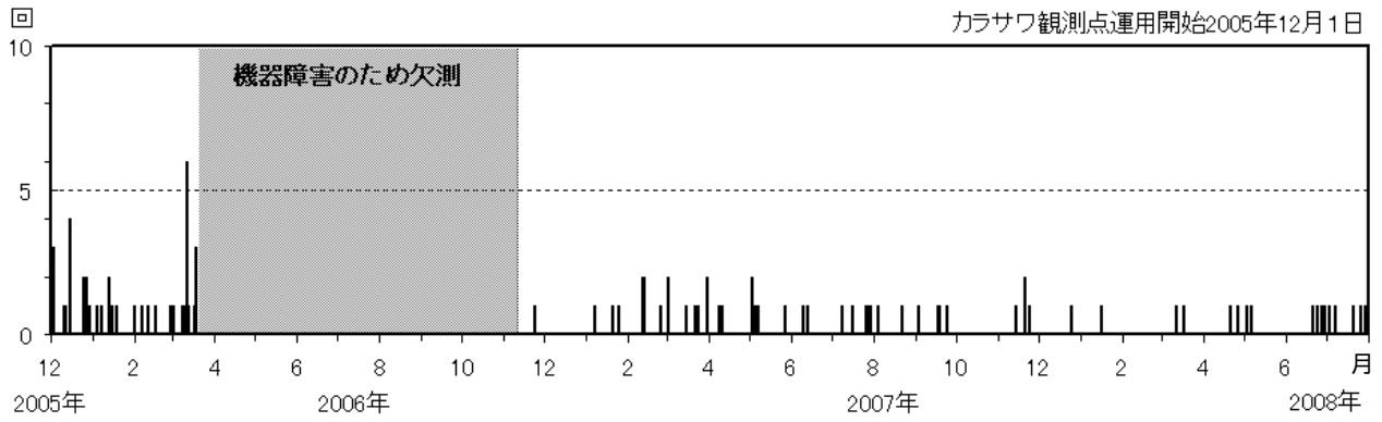
図 2 新潟焼山 日別地震回数（2005 年 12 月 1 日～2008 年 7 月 31 日）
