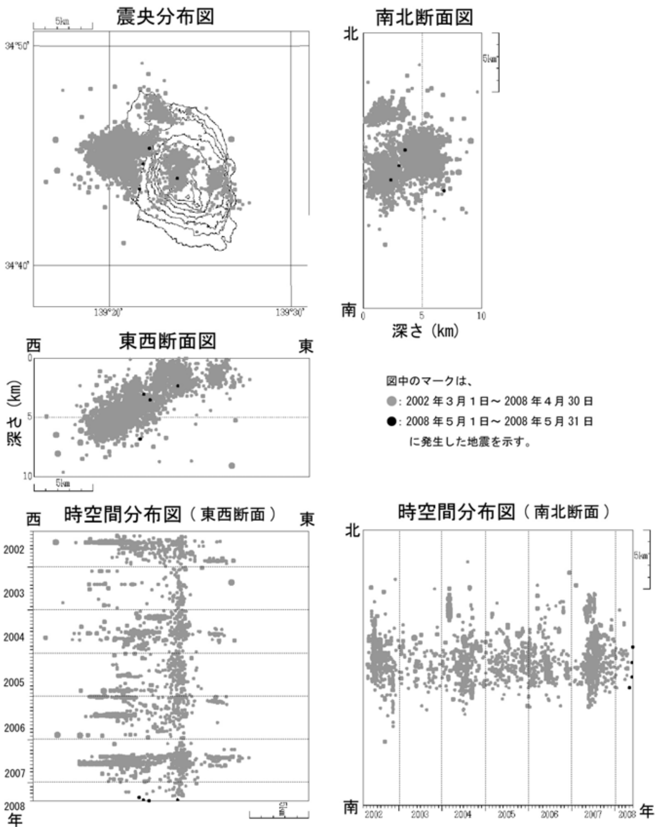
図6 伊豆大島 震源分布図(2002年3月1日～2008年5月31日)
