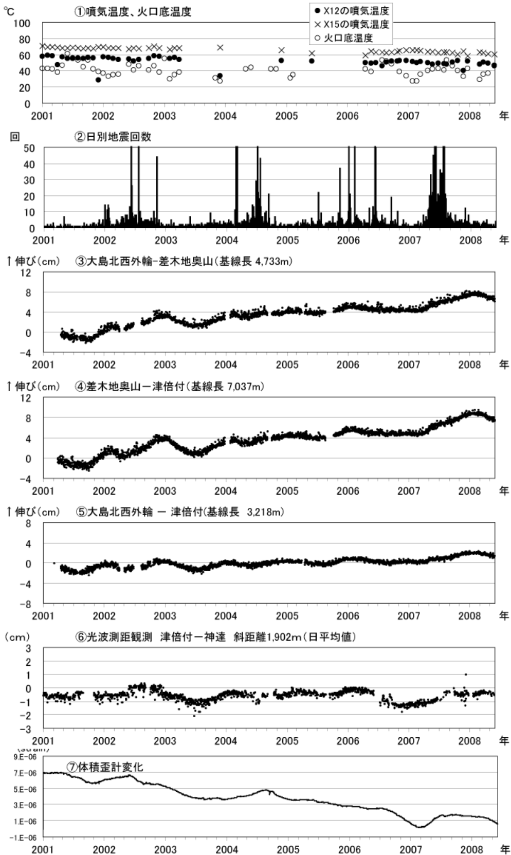
図5 伊豆大島 最近の火山活動経過図(2001年1月~2008年5月)
