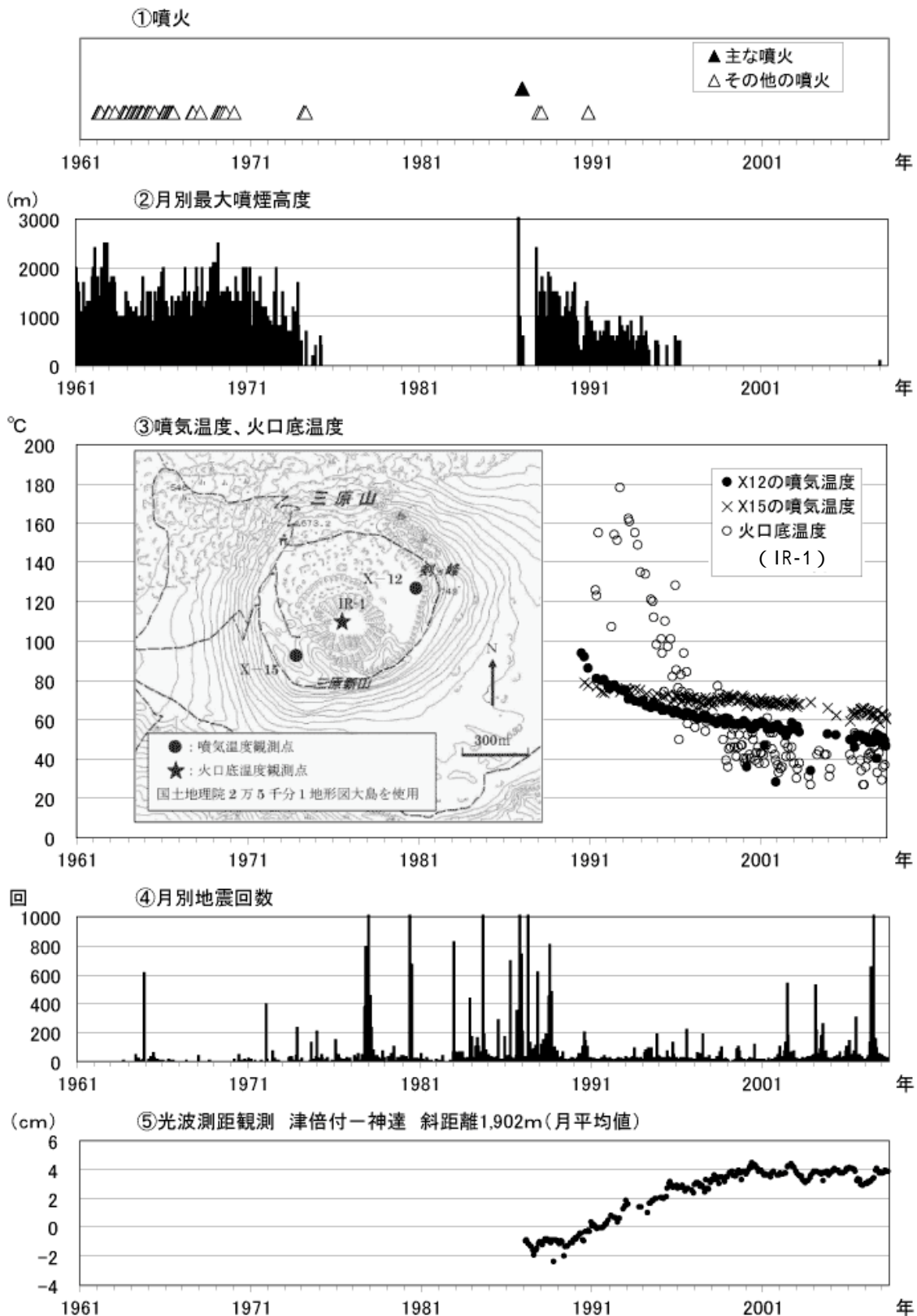
図4 伊豆大島 長期間の火山活動経過図（1961年1月～2008年5月）
