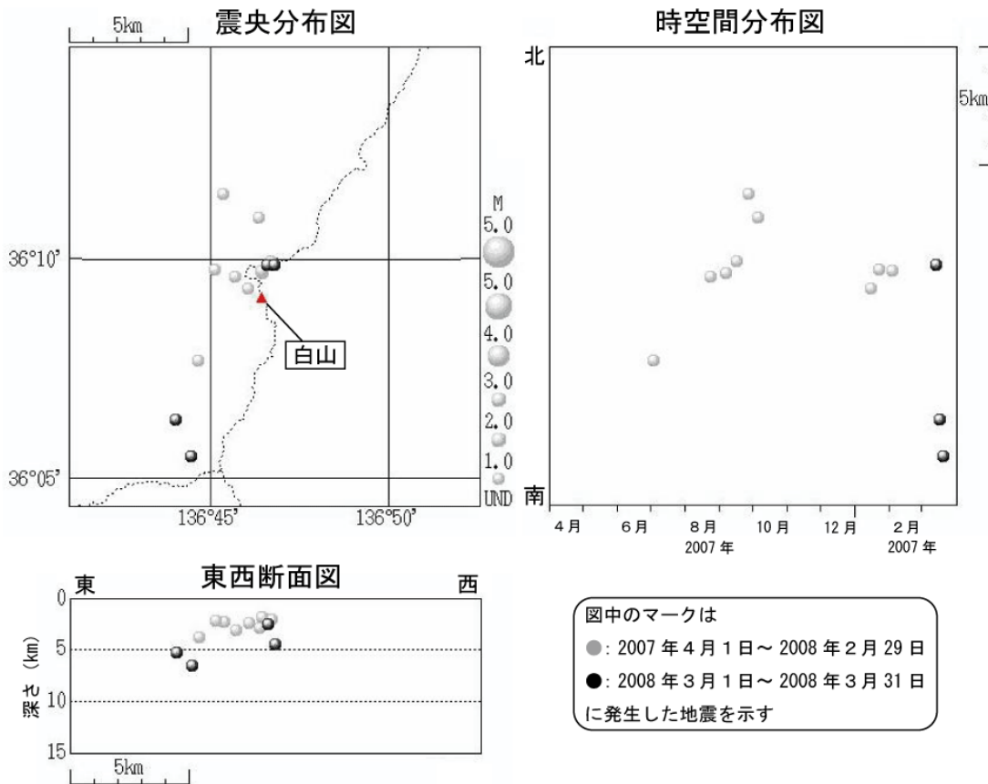
図 1 白山 山体周辺及びその周辺の地震活動（2007 年 4 月 1 日～2008 年 3 月 31 日） M（マグニチュード）は地震の規模を表します。資料中の M は一部暫定値が含まれており、後日変更することがあります。
