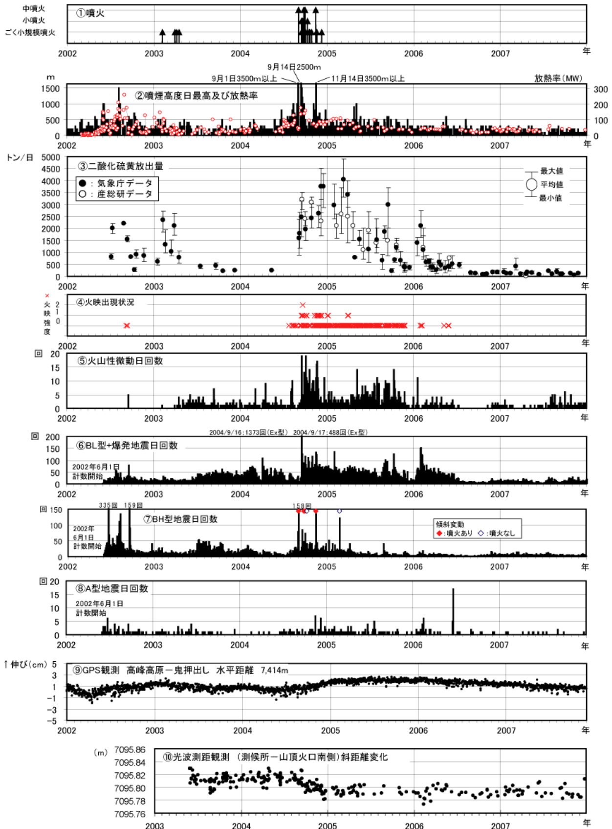
図 2※ 浅間山 最近の火山活動の推移（2002 年 1 月～2007 年 12 月）
