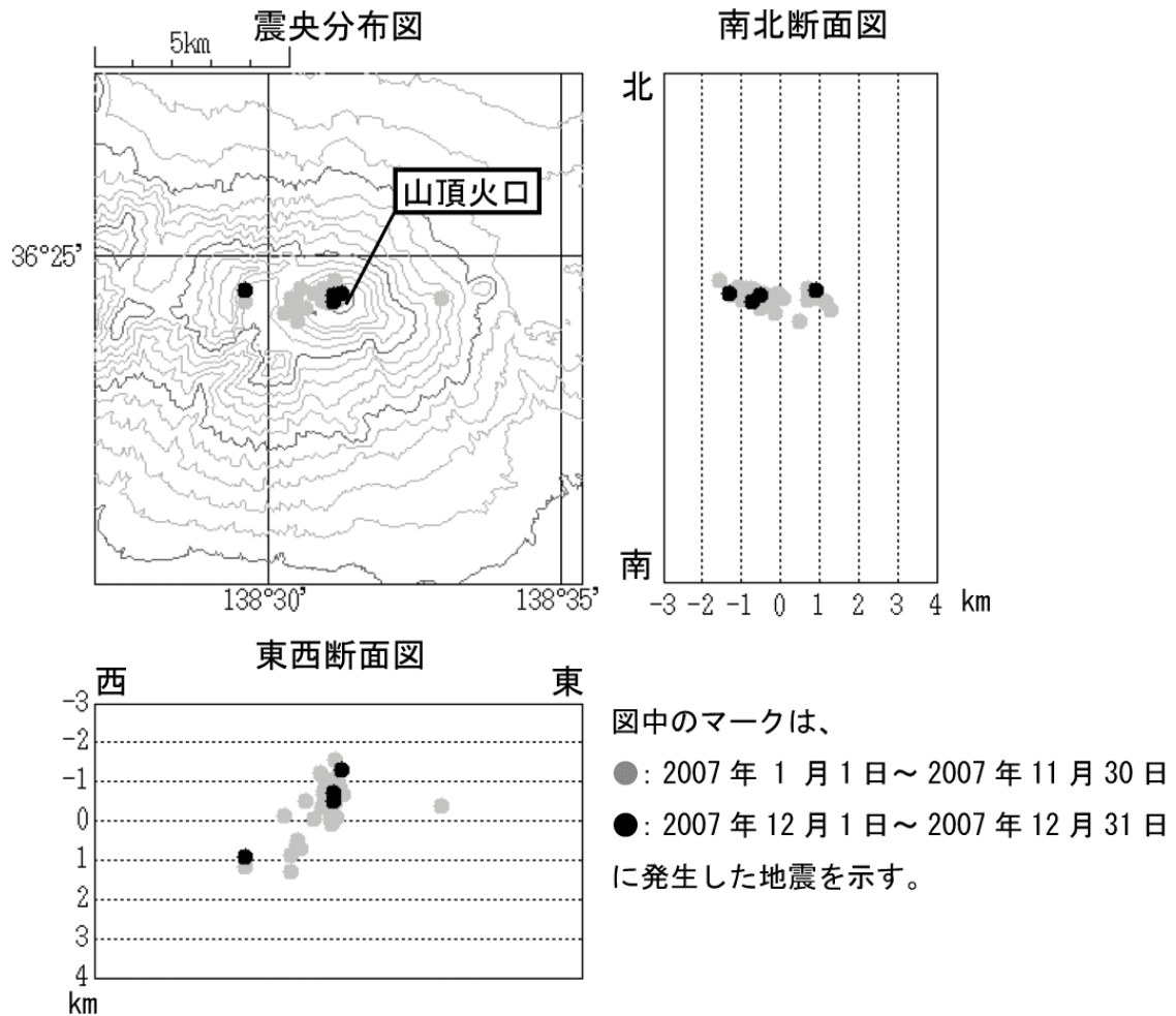
図 3※ 浅間山 火山性地震の震源分布（2007 年 1 月 1 日～2007 年 12 月 31 日）
