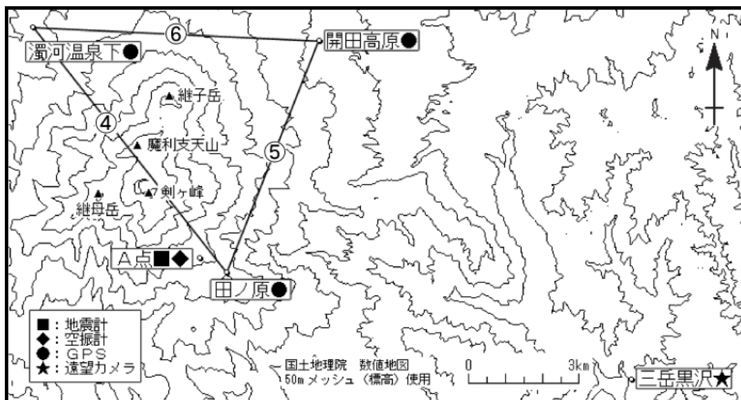
図 5 御嶽山 気象庁の観測点配置図（小さな白丸は観測点位置を示しています） 図中の GPS 基線 ～ は図 3 の ～ に対応しています。
