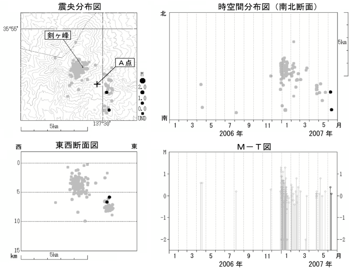
図 4 御嶽山 山頂付近の地震活動（2006 年 1 月 1 日～2007 年 6 月 30 日） ●：2007 年 6 月 1 日～2007 年 6 月 30 日 ●：2006 年 1 月 1 日～2007 年 5 月 31 日 M（マグニチュード）は地震の規模を表します。資料中の M は一部暫定値が含まれており、 後日変更することがあります。+ 印は気象庁地震観測点（A 点）の位置を示しています。
