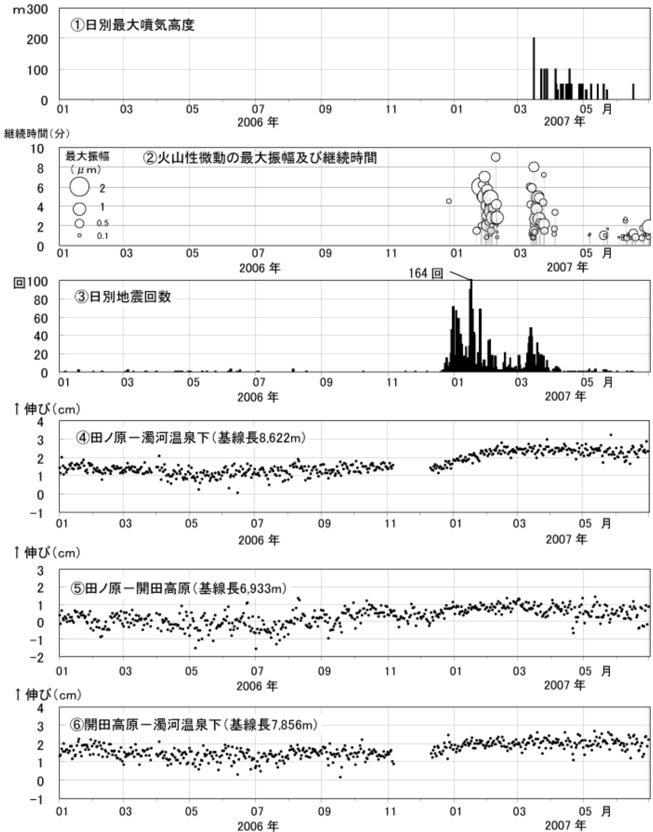
図3 御嶽山 最近の火山活動の推移（2006年1月1日～2007年6月30日） 図中 ～ は図5のGPS基線 ～ に対応しています。
