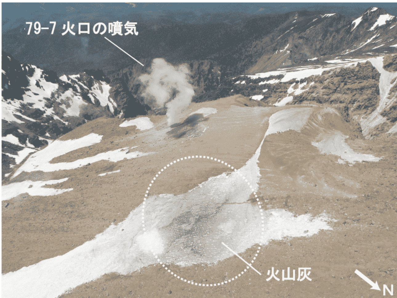
図 2 御嶽山 79-7 火口の噴気の状況（6 月 7 日 長野県の協力による）
