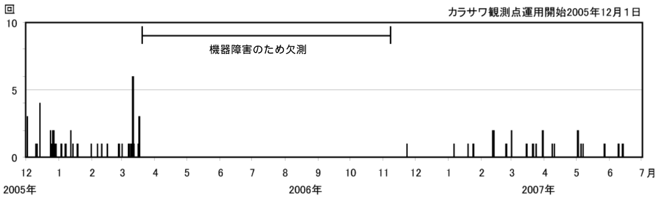
図2 新潟焼山 日別地震回数(2005年12月1日~2007年6月30日)
