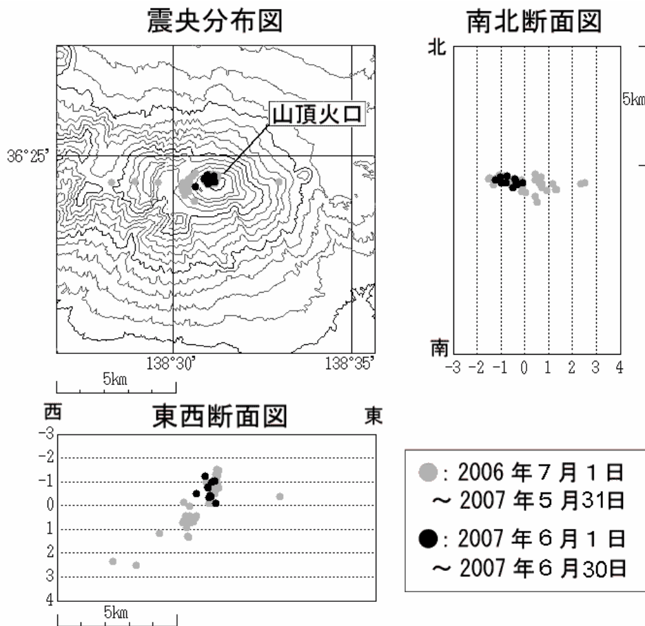
図3 浅間山 火山性地震の震源分布（2006年7月1日～2007年6月30日）
