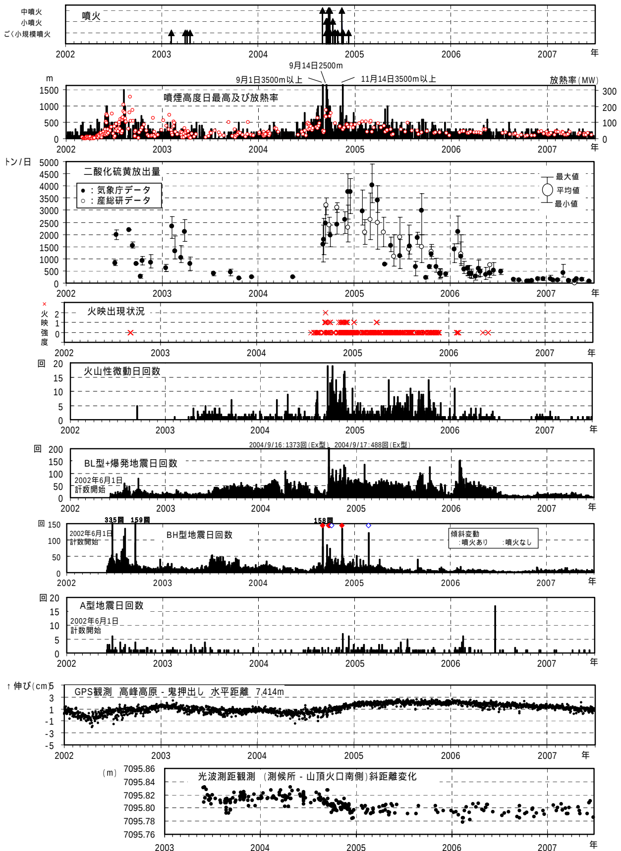
図2 浅間山 最近の火山活動の推移（2002年1月～2007年6月） 産業技術総合研究所による観測データ（産総研データ）が含まれています 地震の種類別（図5参照）に計数を開始した2002年6月1日からのデータを掲載。
