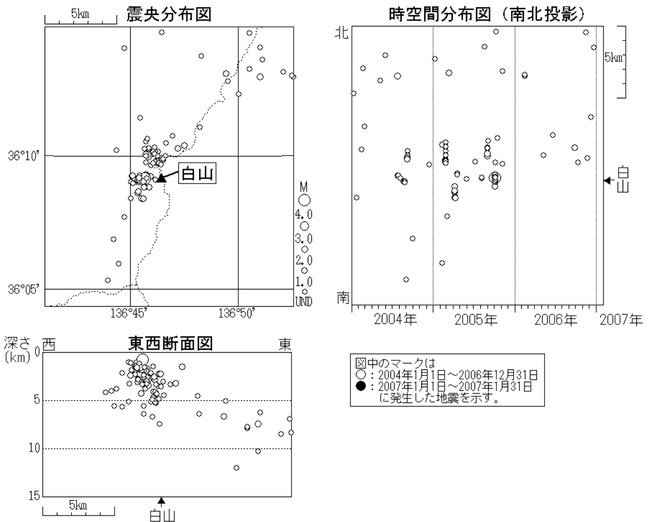
図 3※ 白山 山体及びその周辺の地震活動（2004 年 1 月 1 日～2007 年 1 月 31 日）
