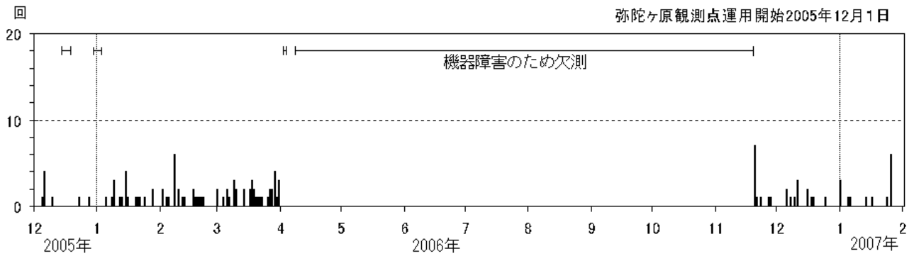
図 2 白山 日別地震回数（2005 年 12 月 1 日～2006 年 12 月 31 日）
