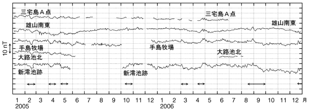
図 4 三宅島 全磁力連続観測による全磁力値の変化（2004 年 12 月 1 日～2006 年 12 月 31 日） ↔で示した期間の全磁力値は三宅島周辺の海流の影響を受けていると推測されます。 nT（ナノテスラ）は磁場の強さを表す単位です。
