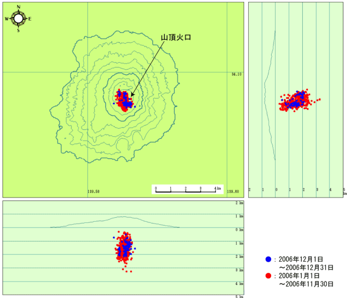
図 3※ 三宅島 火山性地震の震源分布（2006 年 1 月 1 日～2006 年 12 月 31 日）
