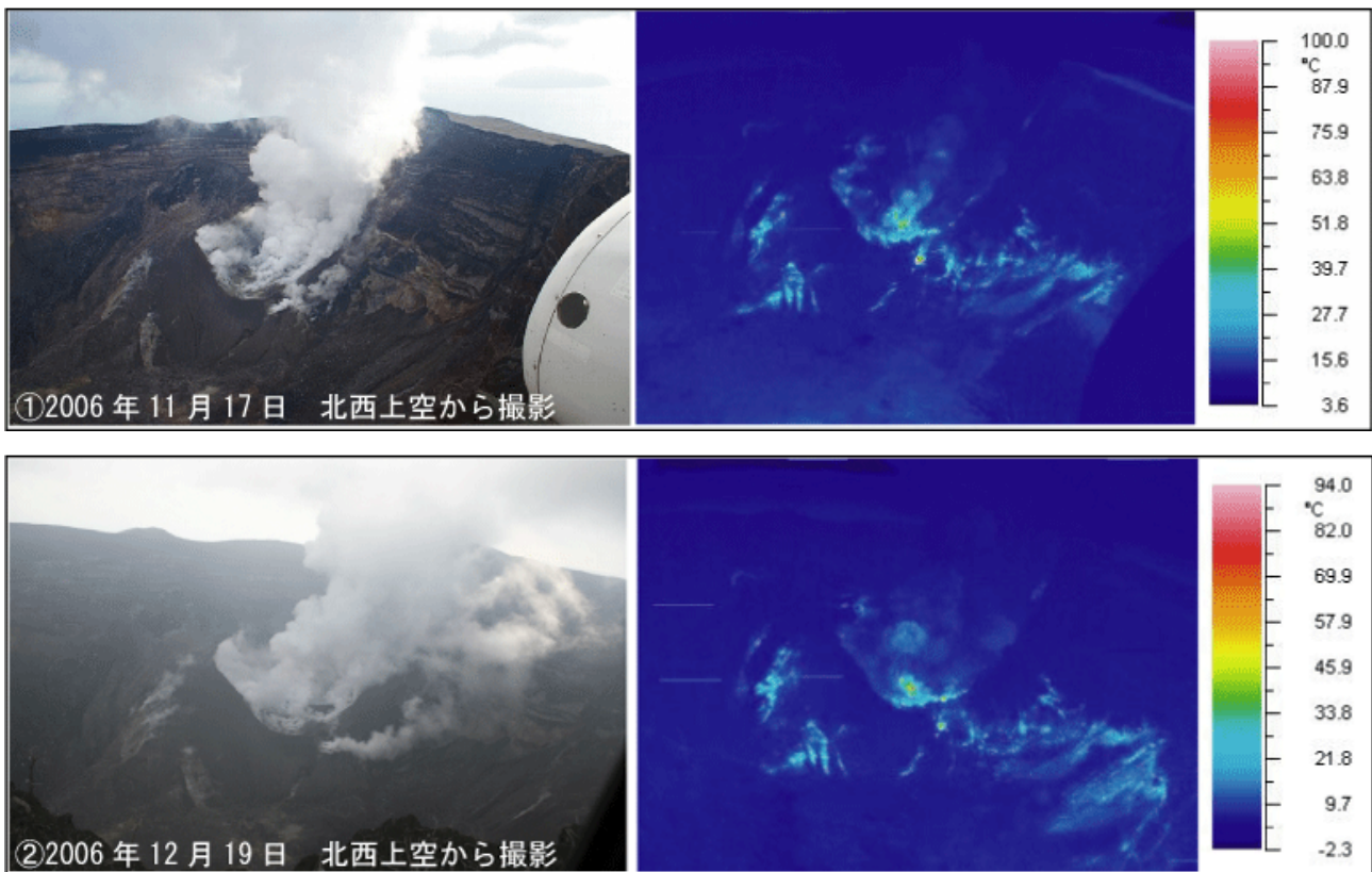
図1 三宅島 山頂火口の噴煙の状況及び赤外熱映像装置で捉えた火口内の温度分布 ①の画像右側には機体が重なり地表面温度分布が描画されていない部分があります。
