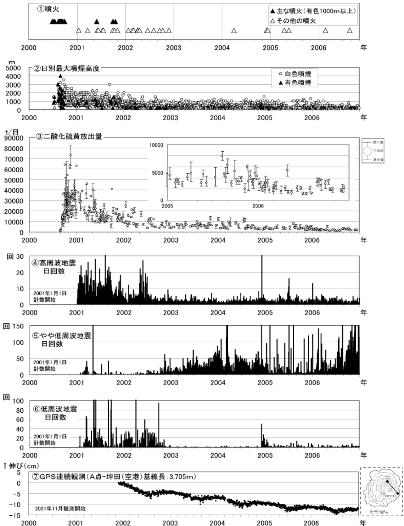
図2 三宅島 最近の火山活動の推移（2000年1月～2006年12月）
