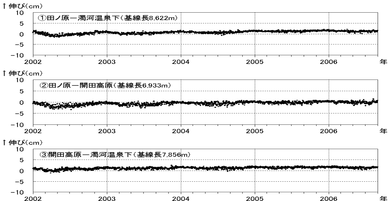
図 2 御嶽山 G P S 連続観測による基線長変化（2002 年 1 月 1 日～2006 年 8 月 31 日）
