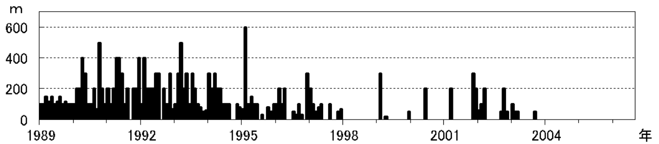
図 3 御嶽山 定時観測（09時・16時）による月別最大噴煙高度（1989年 1 月～2006年 8 月）
