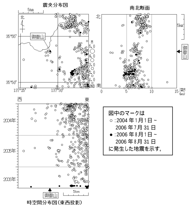
図 1 御嶽山 山体及びその周辺の地震活動 （2004 年 1 月 1 日～2006 年 8 月 31 日）
