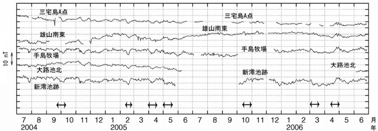
図4 三宅島 全磁力連続観測による全磁力値の変化 (2004年 7 月 1 日～2006年 6 月 30 日)
