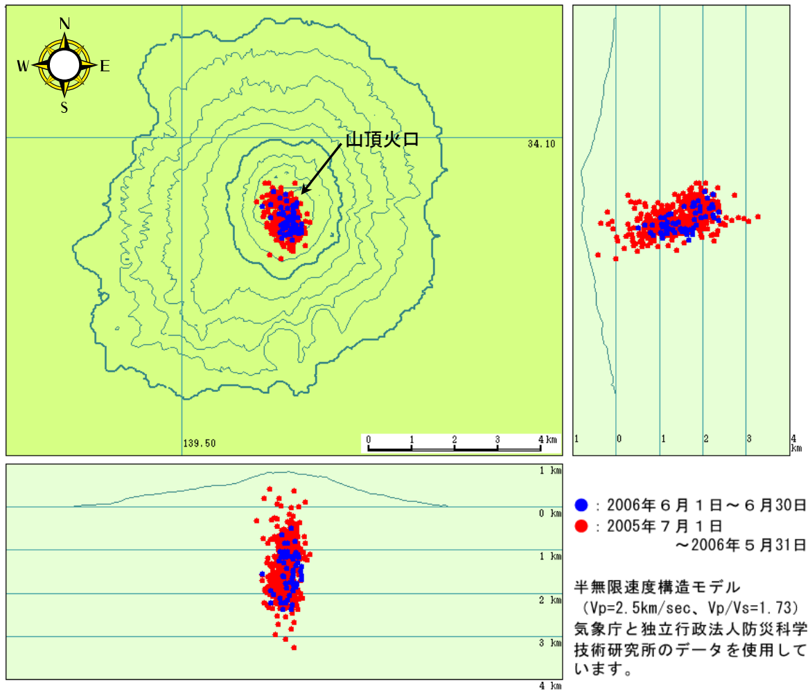
図3 三宅島 火山性地震の震源分布図 (2005年 7 月 1 日～2006年 6 月 30 日)
