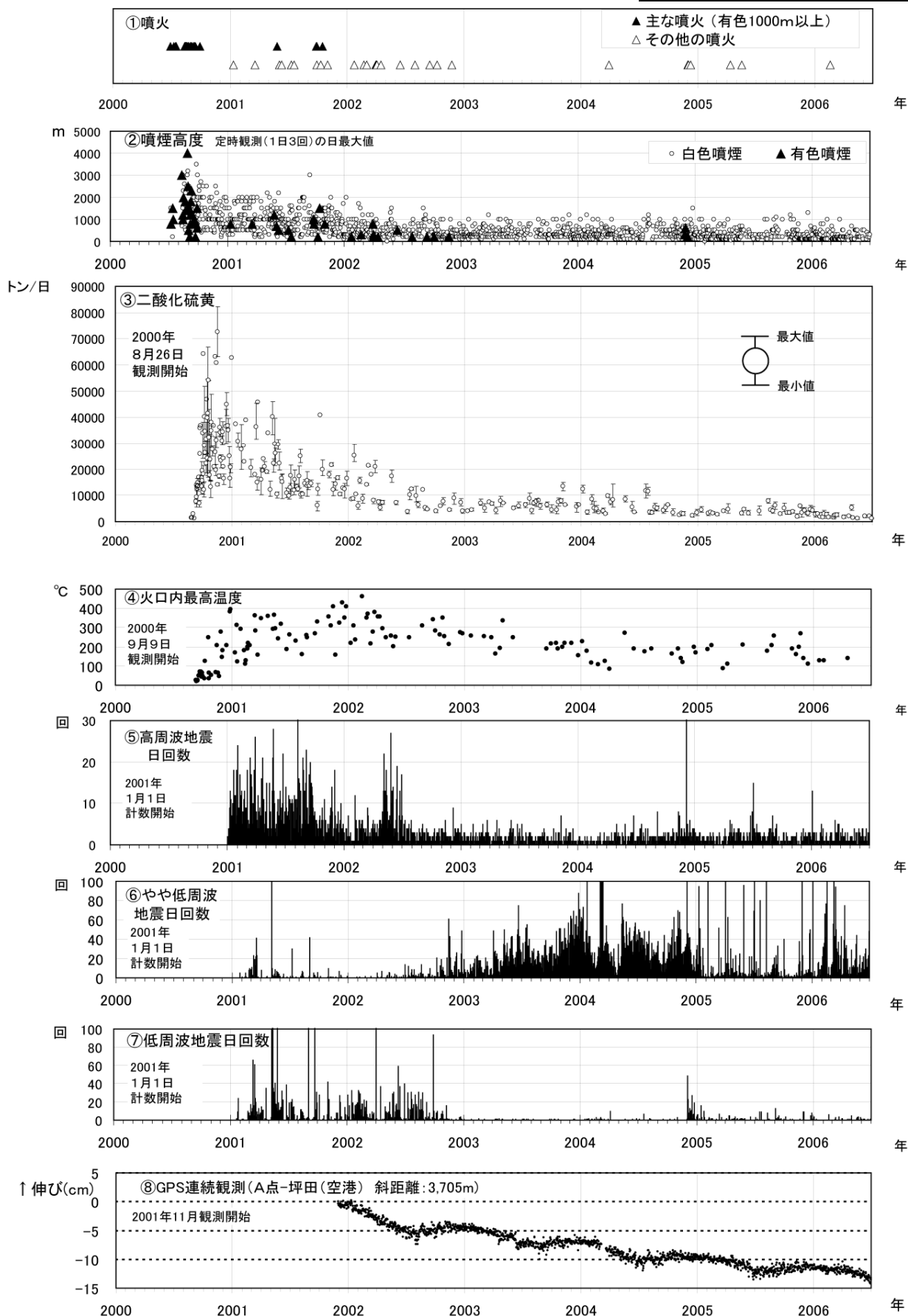
図 2 三宅島 最近の火山活動の推移 (2000年 1月～2006年 6月)
