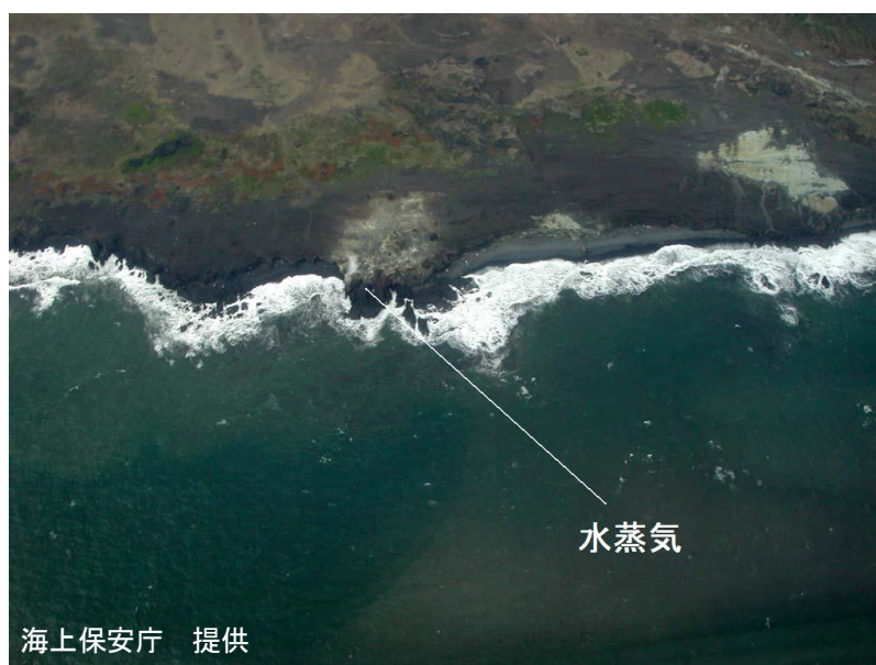
図 2 硫黄島 離岸温泉跡付近水蒸気（近景）（3 月 15 日、島の北東上空から撮影）
