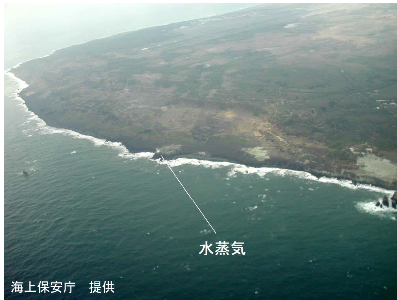
図 1 硫黄島 離岸温泉跡付近水蒸気（遠景）（3 月 15 日、島の北東上空から撮影）
