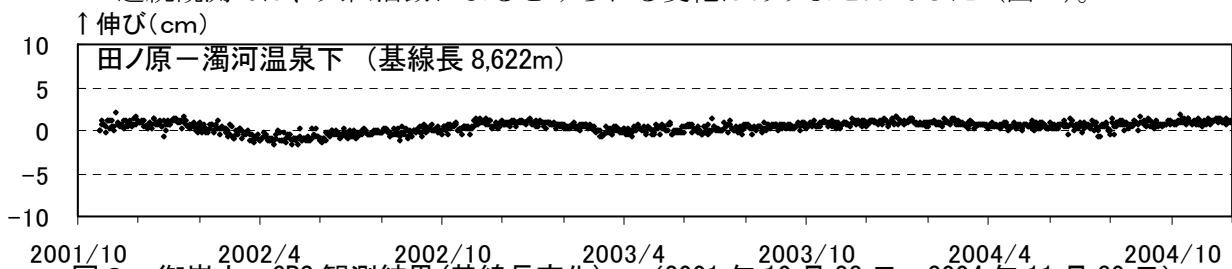
図 2 御嶽山 GPS 観測結果(基線長変化)（2001 年 10 月 23 日～2004 年 11 月 30 日）
