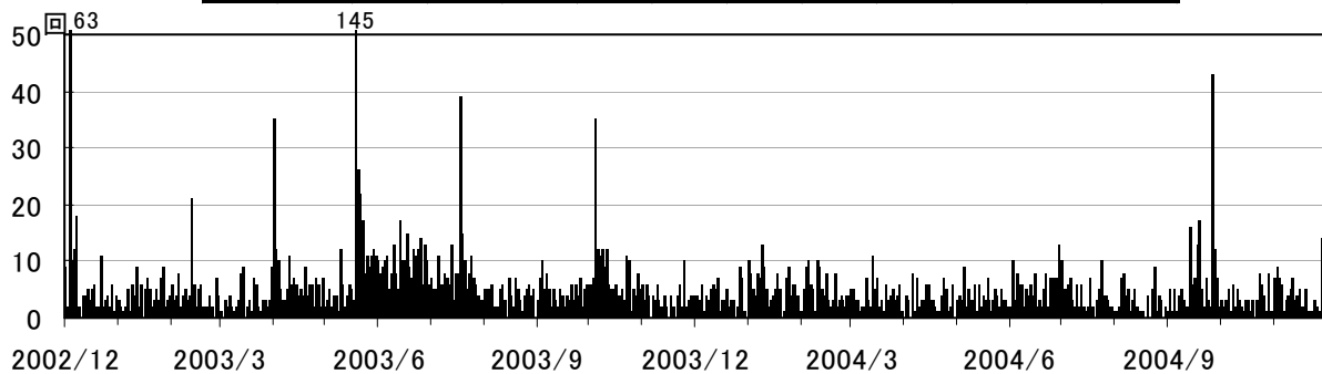
図 1 御嶽山 火山性地震日別回数（2002 年 12 月 1 日～2004 年 11 月 30 日）
