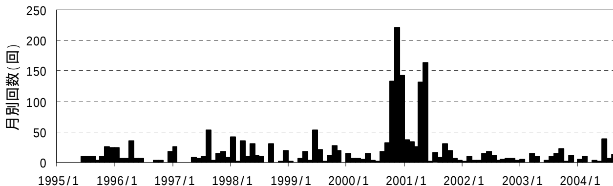
図2 富士山 低周波地震月別回数(1995年6月～2004年8月)
