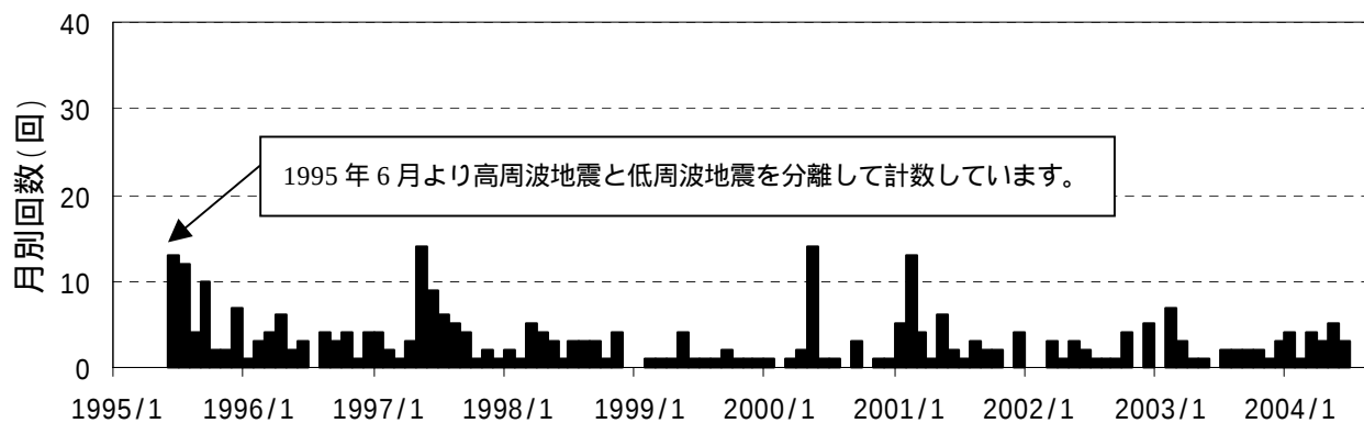
図1 富士山 高周波地震月別回数(1995年6月～2004年8月)
