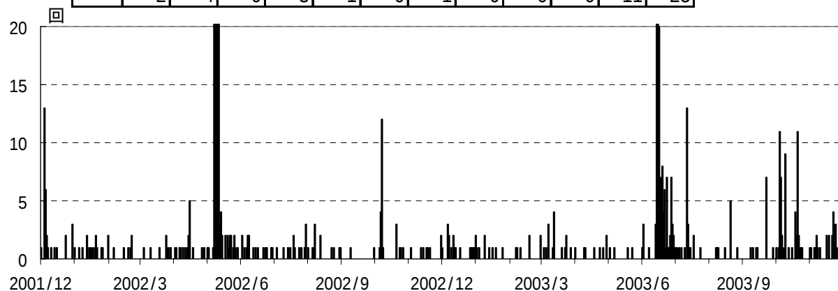
図 1 伊豆東部火山群 火山性地震日別回数(2001 年 12 月 1 日～2003 年 11 月 30 日)
