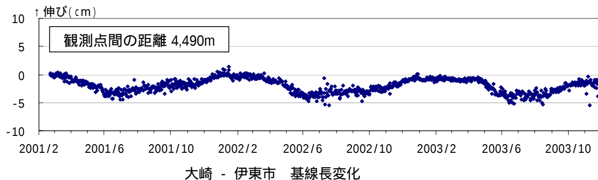
図 2 伊豆東部火山群 GPS 観測結果(2001 年 2 月 1 日～2003 年 11 月 30 日)
