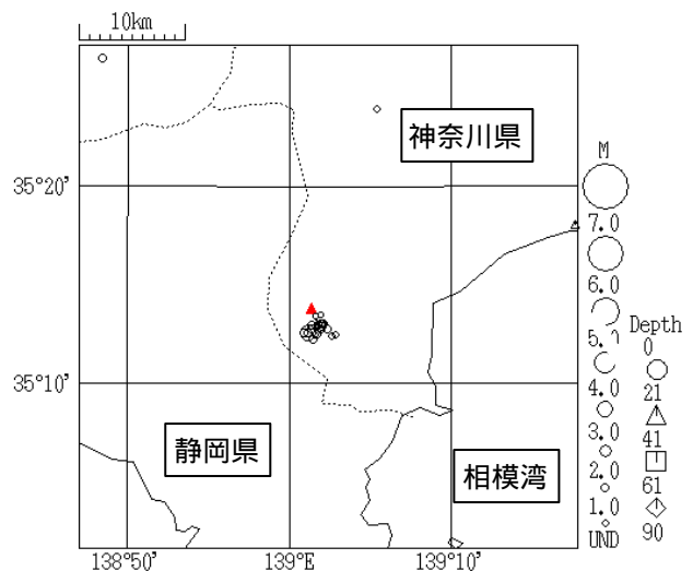
図4 箱根山周辺震央分布図(12/31~1/2)
