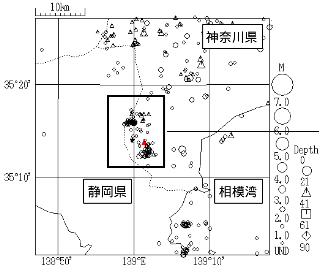
図1 2002年箱根山周辺震央分布図(1/1~12/31)
