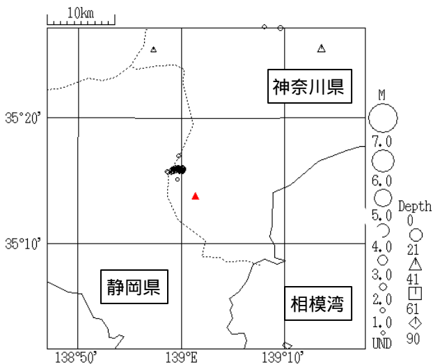
図3 箱根山周辺震央分布図(8/25~8/31)
