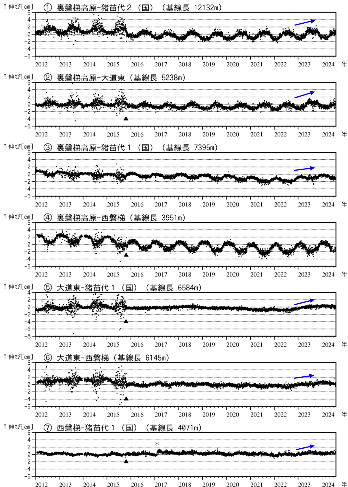
図7 磐梯山 GNSS 基線長変化図 (2012年1月～2024年7月)
