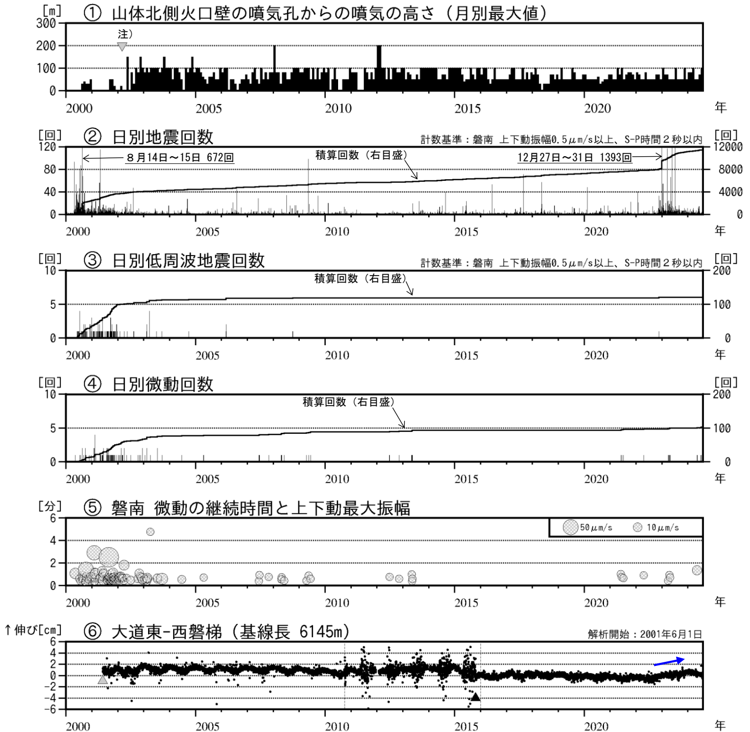
図3 磐梯山 火山活動経過図（2000年1月～2024年7月）
