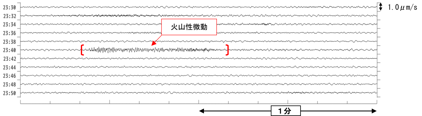
図4 磐梯山 裏磐梯高原観測点（上下成分）での火山性微動の発生状況 （2024年7月3日23時30分～23時52分）
