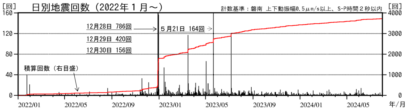
図5 磐梯山 地震回数（2022年1月～2024年7月）
