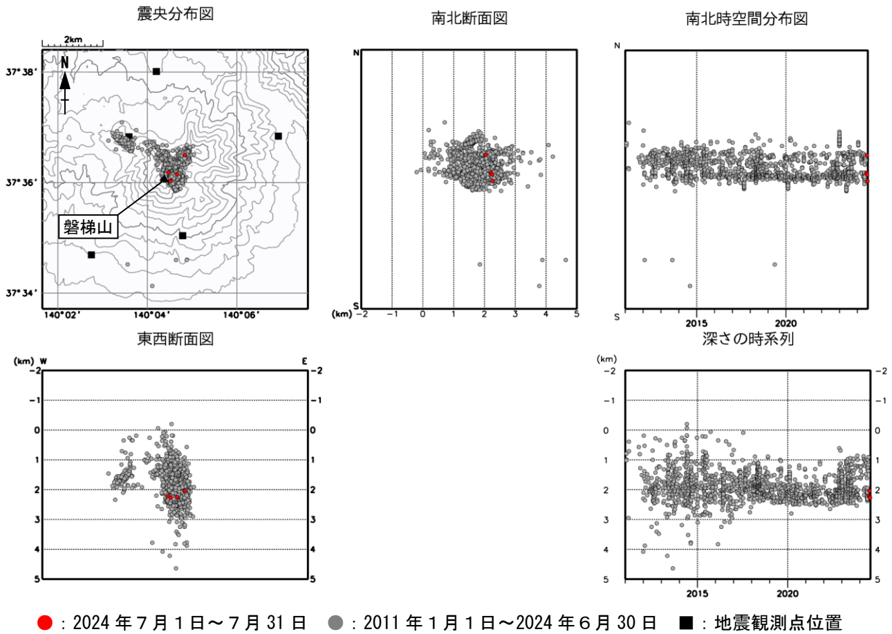
図6 磐梯山 震源分布図（2011年1月～2024年7月）
