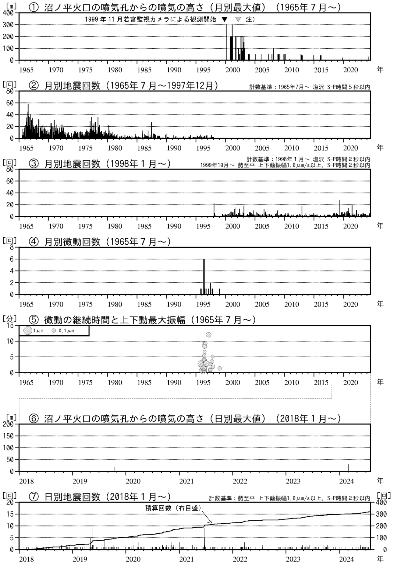
図 3 安達太良山 火山活動経過図（1965 年 7 月～2024 年 7 月）
