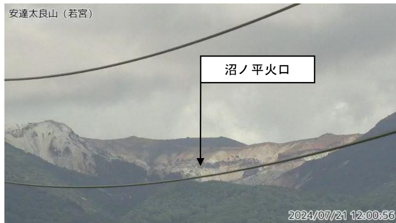
図1 安達太良山 沼ノ平火口周辺の状況（7月21日）
