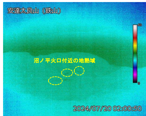
図2 安達太良山 沼ノ平火口周辺の状況（7月21日）と地表面温度分布の状況（7月20日）
