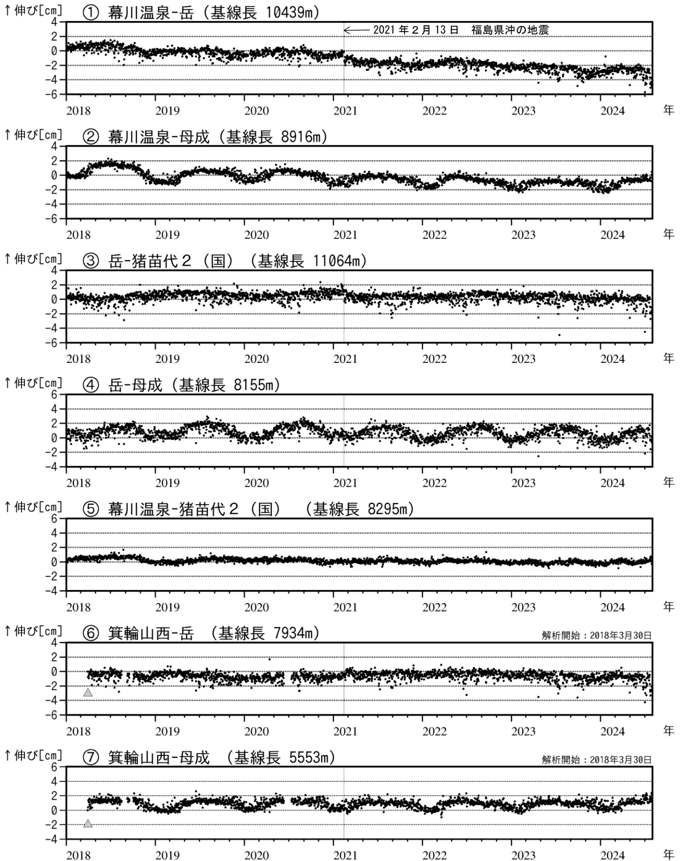
図4 安達太良山 GNSS 基線長変化図（2018年1月～2024年7月）
