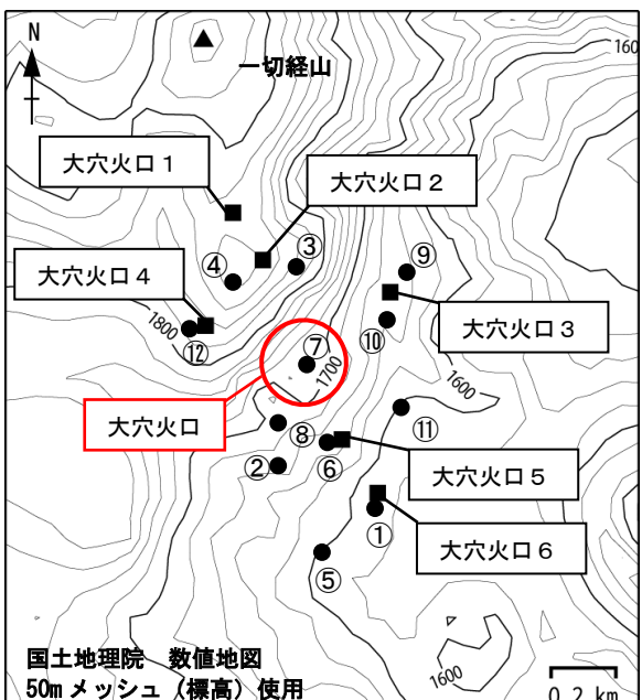
図14 吾妻山 全磁力観測点配置図
