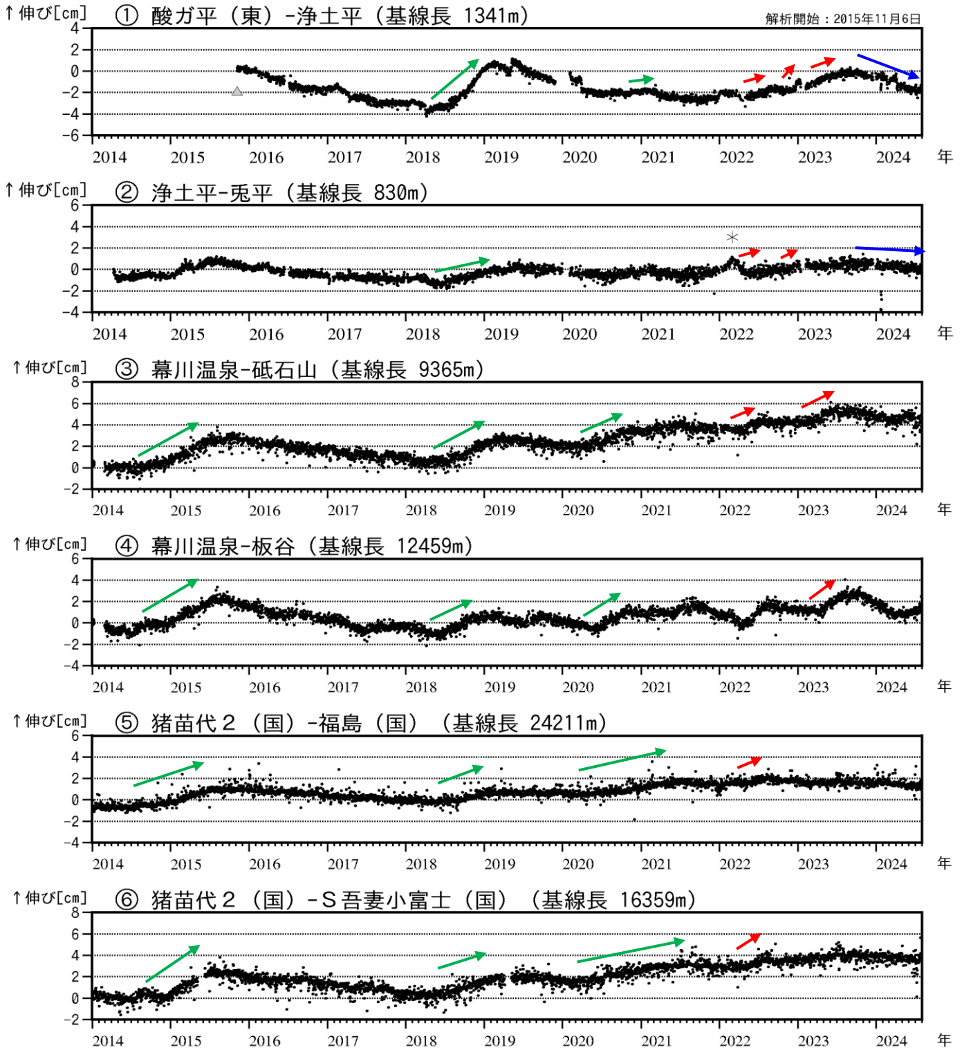
図4 吾妻山 吾妻山浅部・深部の地殻変動(2014年1月~2024年7月)
