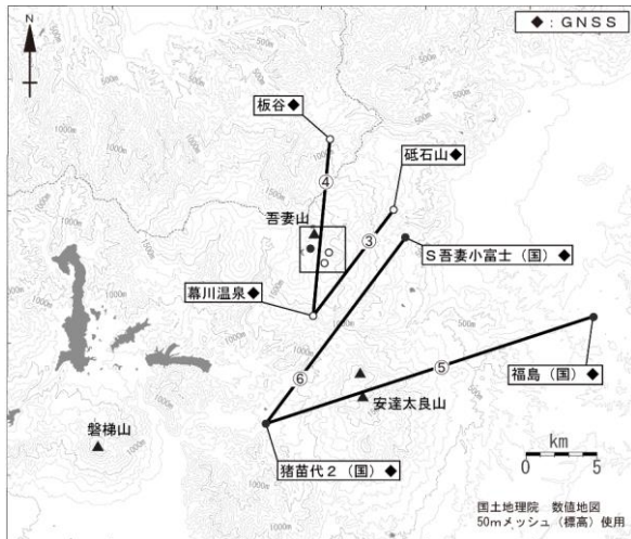
図13 吾妻山 GNSS 観測基線図
