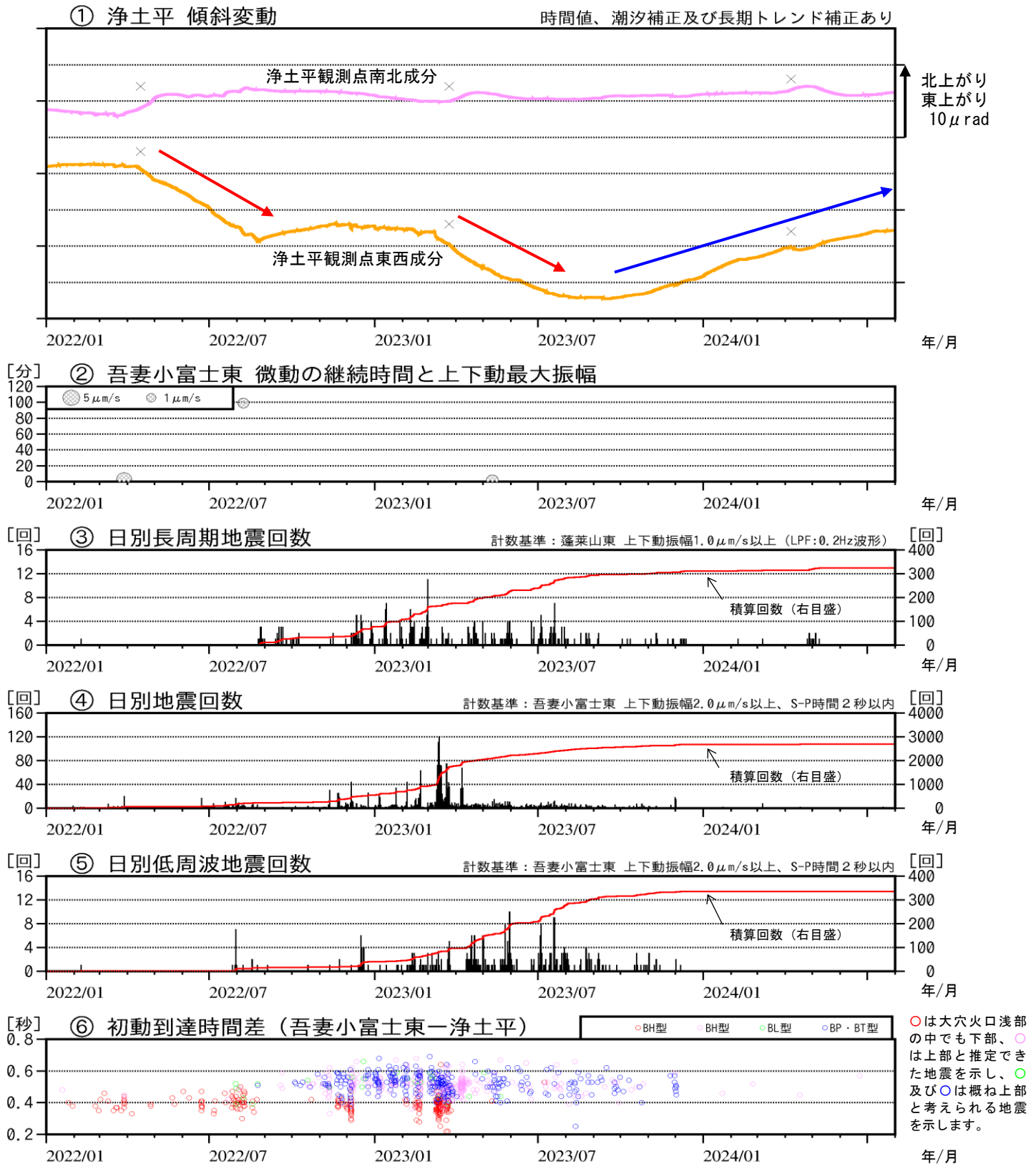
図3 吾妻山 火山活動経過図（2022年1月～2024年7月）
