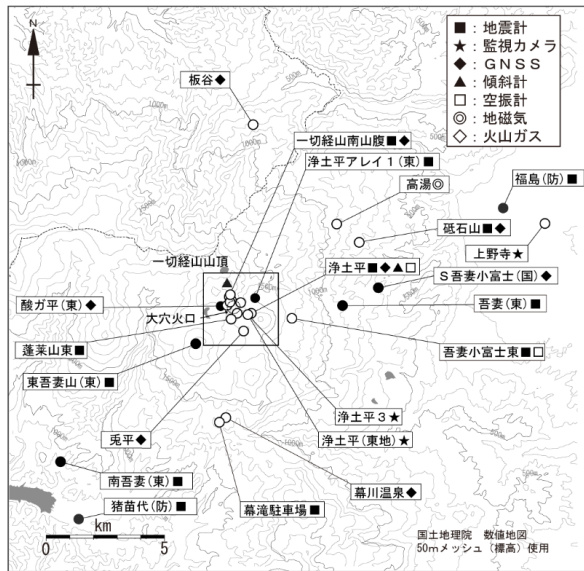
図12 吾妻山 観測点配置図
