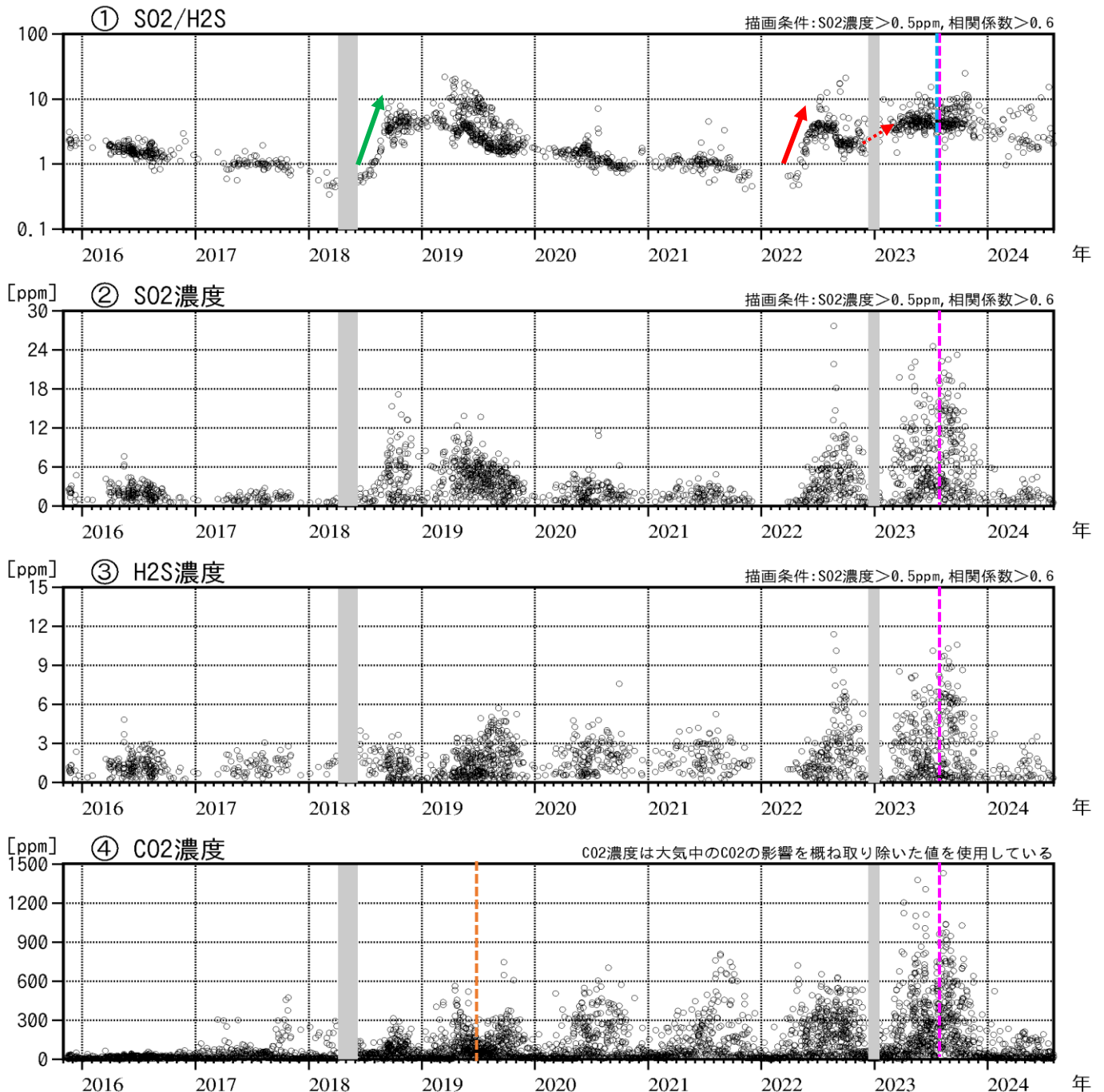
図9 吾妻山 火山ガス観測装置による観測（2015年11月～2024年7月）
