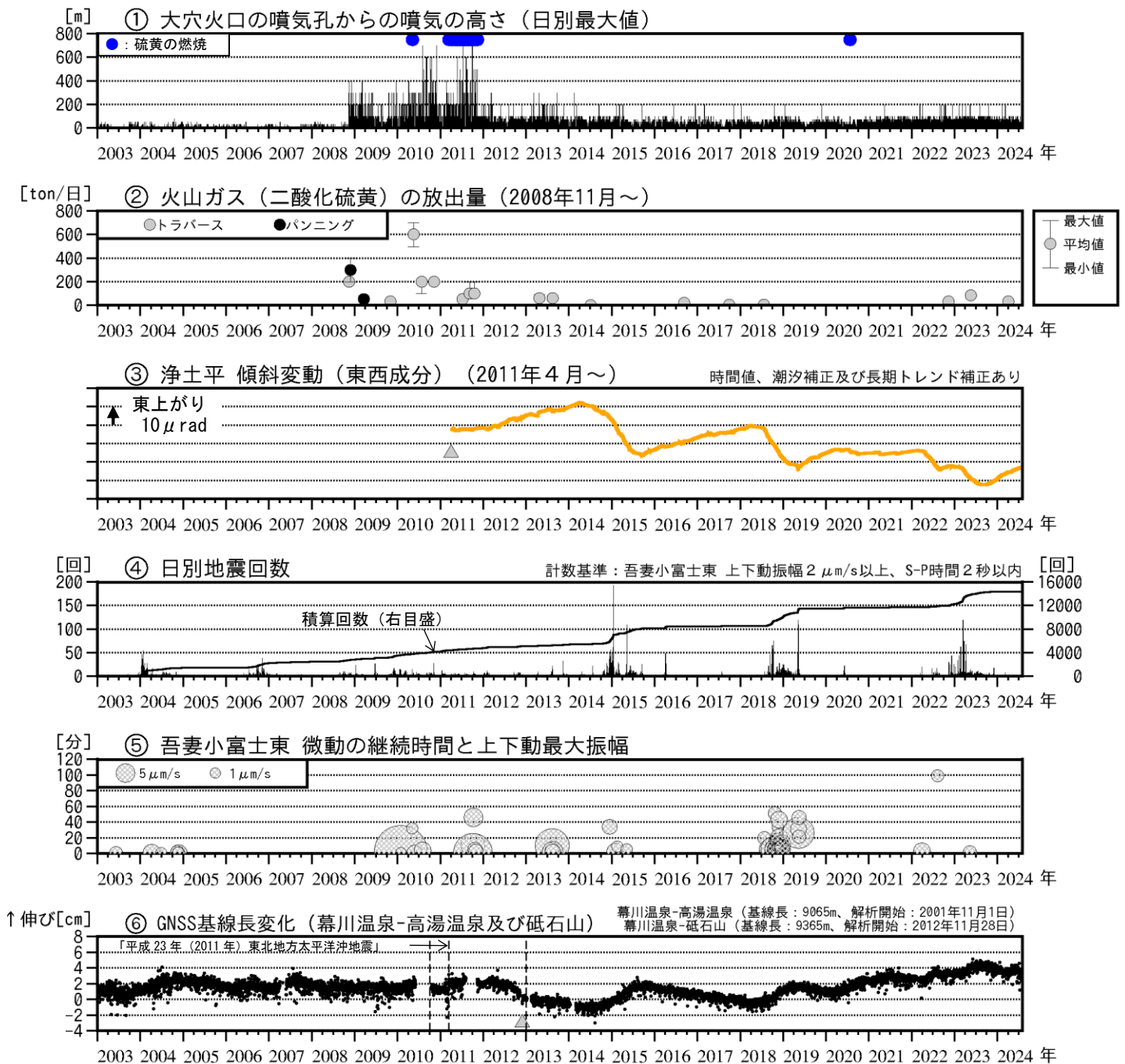
図2 吾妻山 中期的な火山活動の経過（2003年1月～2024年7月）
