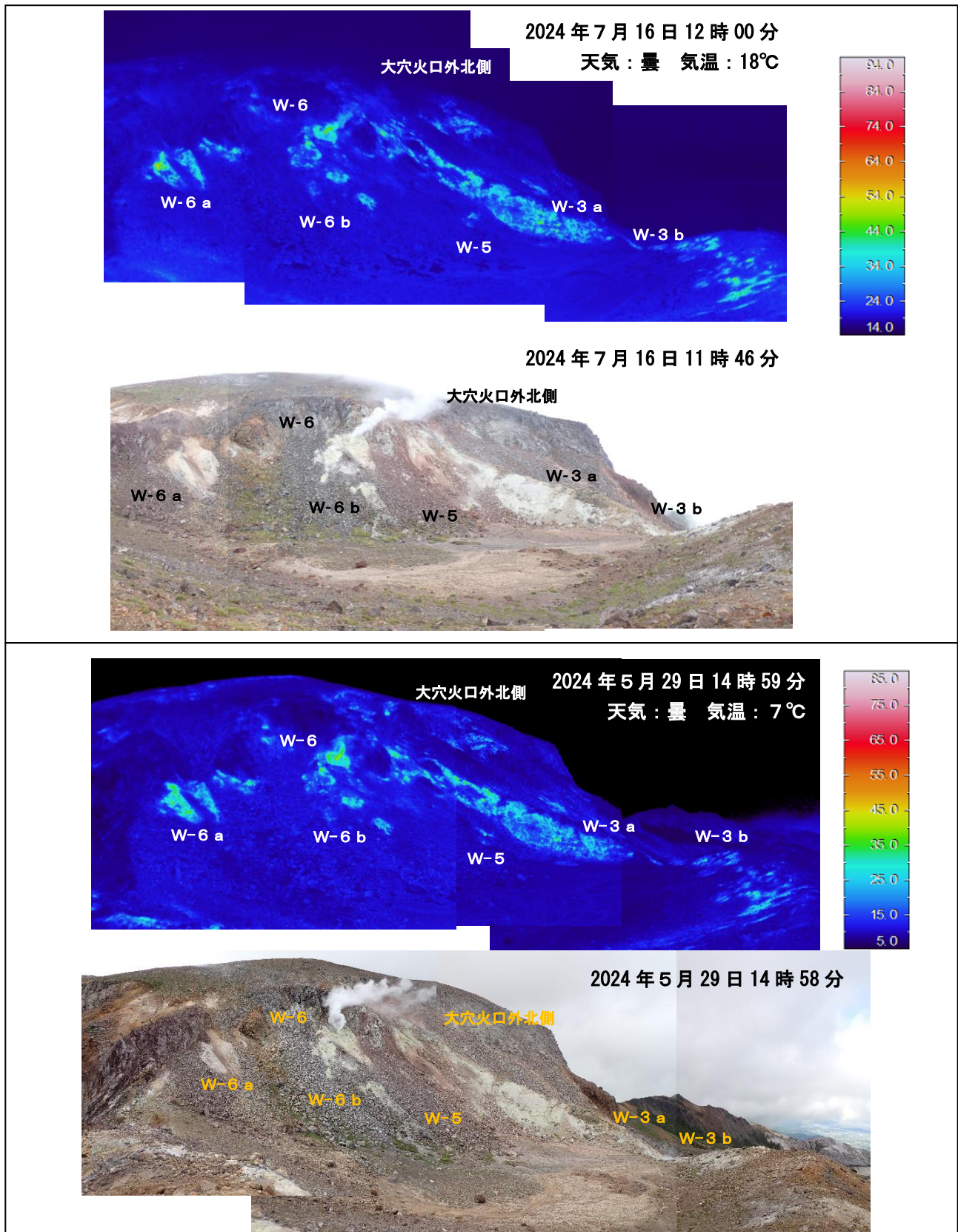
図7 吾妻山 大穴火口付近及びその周辺の状況（下）と地表面温度分布（上）
