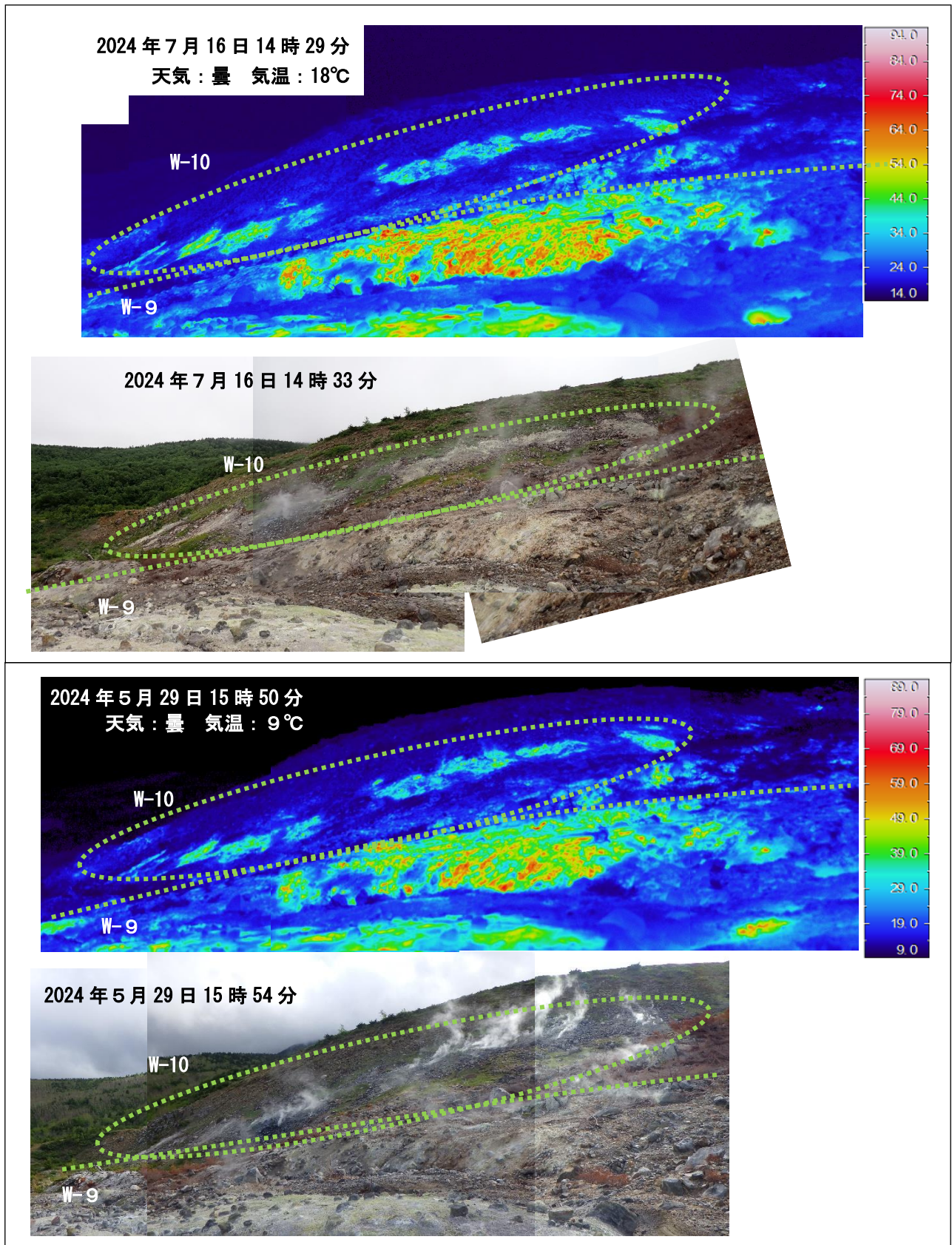
図8 吾妻山 八幡焼の状況（下）と地表面温度分布（上）
