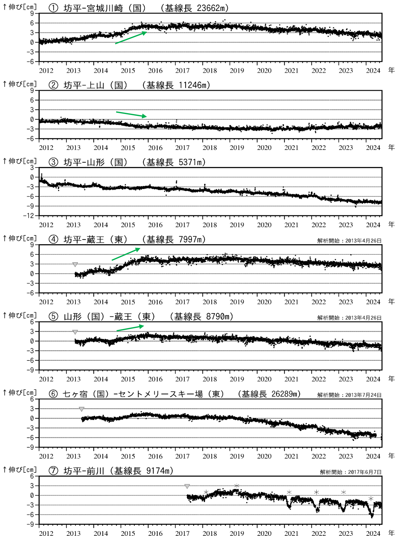
図3 蔵王山 GNSS 基線長変化図 (2012年1月～2024年7月)
