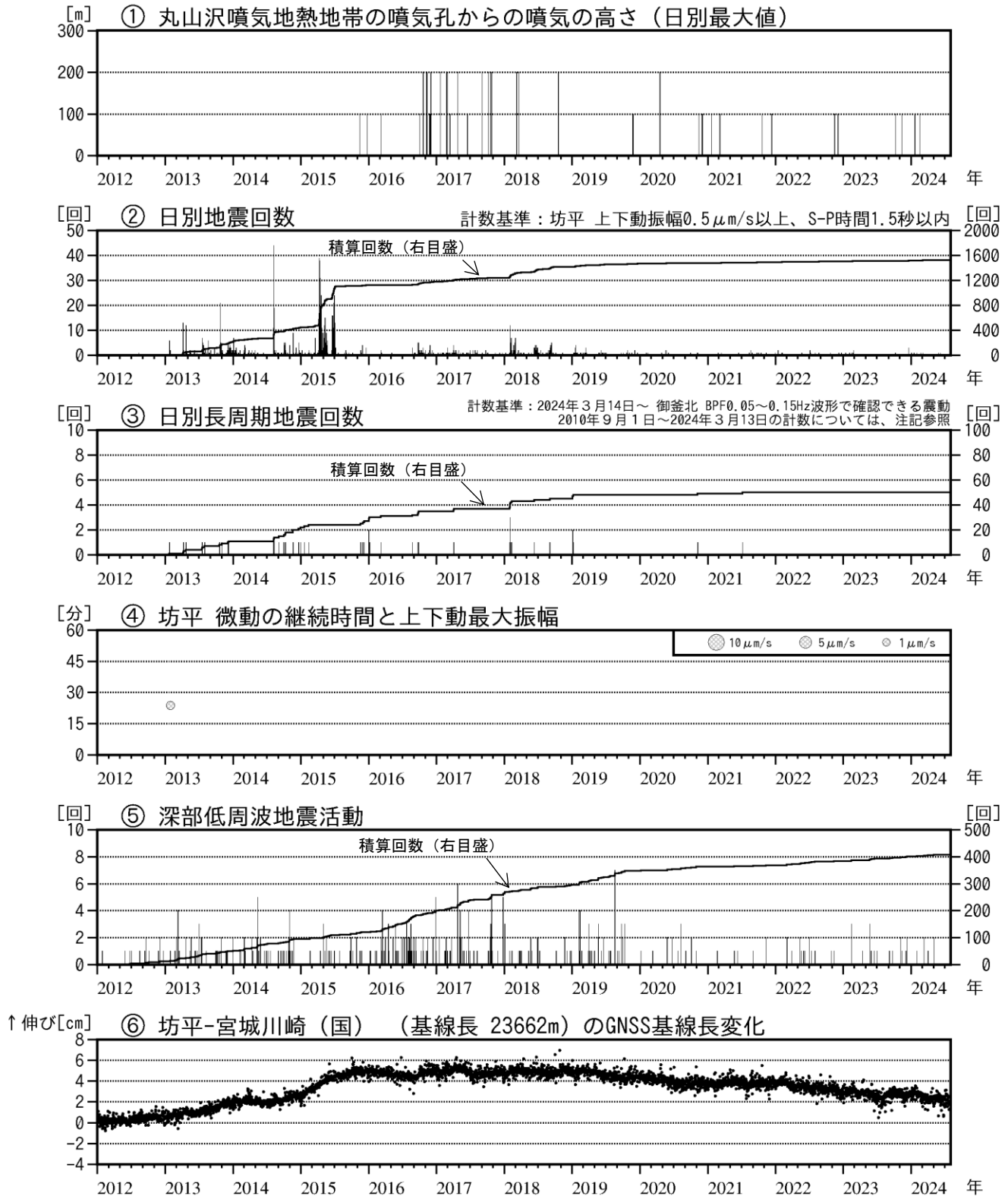
図2 蔵王山 火山活動経過図（2012年1月～2024年7月）
