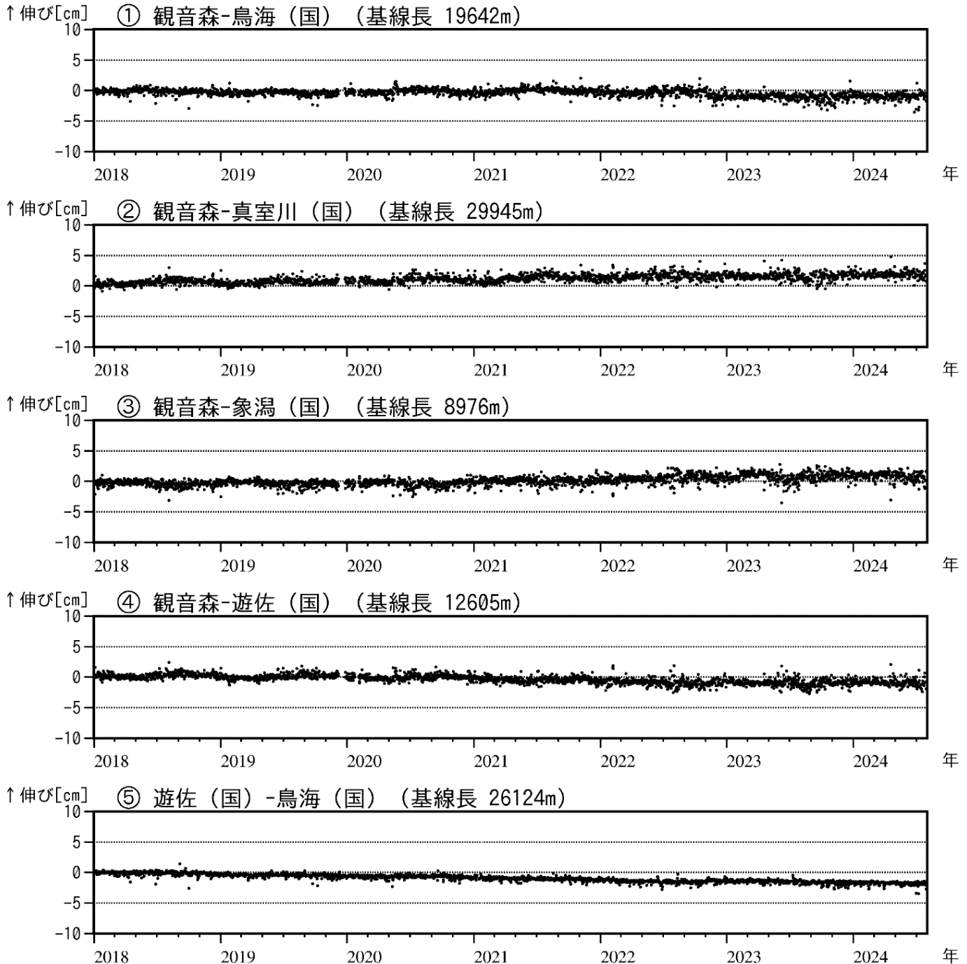
図4 鳥海山 GNSS 基線長変化図（2018年1月～2024年7月）
