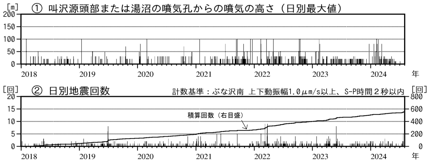
図3 秋田焼山 火山活動経過図（2018年1月～2024年7月）
