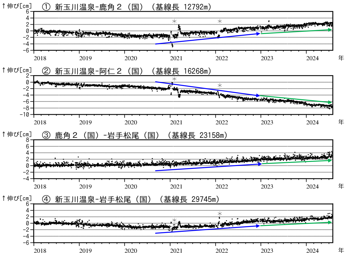
図4 秋田焼山 GNSS 基線長変化図（2018年1月～2024年7月）
