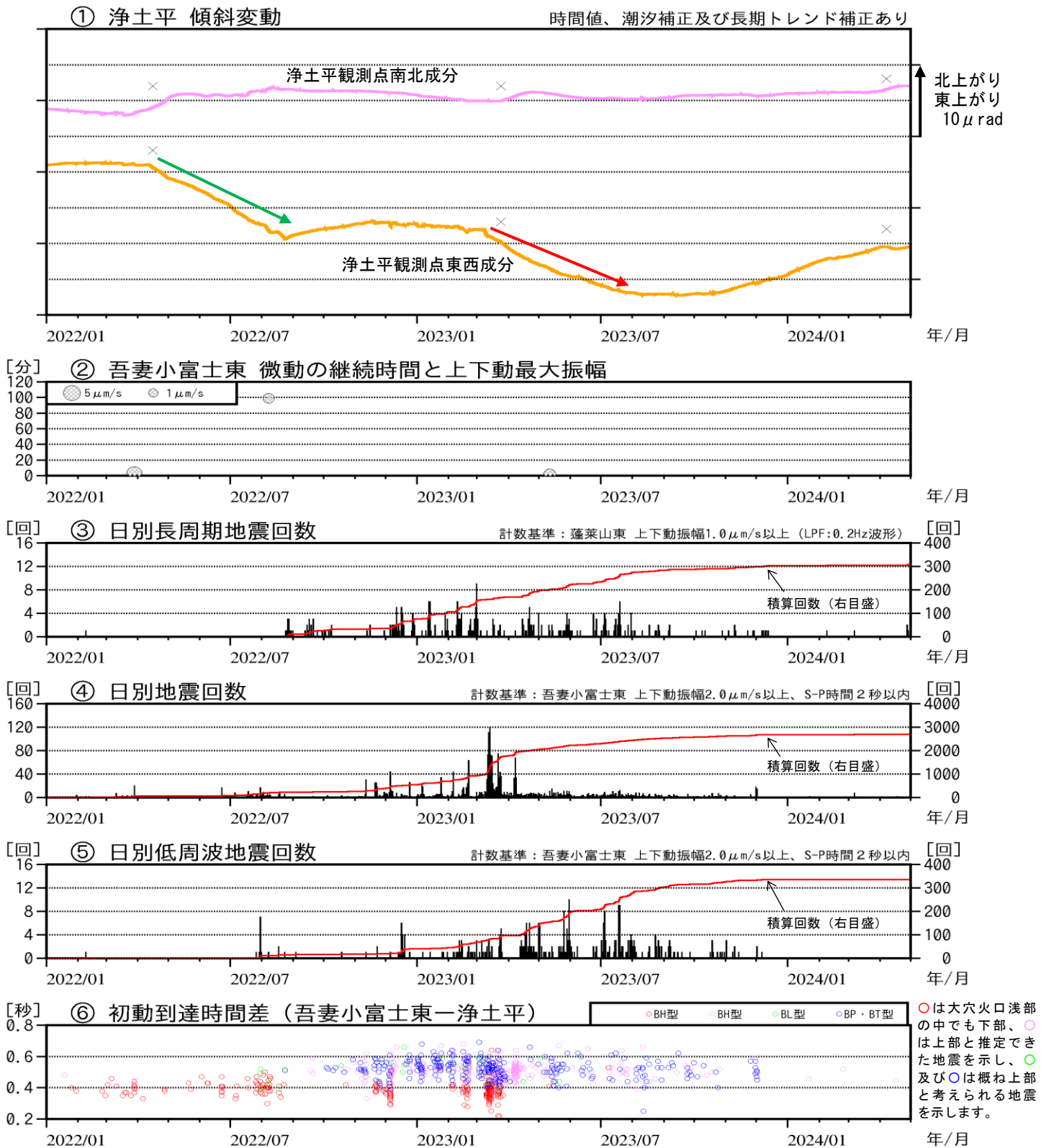
図3 吾妻山 火山活動経過図 (2022年1月~2024年4月)
