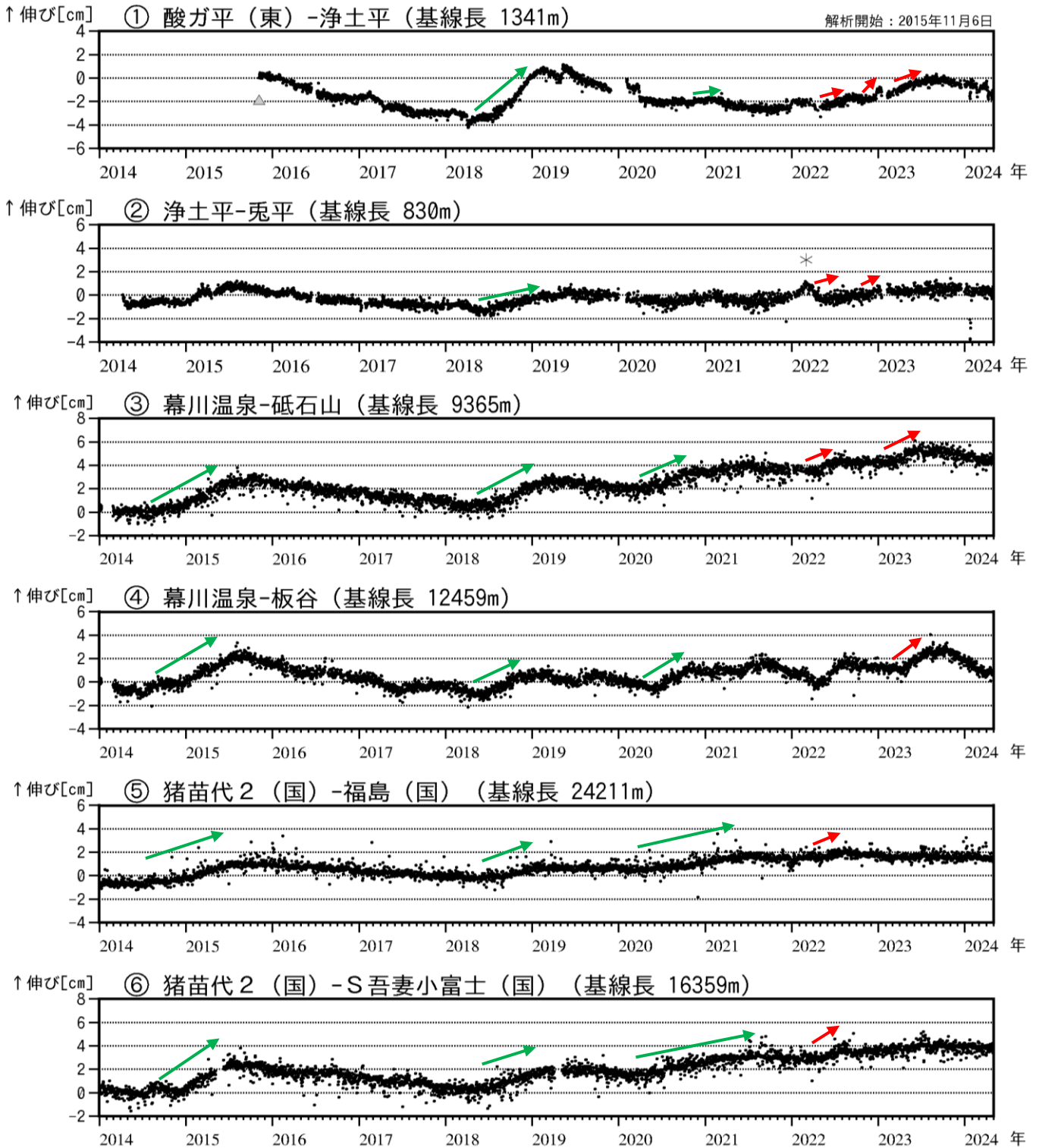
図4 吾妻山 吾妻山浅部・深部の地殻変動（2014年1月～2024年4月）
