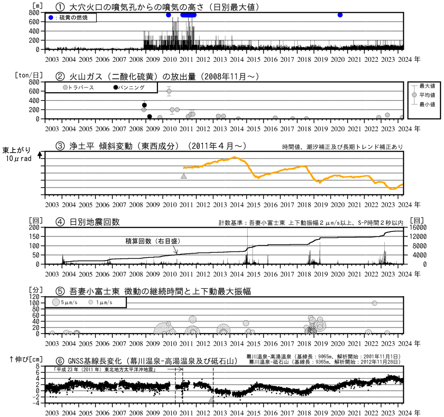
図2 吾妻山 中期的な火山活動の経過（2003年1月～2024年4月）
