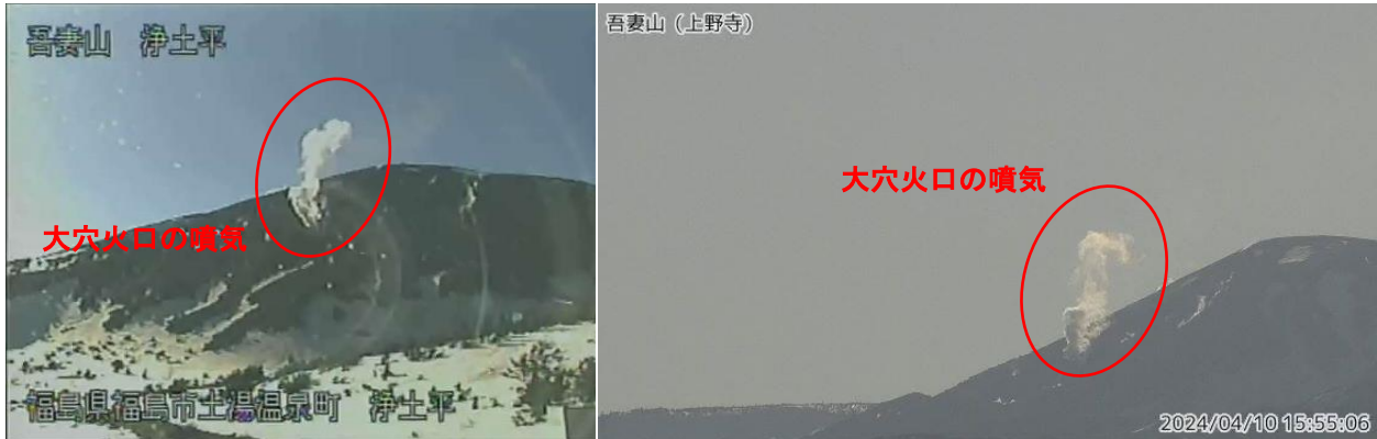
図1 吾妻山 大穴火口周辺の噴気の状態（4月10日）
