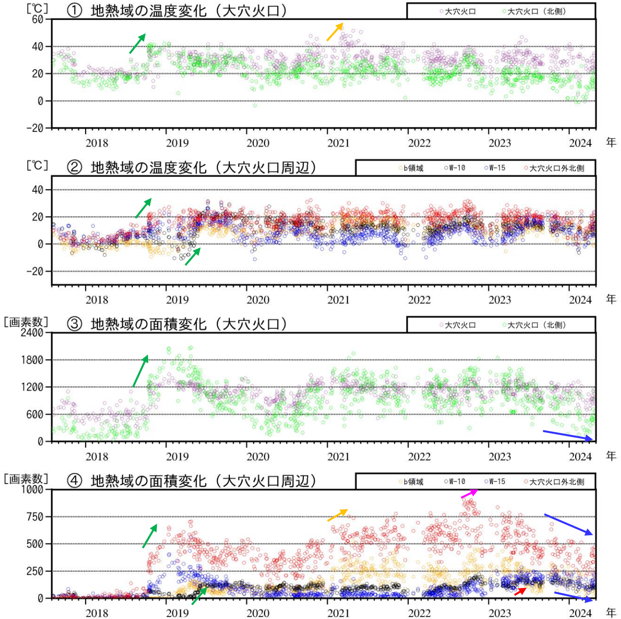
図5 吾妻山 監視カメラによる大穴火口周辺の地熱域の経過（2017年8月～2024年4月）
