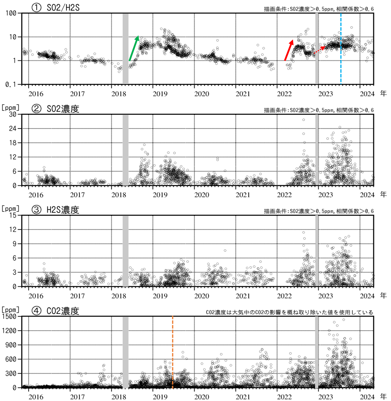
図6 吾妻山 火山ガス観測装置による観測（2015年11月～2024年4月）
