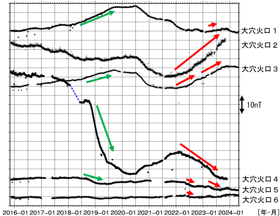
図7 吾妻山 全磁力連続観測点の全磁力値変化（2015年11月～2024年4月）
