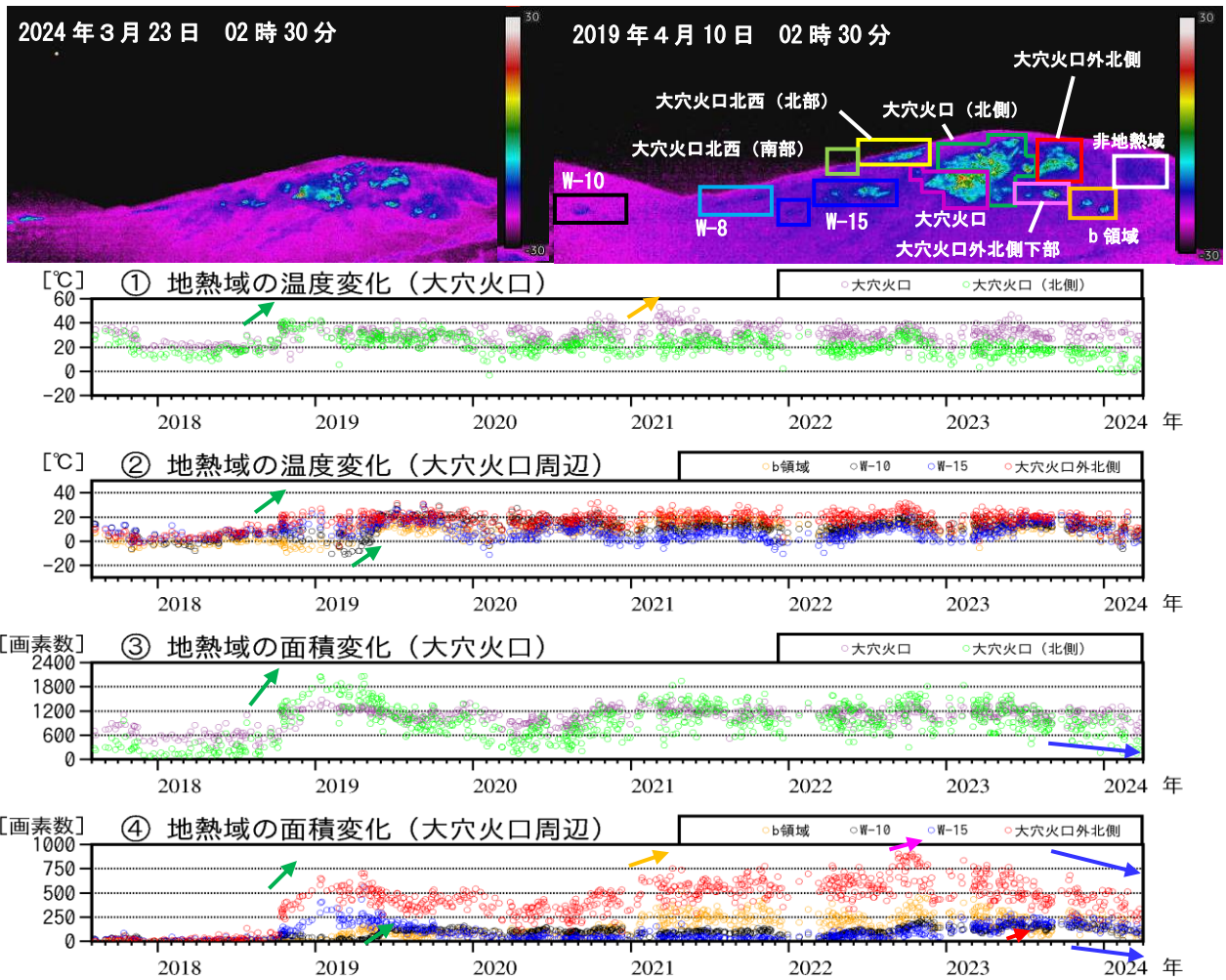
図4 吾妻山 監視カメラによる大穴火口周辺の地熱域の経過（2017年8月～2024年3月）
