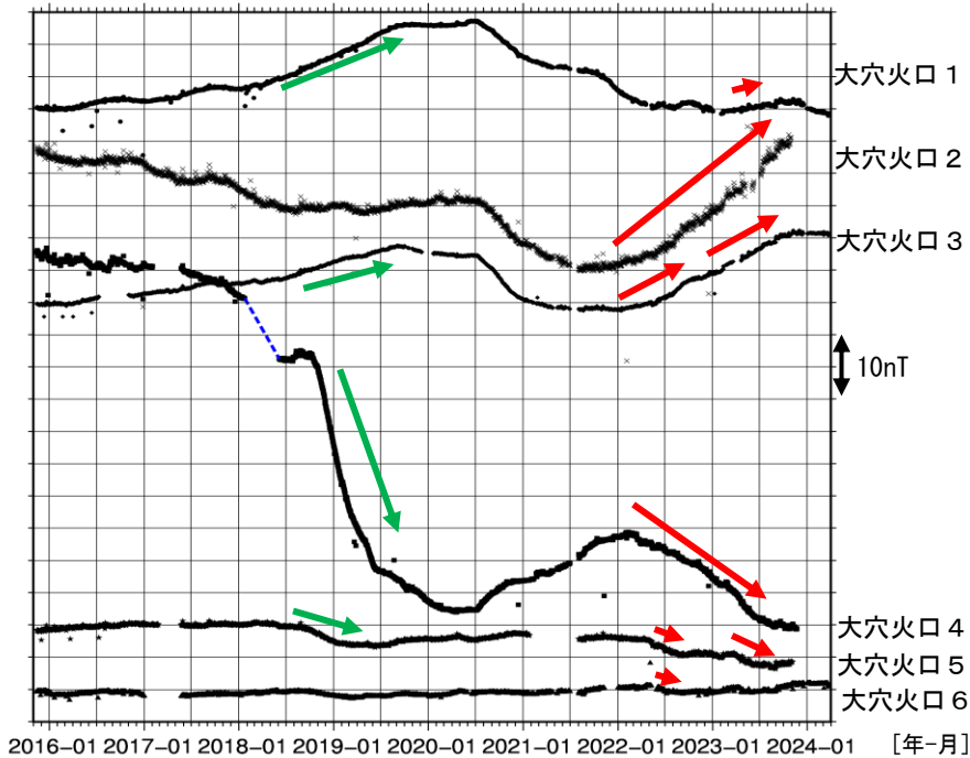
図7 吾妻山 全磁力連続観測点の全磁力値変化（2015年11月～2024年3月）
