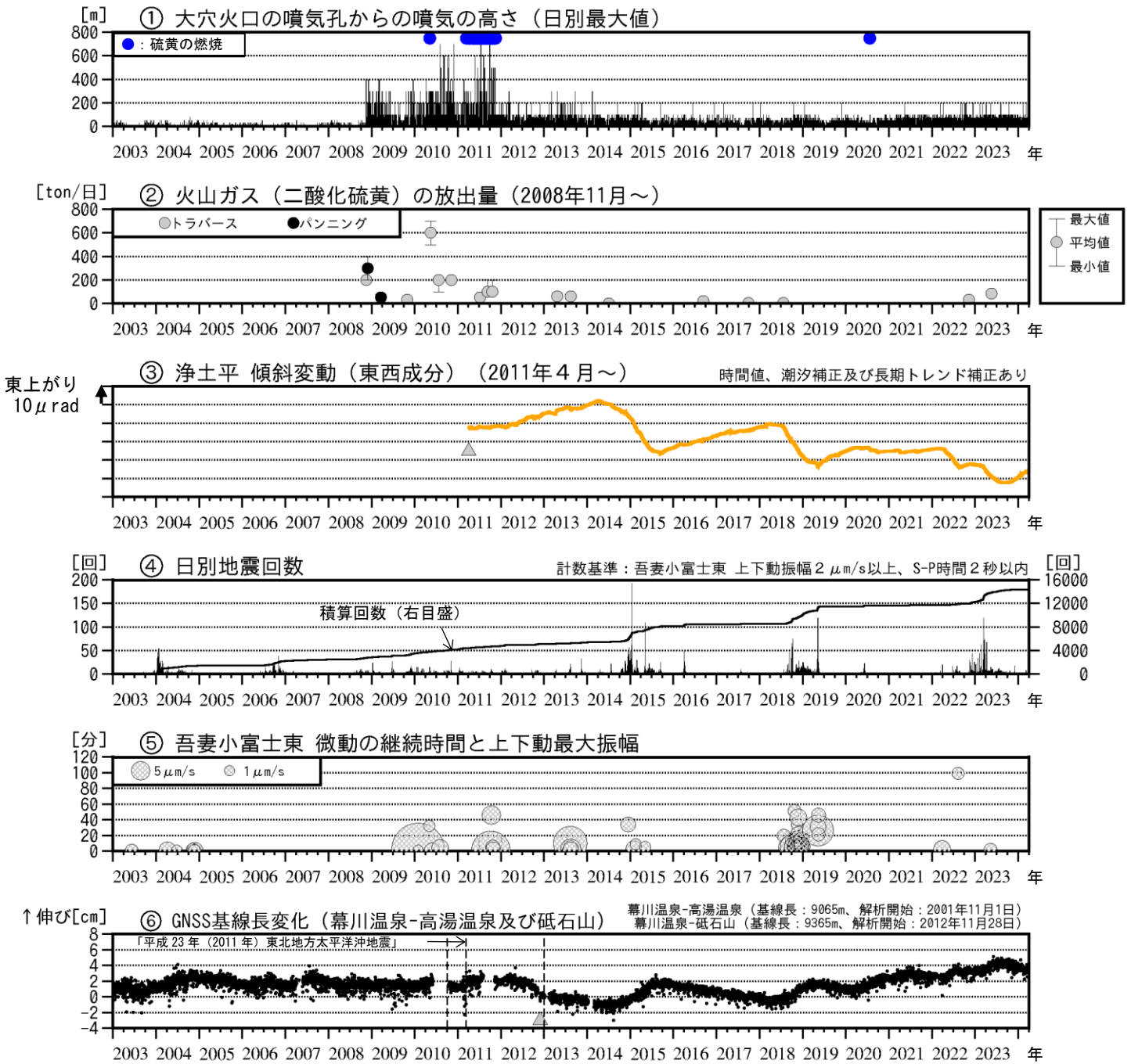
図1 吾妻山 中期的な火山活動の経過（2003年1月～2024年3月）
