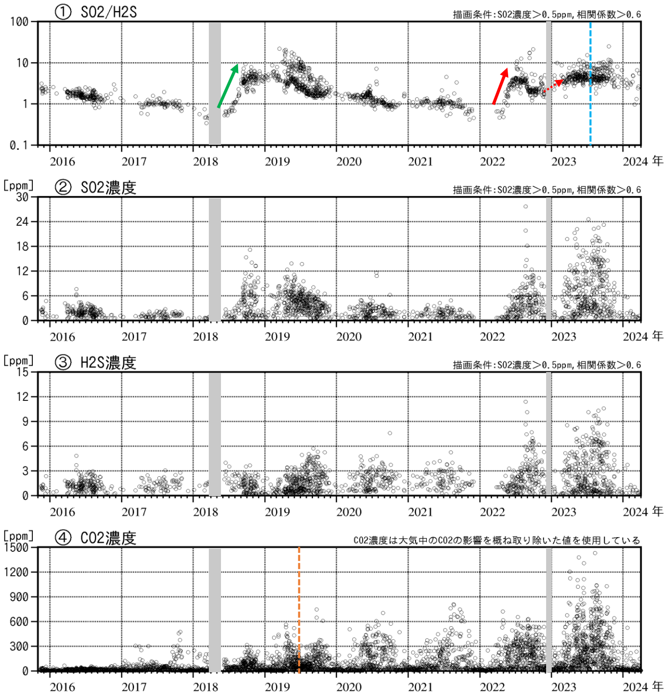
図6 吾妻山 火山ガス観測装置による観測（2015年11月～2024年3月）
