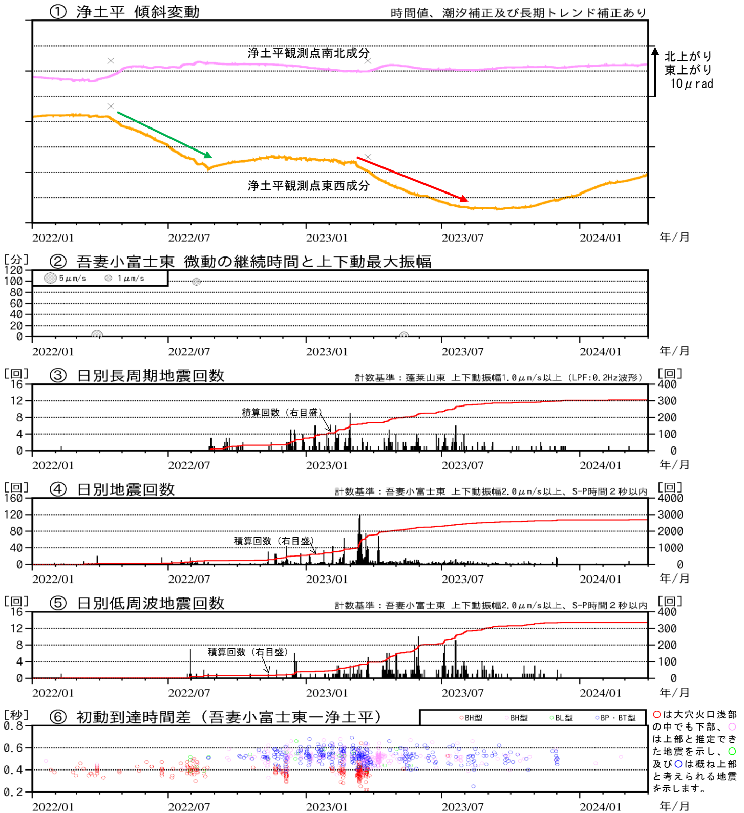
図2 吾妻山 火山活動経過図（2022年1月～2024年3月）
