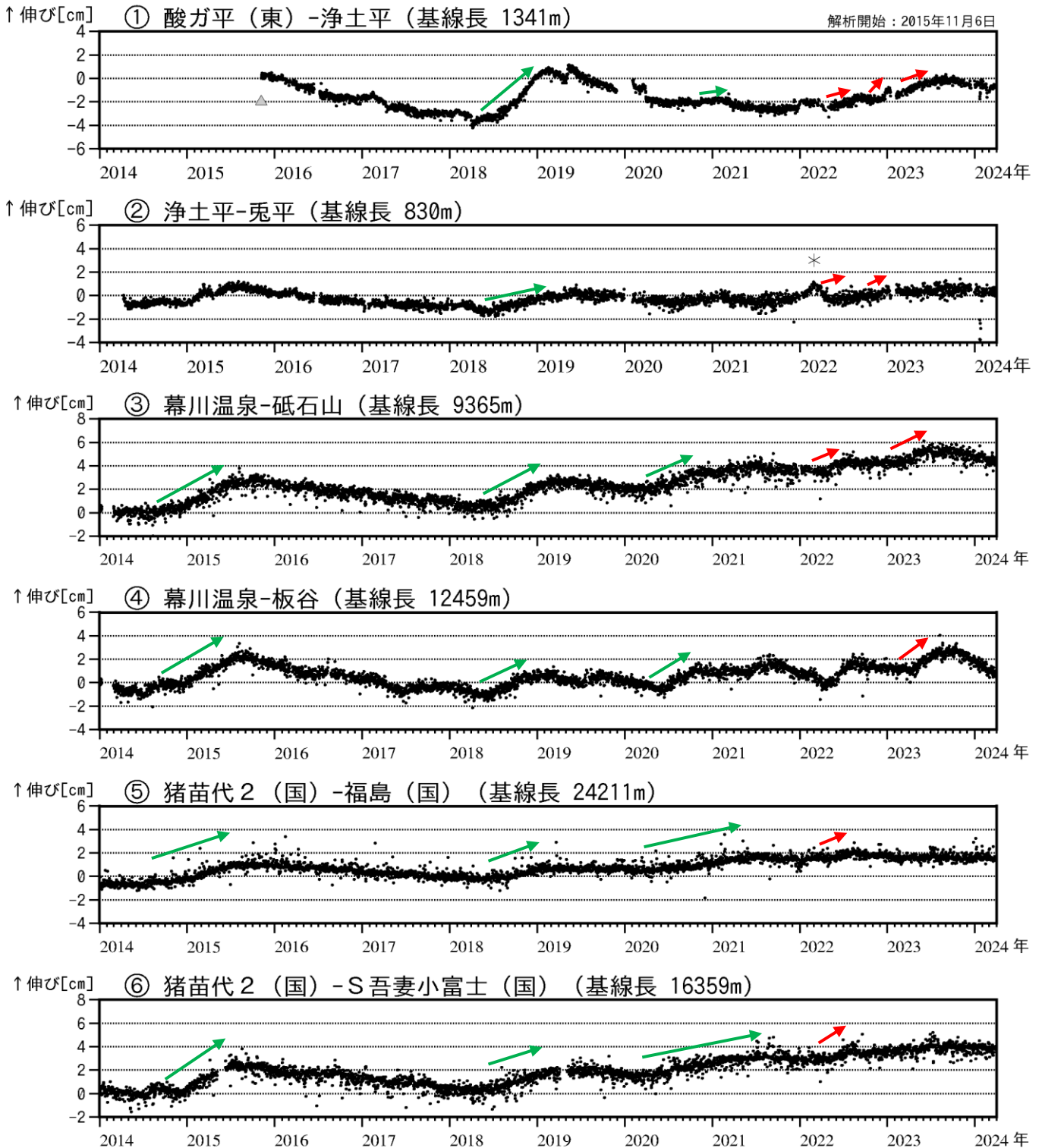
図3 吾妻山 吾妻山浅部・深部の地殻変動（2014年1月～2024年3月）
