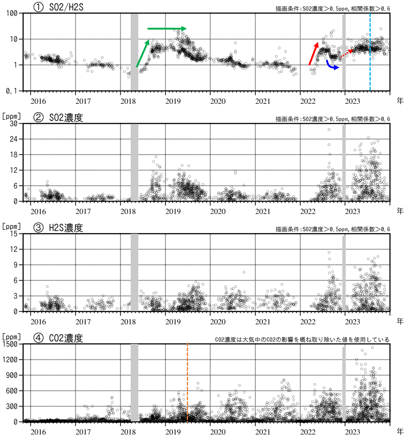
図6 吾妻山 火山ガス観測装置による観測（2015年11月～2023年12月）
