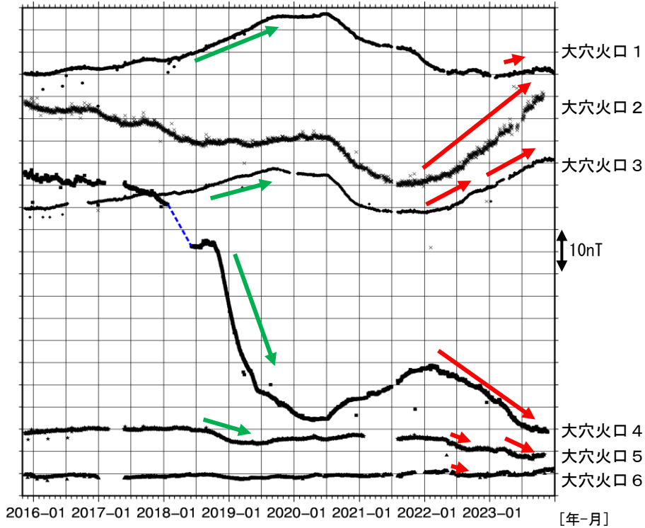
図7 吾妻山 全磁力連続観測点の全磁力値変化（2015年11月～2023年12月）
