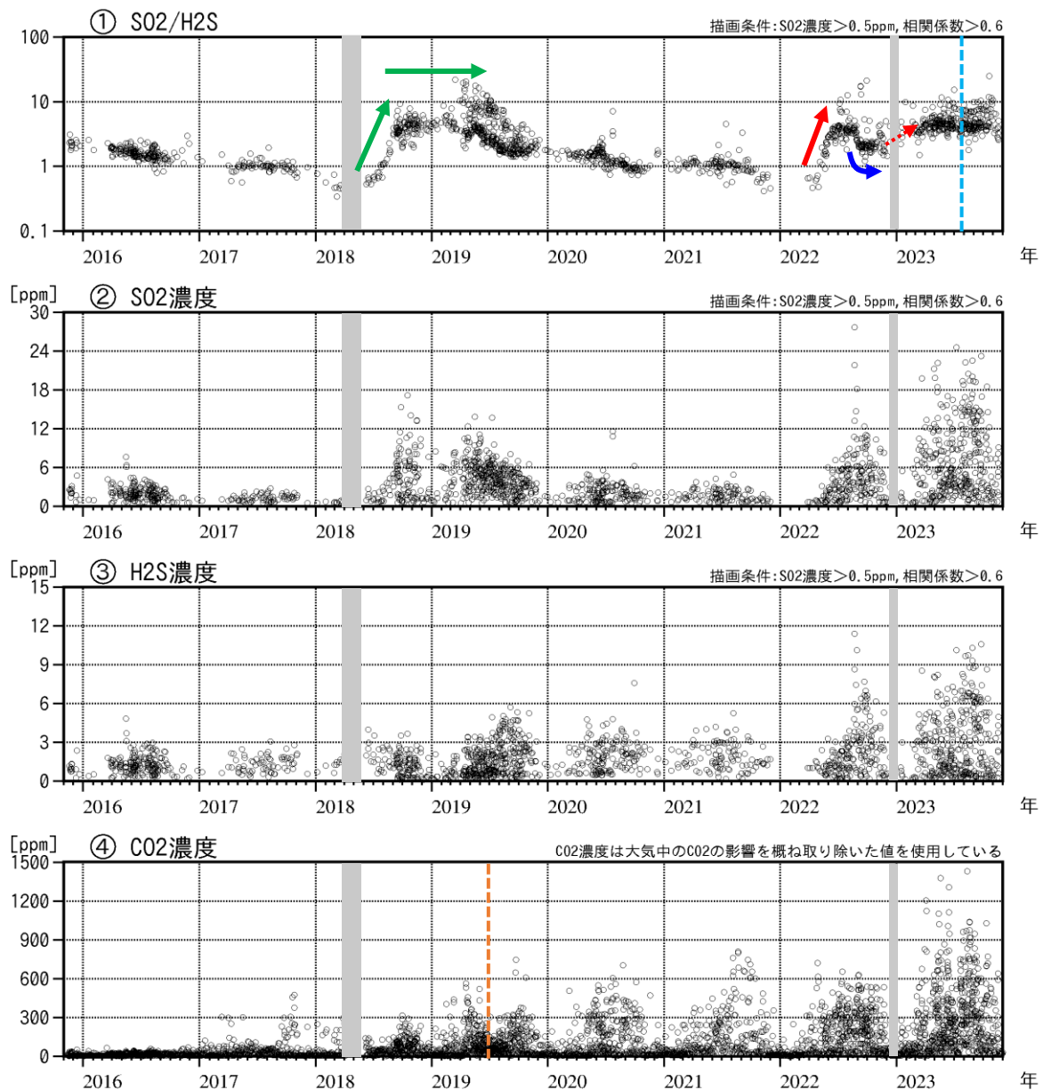
図 11 吾妻山 火山ガス観測装置による観測（2015年11月～2023年11月）
