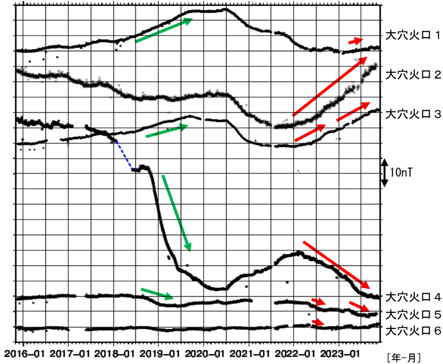
図 12 吾妻山 全磁力連続観測点の全磁力値変化（2015年11月～2023年11月）
