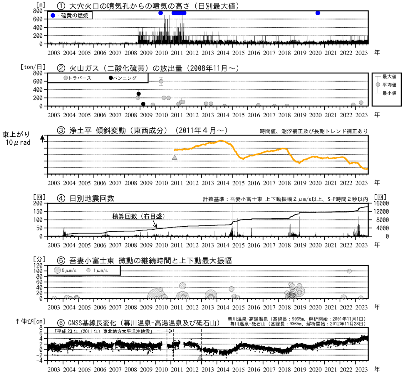
図1 吾妻山 中期的な火山活動の経過（2003年1月～2023年10月）
