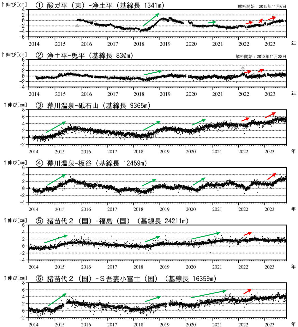
図3 吾妻山 吾妻山浅部・深部の地殻変動（2014年1月～2023年10月）
