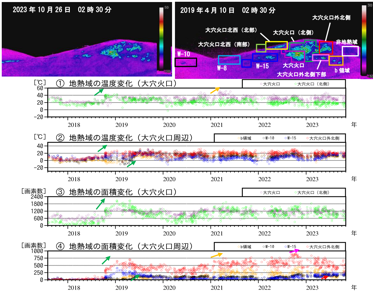
図4 吾妻山 監視カメラによる大穴火口周辺の地熱域の経過（2017年8月～2023年10月）
