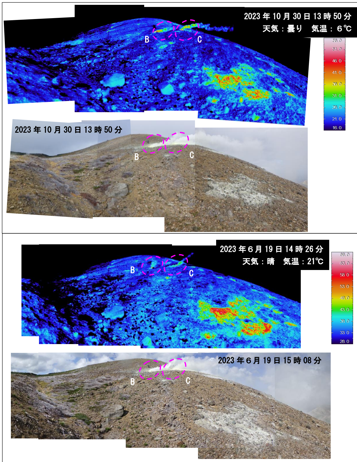
図7 吾妻山 大穴火口北西の状況（下）と地表面温度分布（上）
