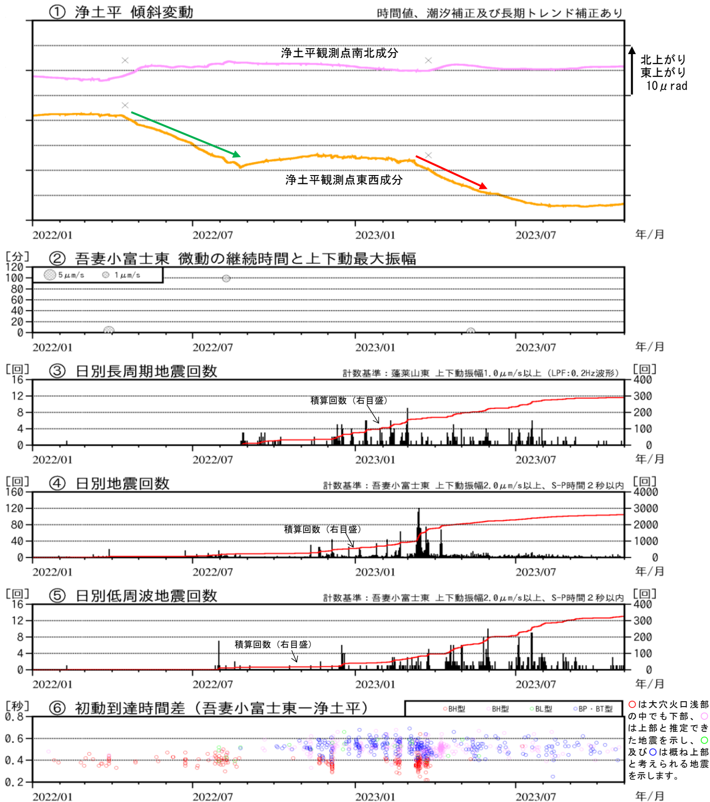
図2 吾妻山 火山活動経過図（2022年1月～2023年10月）
