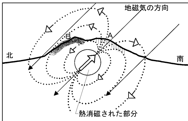
図10 熱消磁に伴う全磁力変化のモデル
