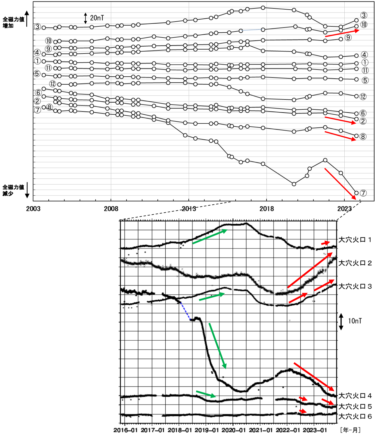
図9 吾妻山 全磁力繰り返し観測（上）及び連続観測（下）の全磁力値変化 （2003年9月～2023年10月）
