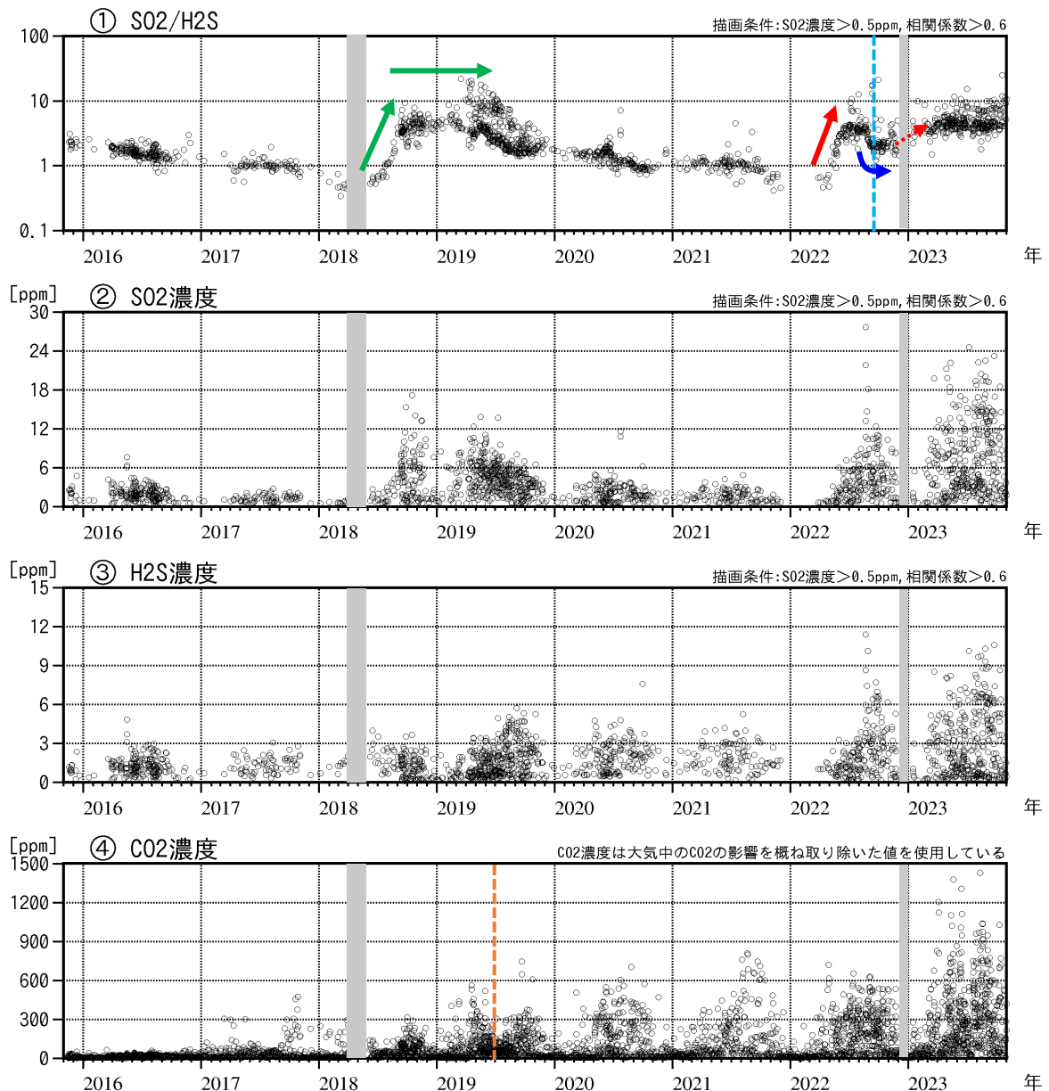
図8 吾妻山 火山ガス観測装置による観測（2015年11月～2023年10月）
