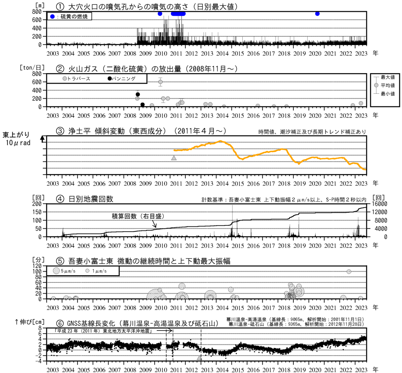
図1 吾妻山 中期的な火山活動の経過（2003年1月～2023年9月）
