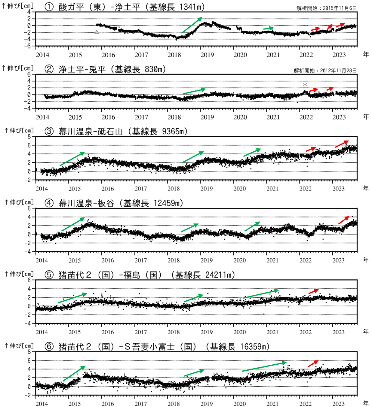
図3 吾妻山 吾妻山浅部・深部の地殻変動（2014年1月～2023年9月）
