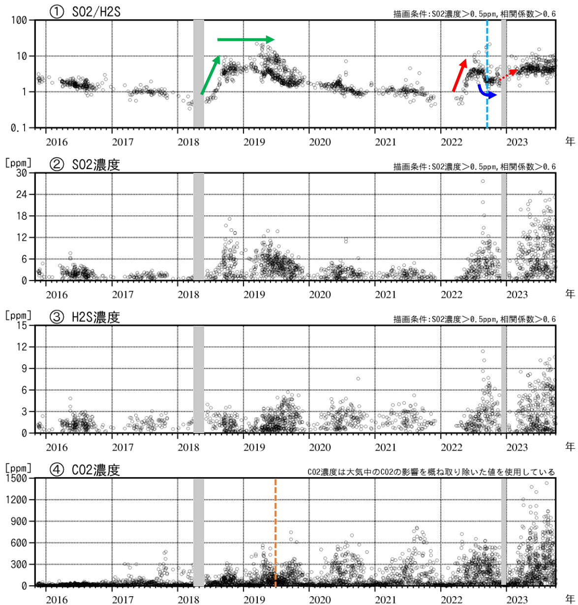
図6 吾妻山 火山ガス観測装置による観測（2015年11月～2023年9月）
