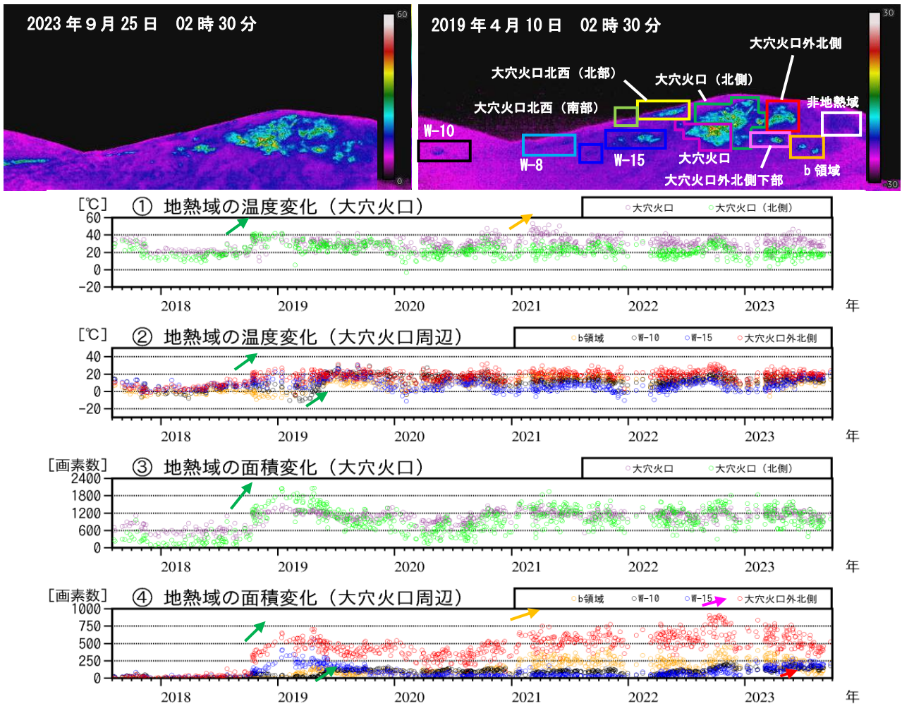
図4 吾妻山 監視カメラによる大穴火口周辺の地熱域の経過（2017年8月～2023年9月）
