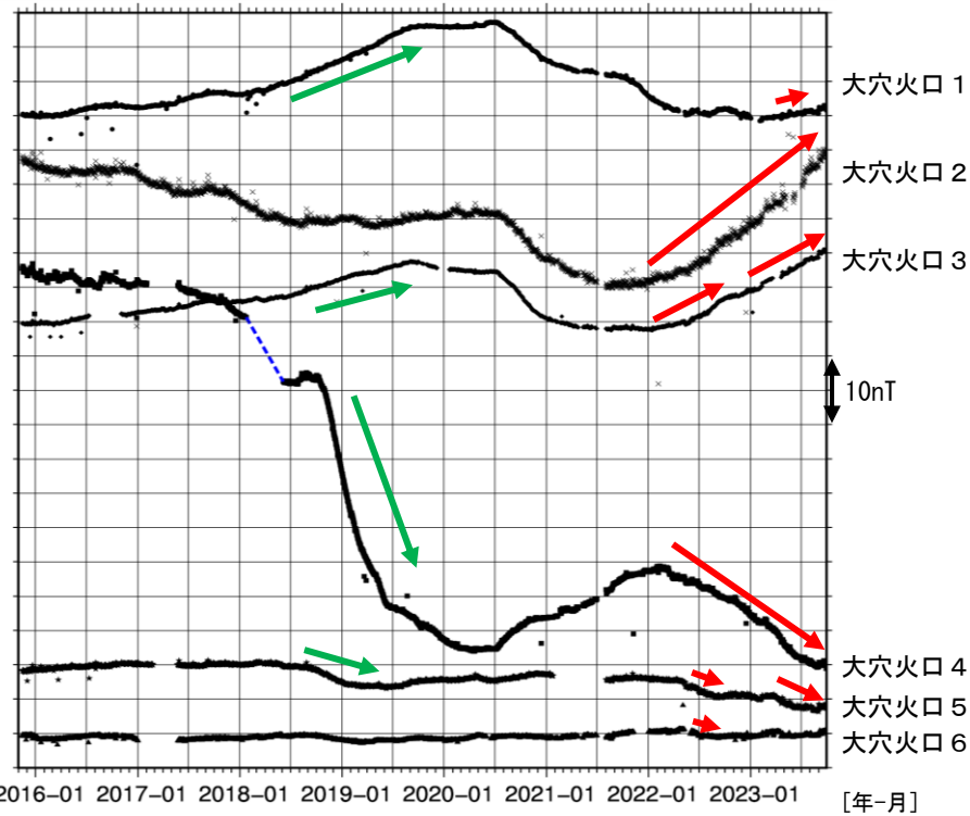
図7 吾妻山 全磁力連続観測点の全磁力値変化（2015年11月～2023年9月）
