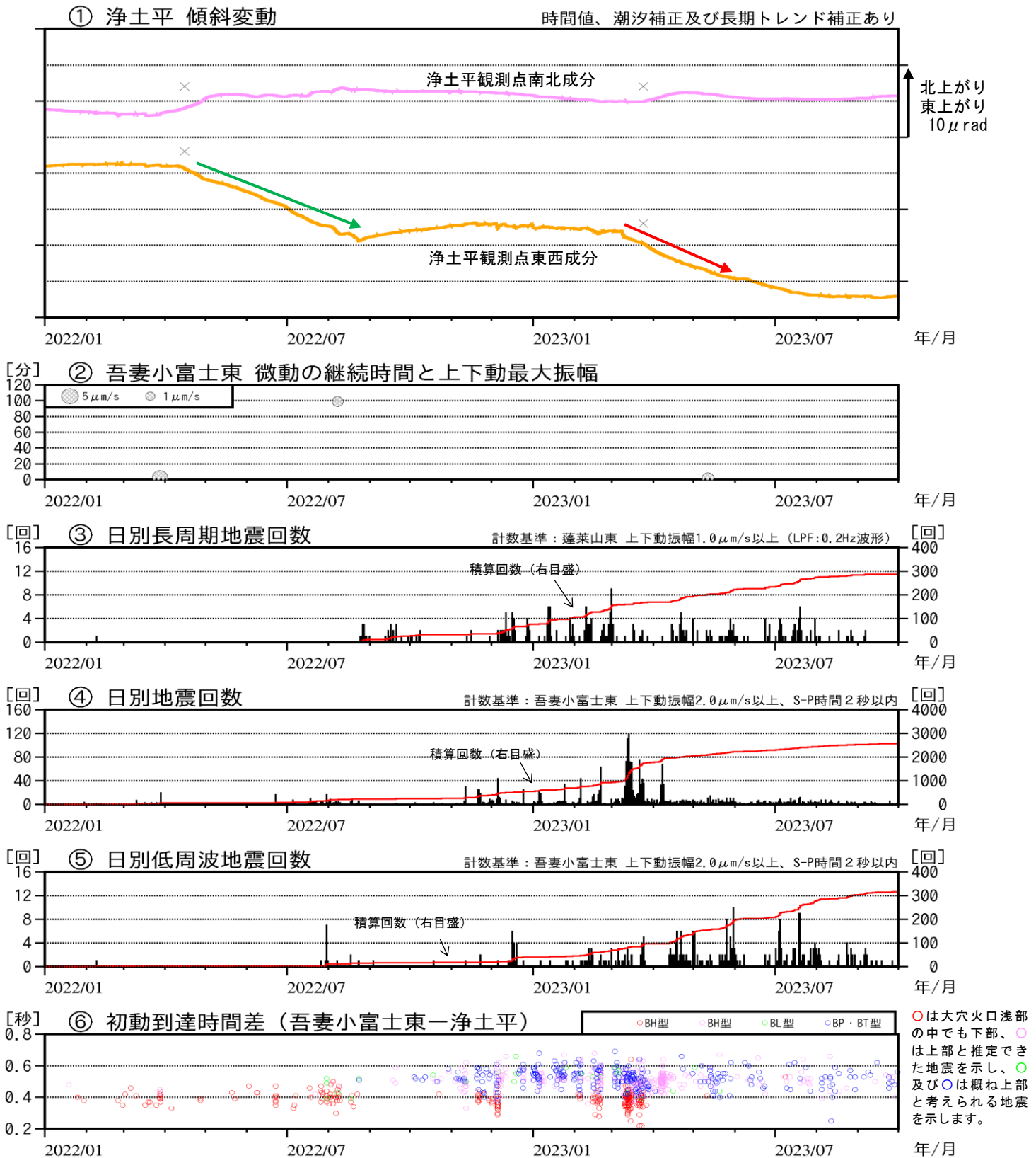
図2 吾妻山 火山活動経過図（2022年1月～2023年9月）
