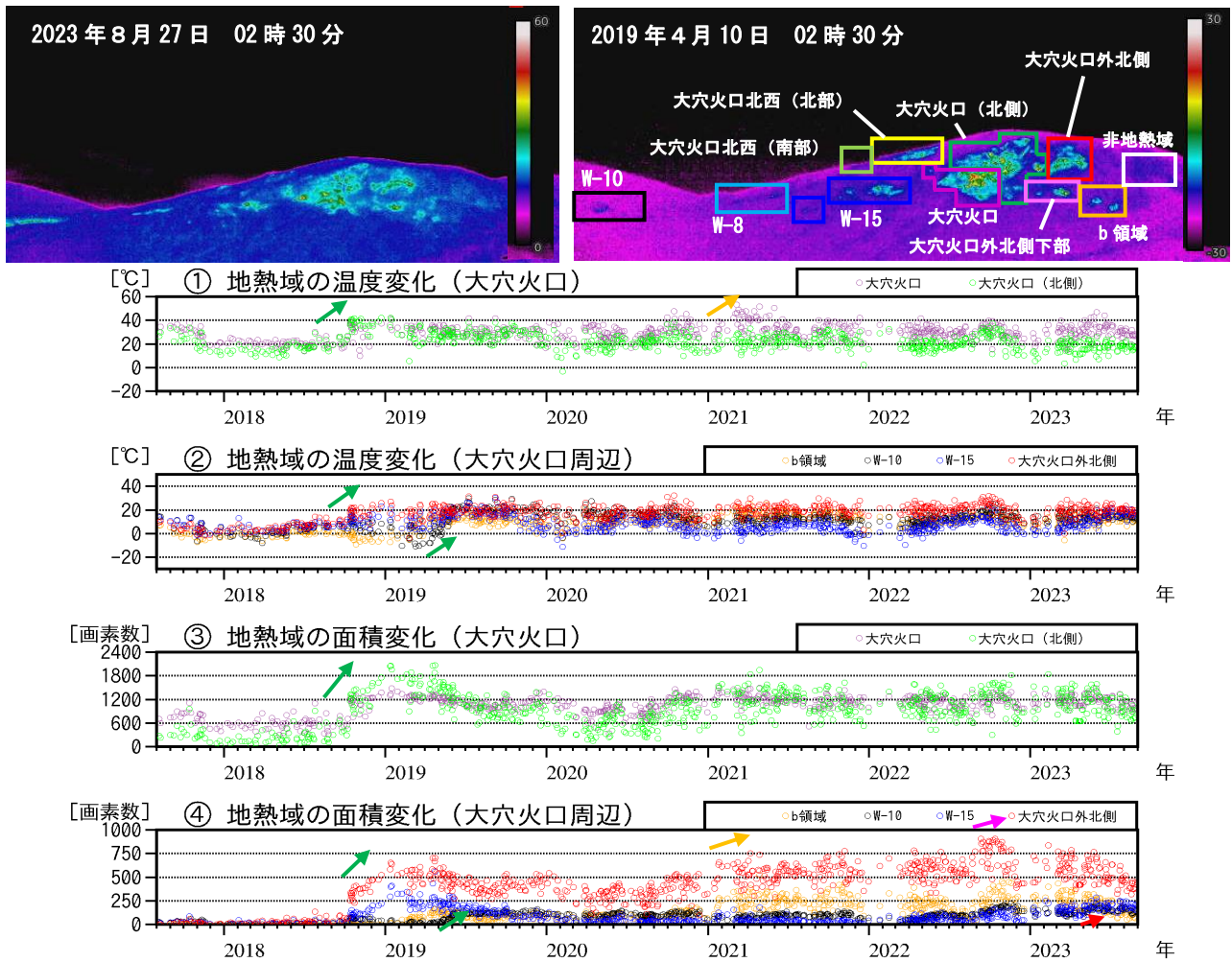
図4 吾妻山 監視カメラによる大穴火口周辺の地熱域の経過（2017年8月～2023年8月）
