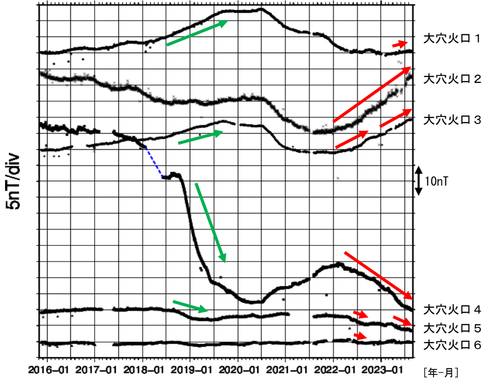
図7 吾妻山 全磁力連続観測点の全磁力値変化（2015年11月～2023年8月）
