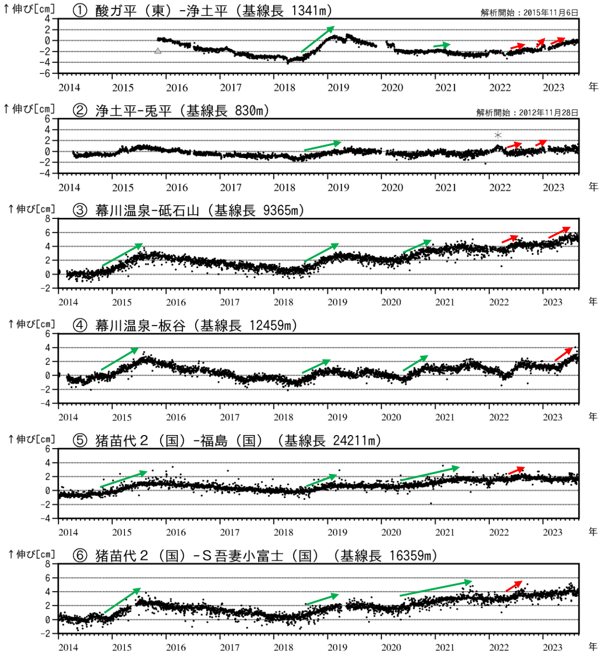
図3 吾妻山 吾妻山浅部・深部の地殻変動（2014年1月～2023年8月）
