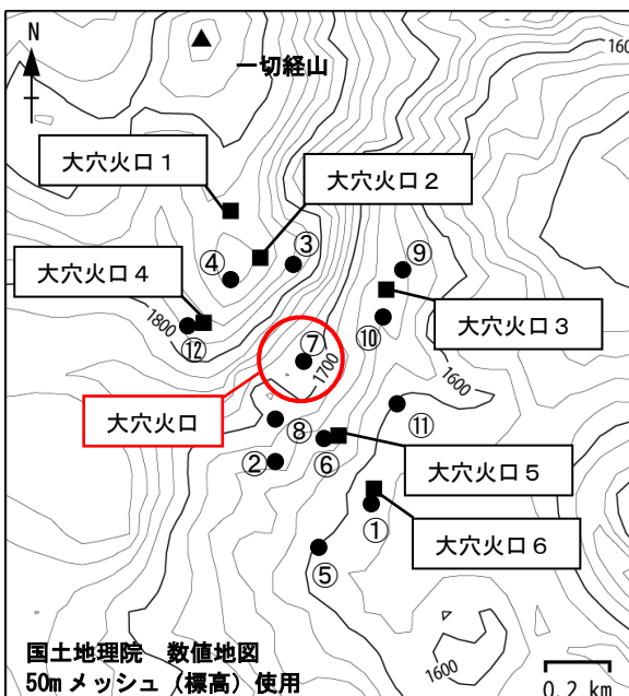
図11 吾妻山 全磁力観測点配置図
