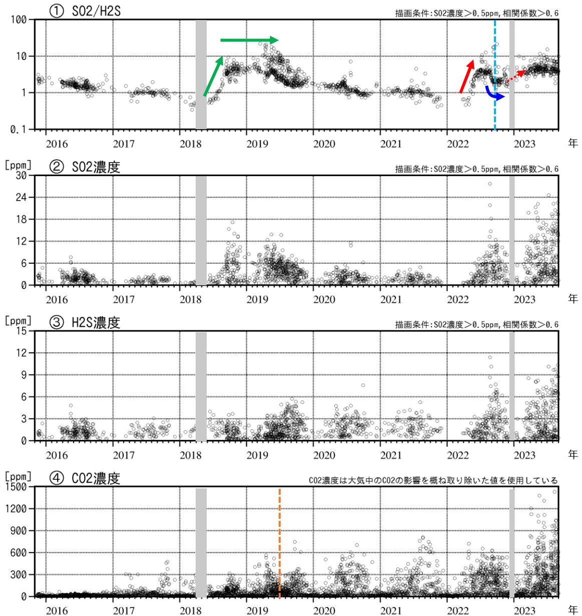
図6 吾妻山 火山ガス観測装置による観測（2015年11月～2023年8月）
