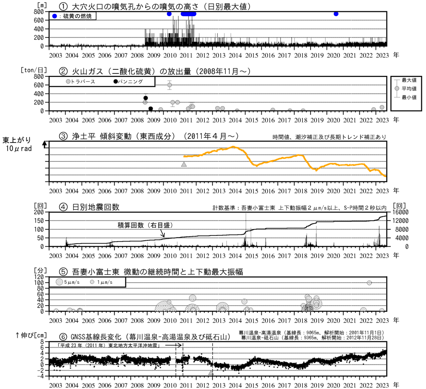
図1 吾妻山 中期的な火山活動の経過（2003年1月～2023年8月）
