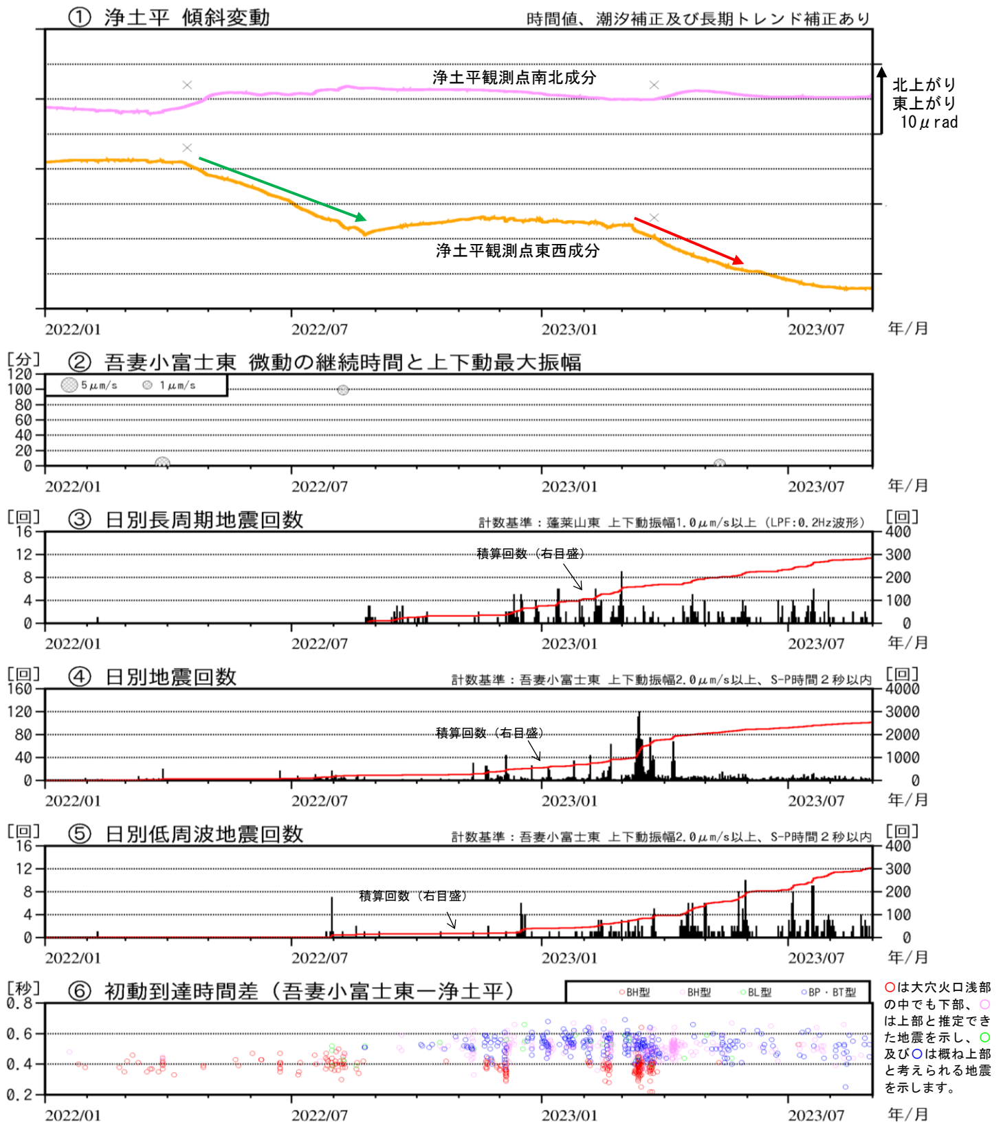
図2 吾妻山 火山活動経過図 (2022年1月~2023年8月)
