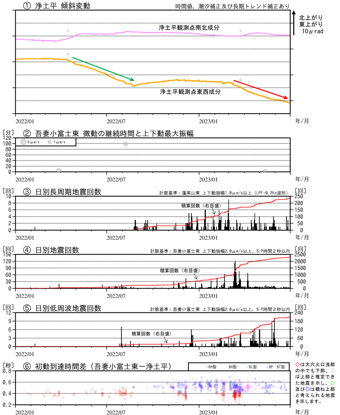
図2 吾妻山 火山活動経過図（2022年1月～2023年6月）
