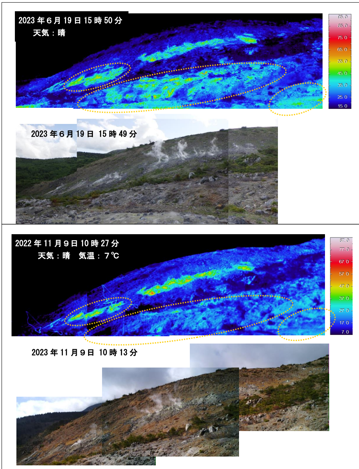
図9 吾妻山 八幡焼の状況（下）と地表面温度分布（上）
