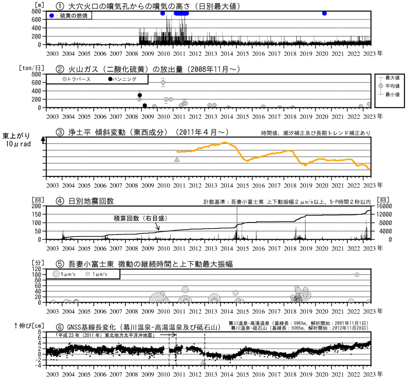
図1 吾妻山 中期的な火山活動の経過（2003年1月～2023年6月）
