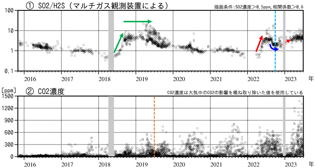
図10 吾妻山 火山ガス観測装置による観測（2015年11月～2023年6月）
