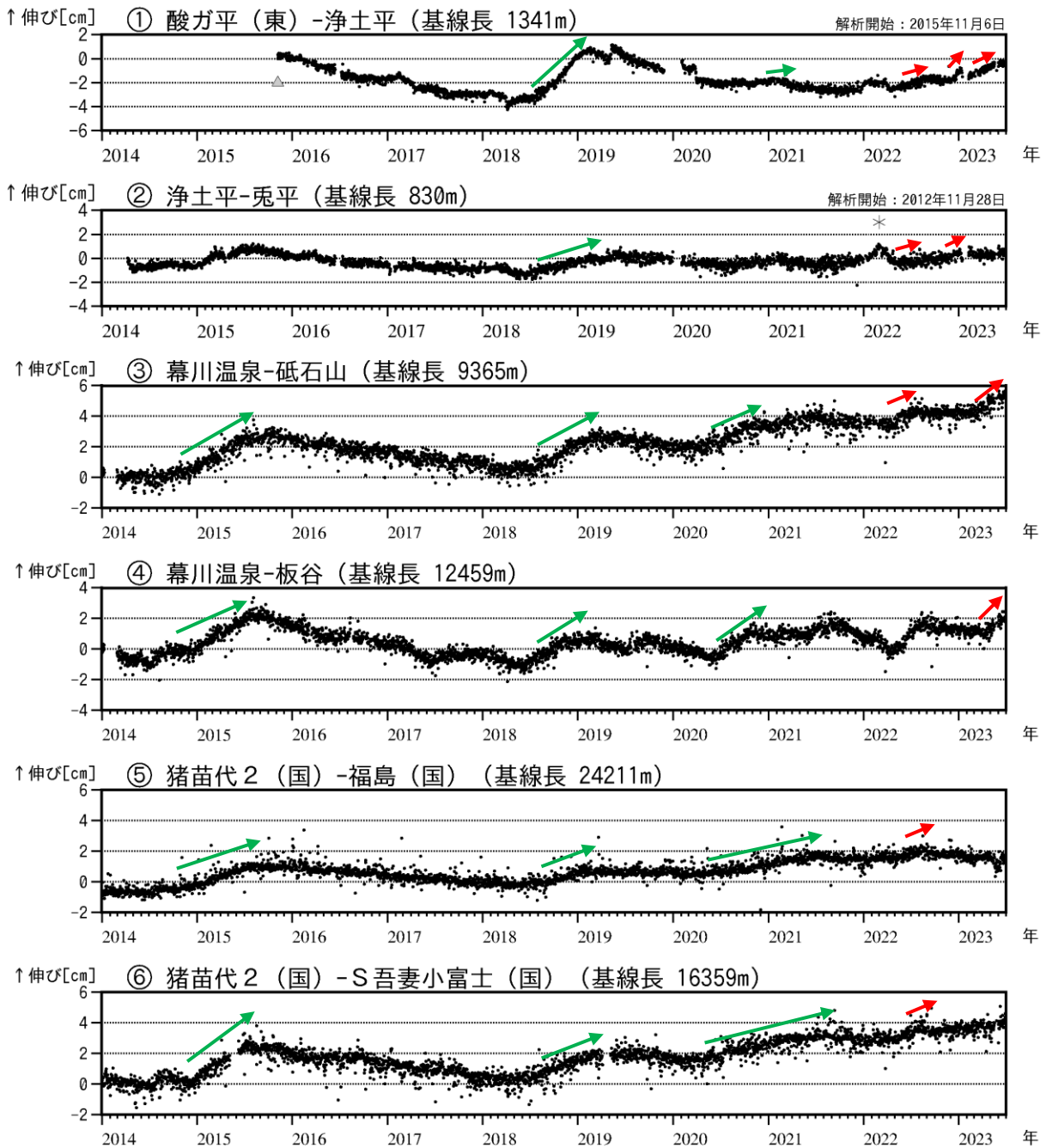
図3 吾妻山 吾妻山浅部・深部の地殻変動（2014年1月～2023年6月）
