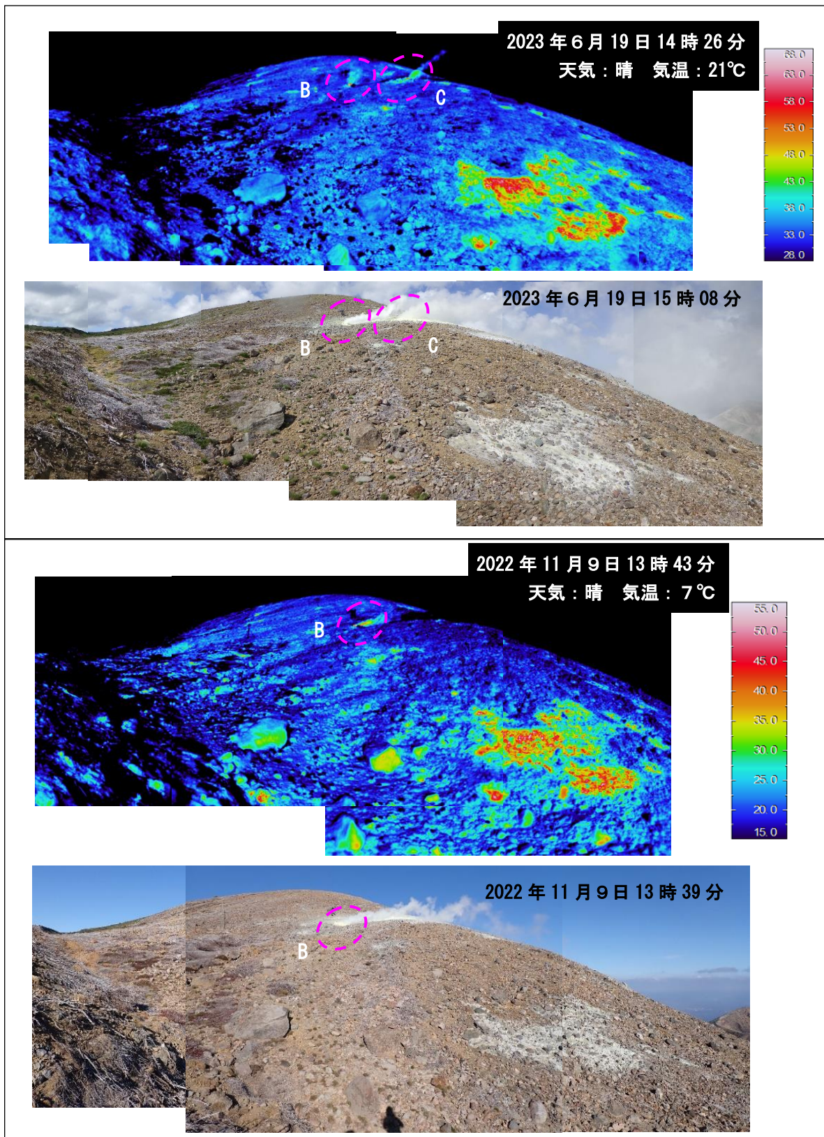
図8 吾妻山 大穴火口北西の状況（下）と地表面温度分布（上）
