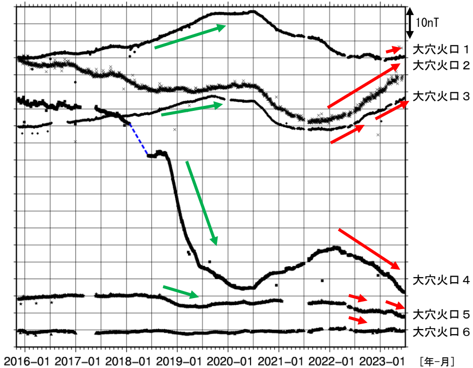
図 11 吾妻山 全磁力連続観測点の全磁力値変化（2015年11月～2023年6月）
