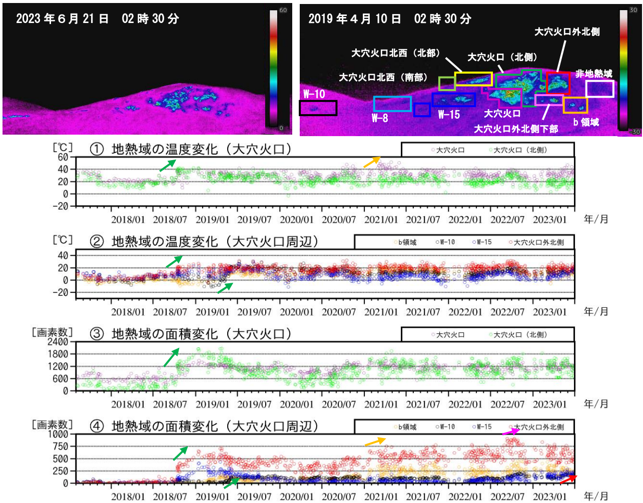
図4 吾妻山 監視カメラによる大穴火口周辺の地熱域の経過（2017年8月～2023年6月）
