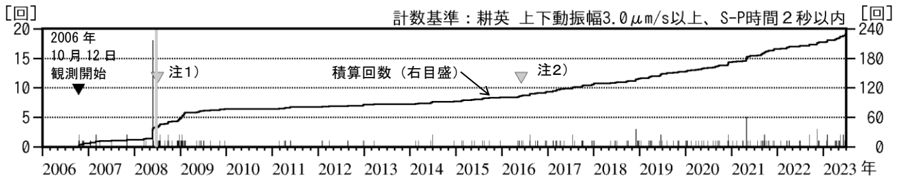
図3 栗駒山 日別地震回数（2006年10月～2023年6月）
