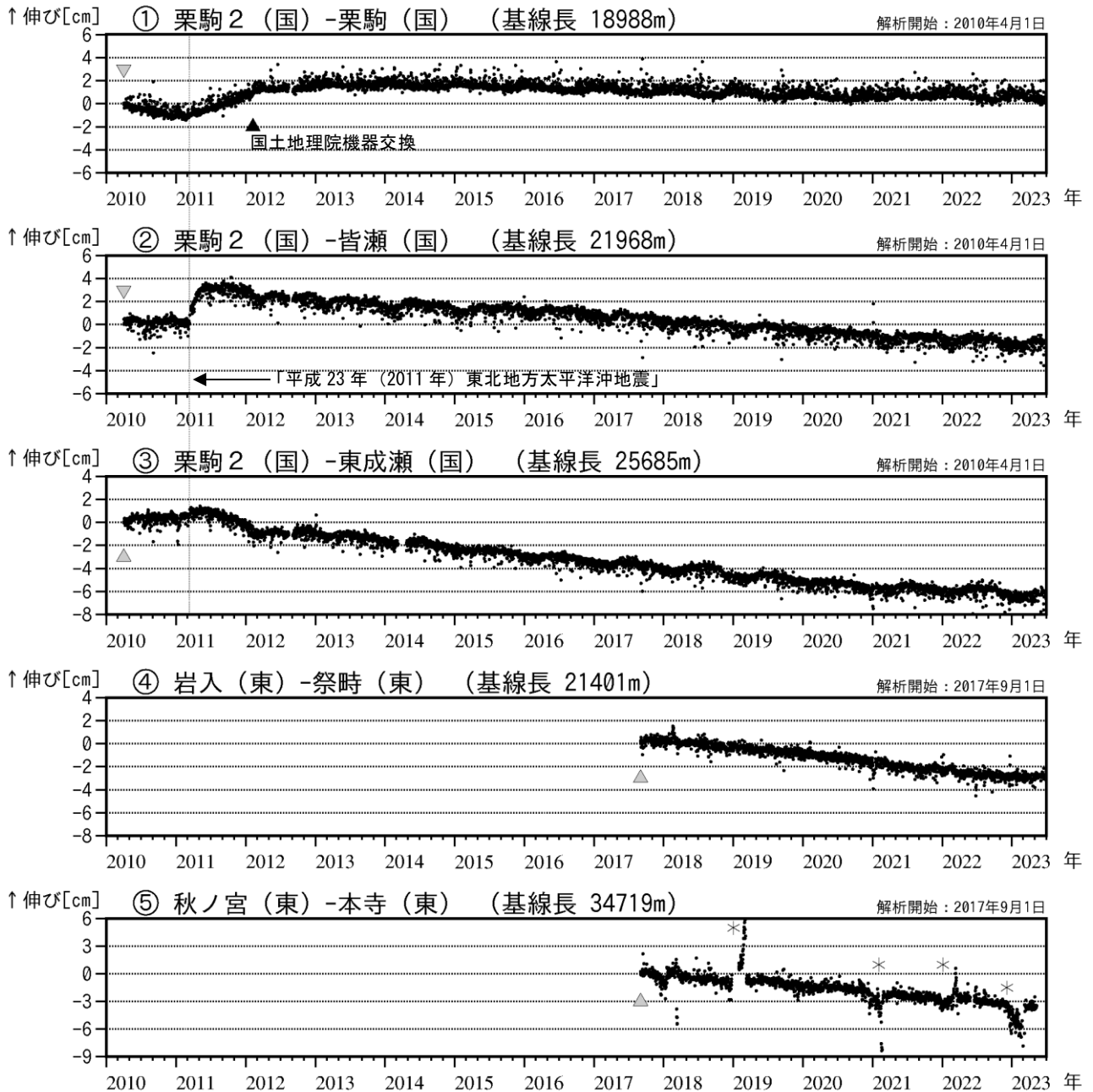
図4 栗駒山 GNSS 基線長変化図（2010年4月～2023年6月）
