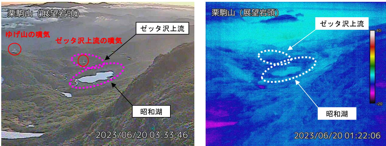
図2 栗駒山 昭和湖及びゼッタ沢上流周辺の状態（6月20日）
