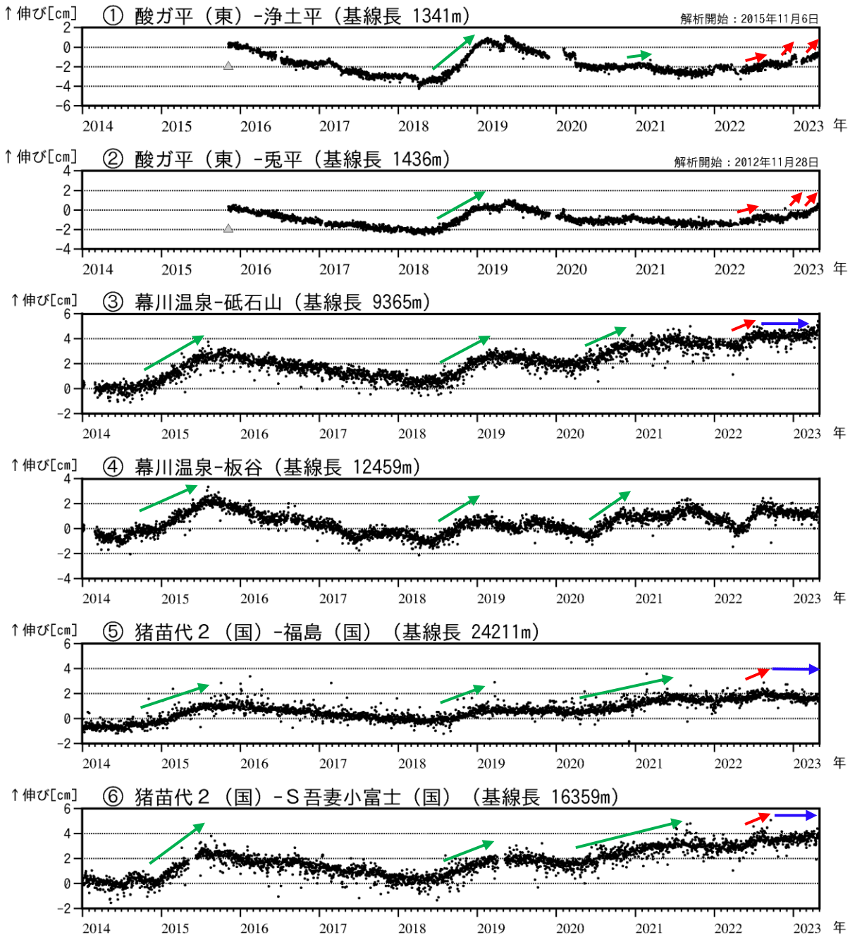
図3 吾妻山 吾妻山浅部・深部の地殻変動（2014年1月～2023年4月）
