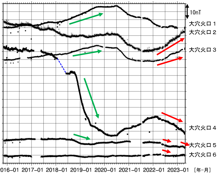
図7 吾妻山 全磁力連続観測点の全磁力値変化（2015年11月～2023年4月）
