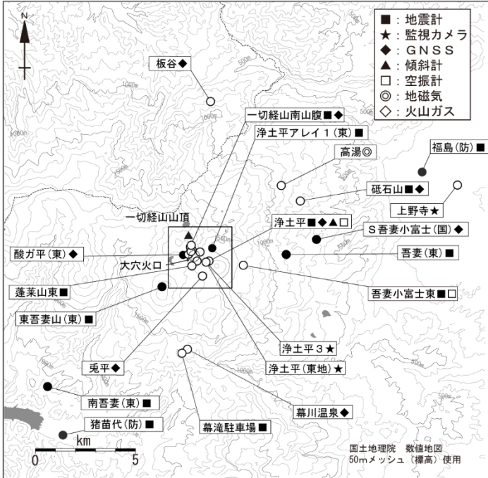
図9 吾妻山 観測点配置図
