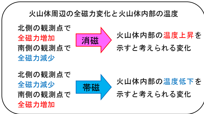
図8 熱消磁に伴う全磁力変化のモデル
