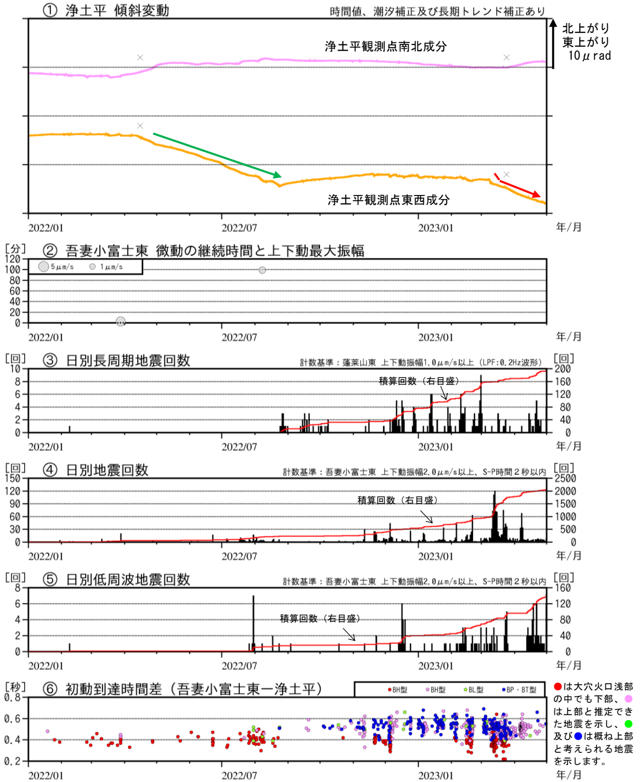
図2 吾妻山 火山活動経過図（2022年1月～2023年4月）
