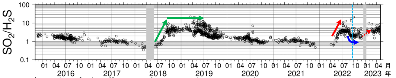
図6 吾妻山 火山ガス観測装置による観測（2015年11月～2023年4月）
