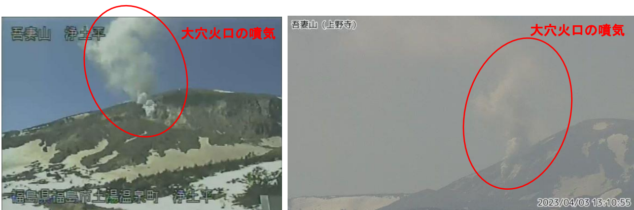
図5 吾妻山 大穴火口周辺の噴気の状態（4月3日）
