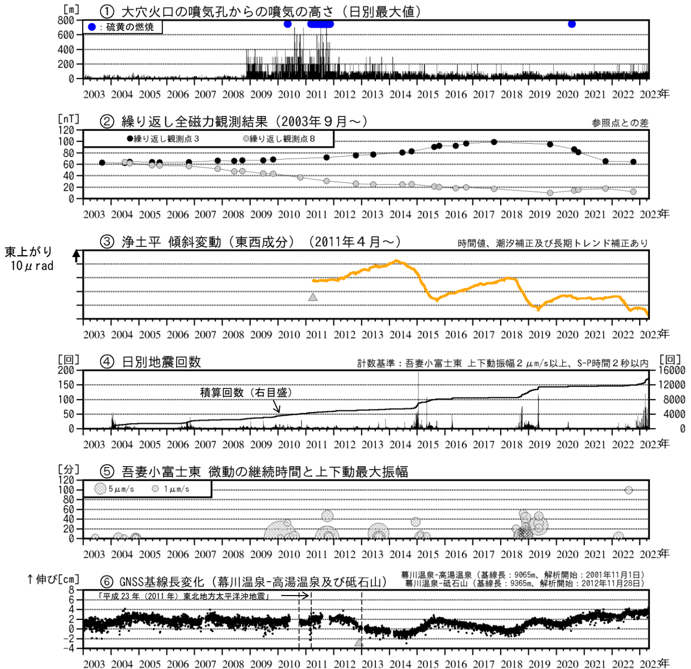
図1 吾妻山 中期的な火山活動の経過（2003年1月～2023年4月）
