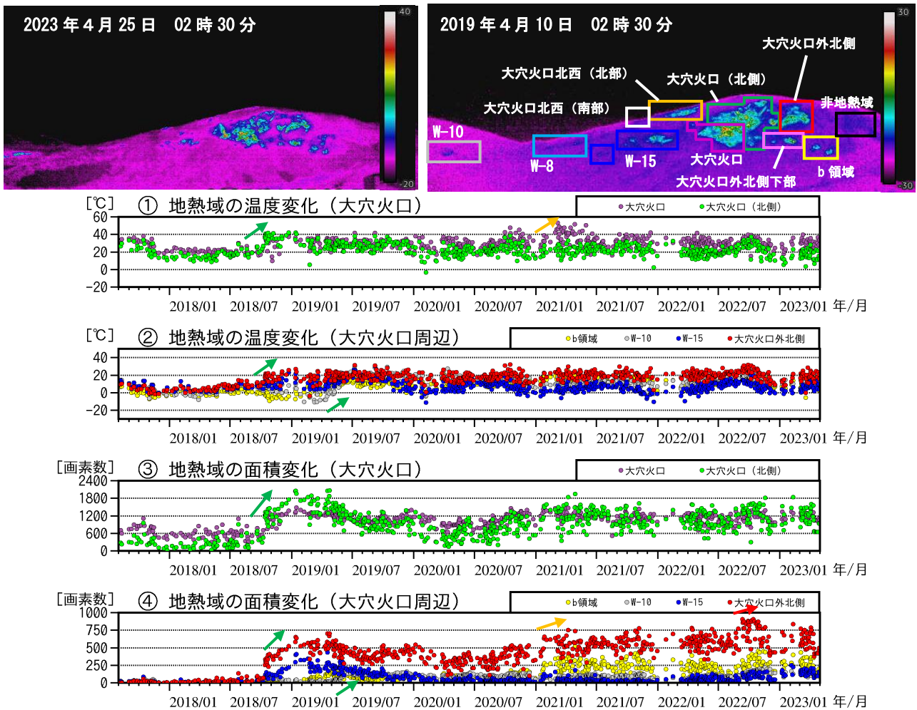
図4 吾妻山 監視カメラによる大穴火口周辺の地熱域の経過（2017年8月～2023年4月）
