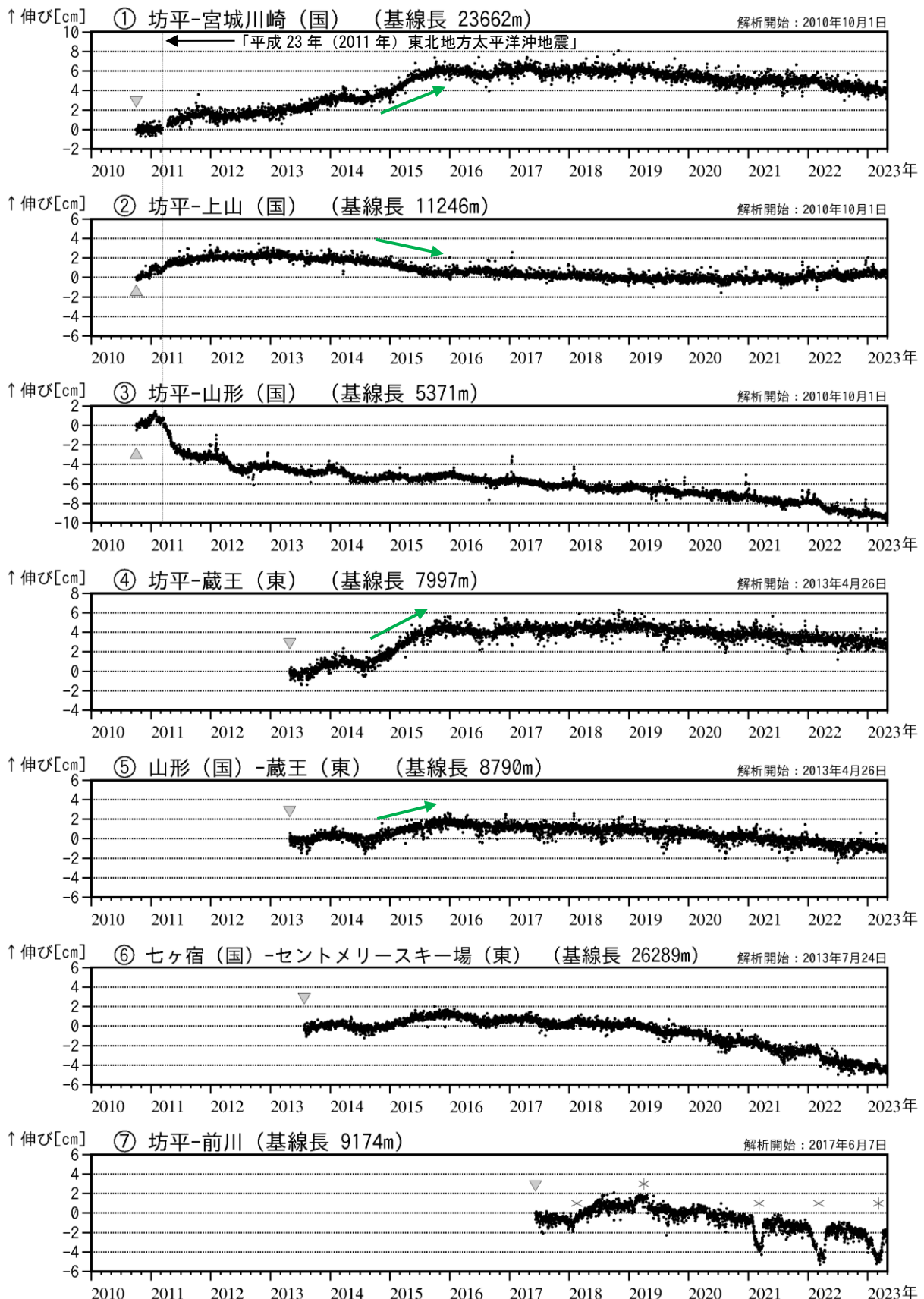
図3 蔵王山 GNSS 基線長変化図（2010年10月～2023年4月）
