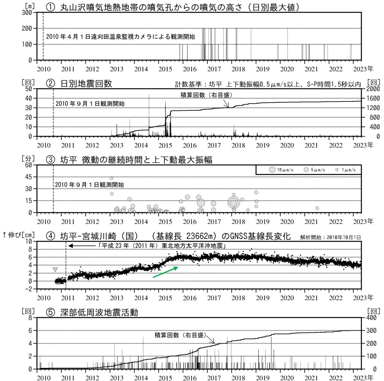
図2 蔵王山 火山活動経過図（2010年4月～2023年4月）
