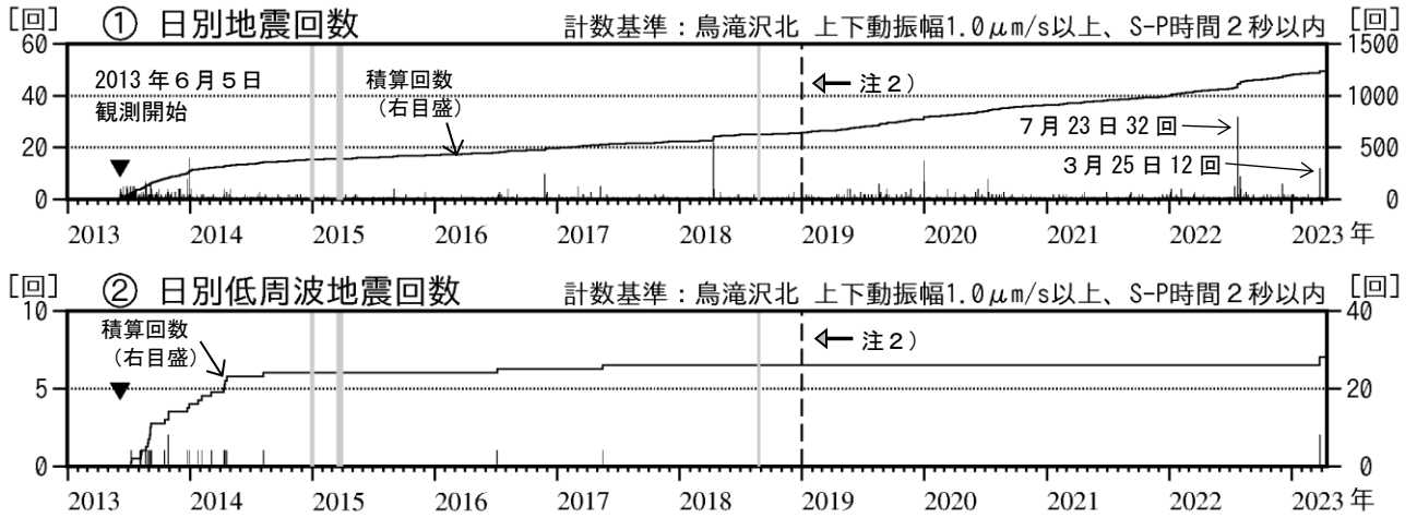
図2 八甲田山 日別地震回数（2013年6月～2023年3月）
