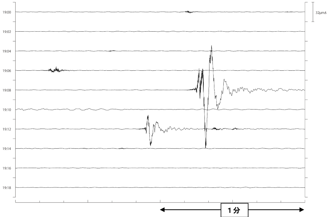
図3 八甲田山 酸ヶ湯（東北大学）観測点（上下成分）での低周波地震等の発生状況（2023年3月25日19時00分～19時20分）
