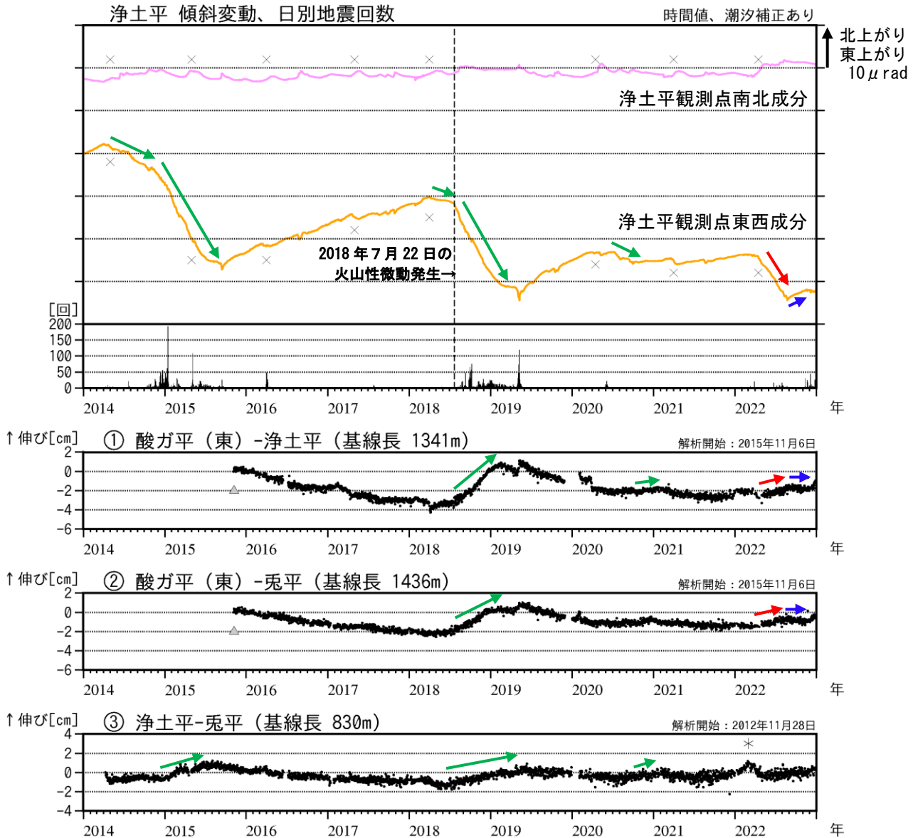
図6 吾妻山 大穴火口浅部の地殻変動（2014年1月～2022年12月）
