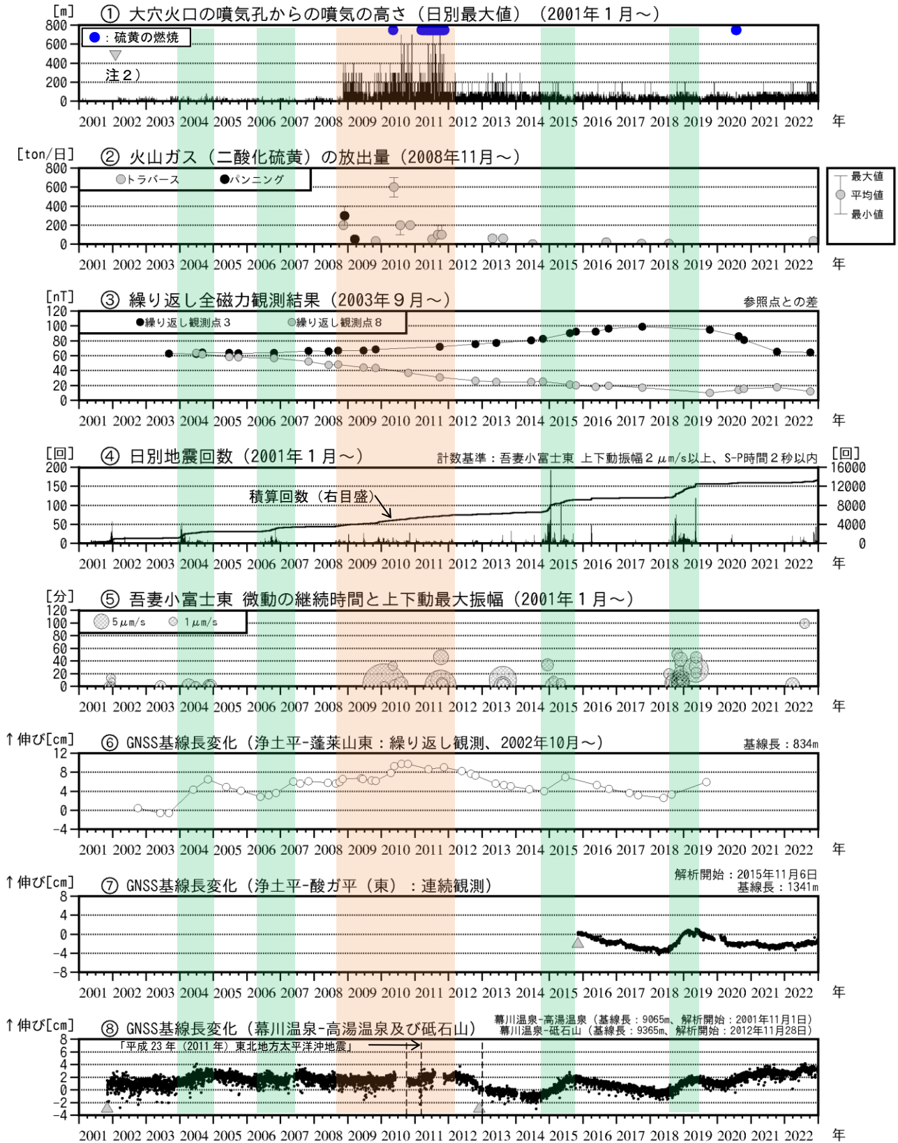
図2 吾妻山 中期的な火山活動の経過（2001年1月～2022年12月）
