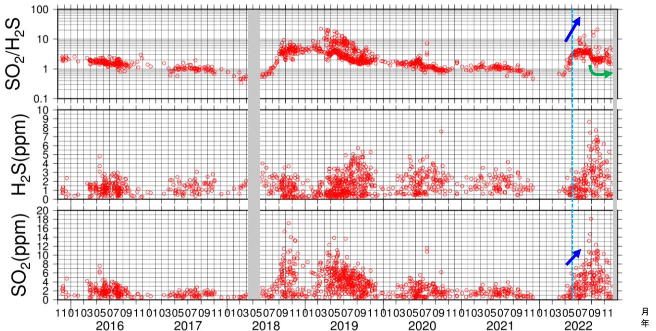
図10 吾妻山 火山ガス観測装置による観測（2015年11月～2022年12月）
