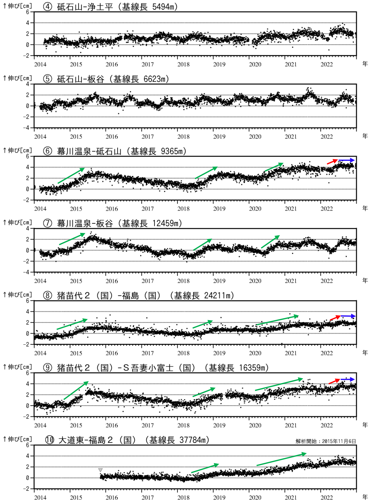
図7 吾妻山 吾妻山深部の地殻変動（2014年1月～2022年12月）
