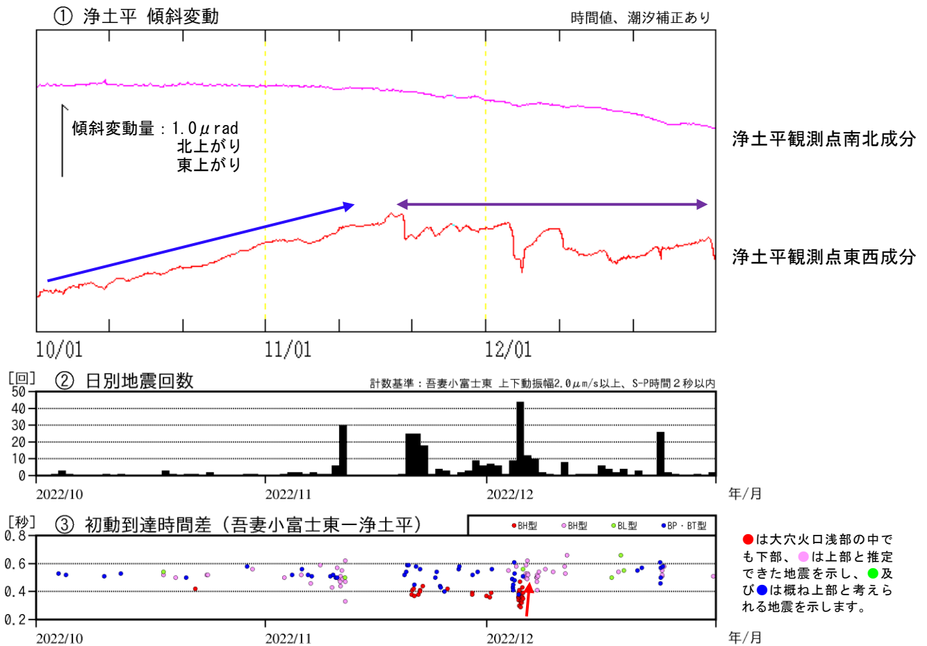
図4 吾妻山 浄土平観測点での傾斜変動と吾妻山の地震活動の推移（2022年10月～2022年12月）
