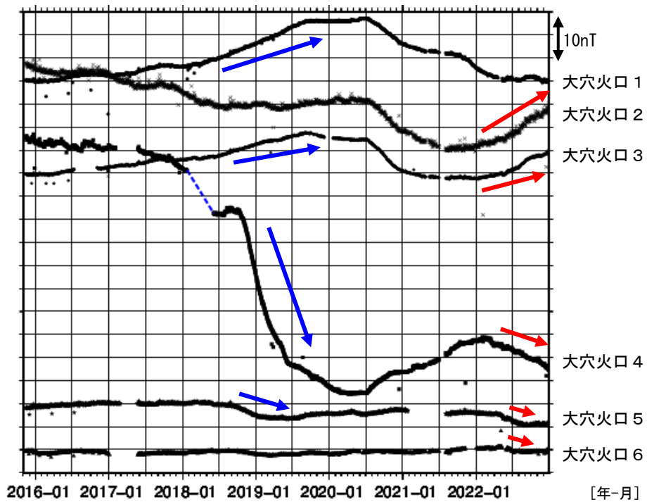
図 12 吾妻山 全磁力連続観測点の全磁力値変化 (2015年11月~2022年12月)
