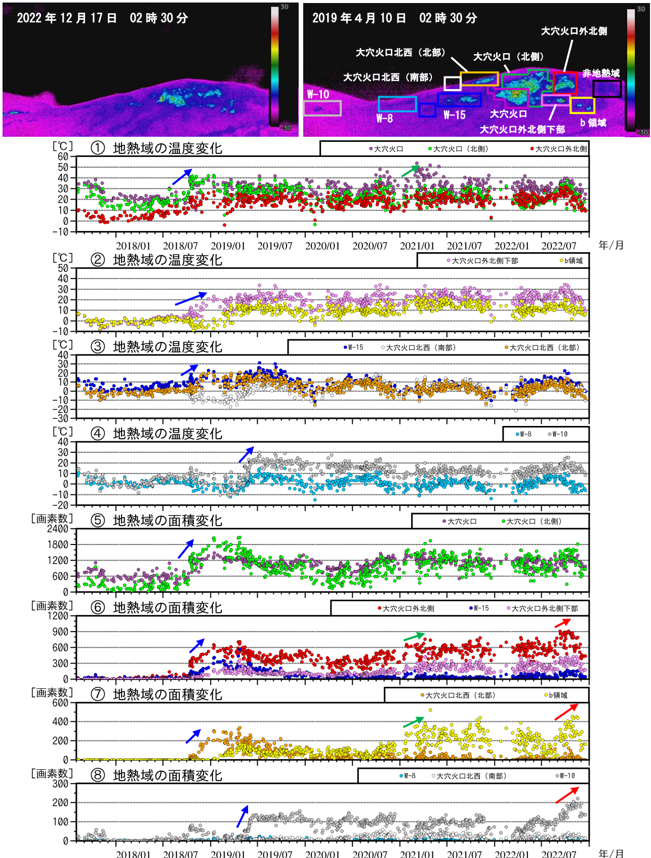
図8 吾妻山 監視カメラによる大穴火口周辺の地熱域の経過（2017年8月～2022年12月）
