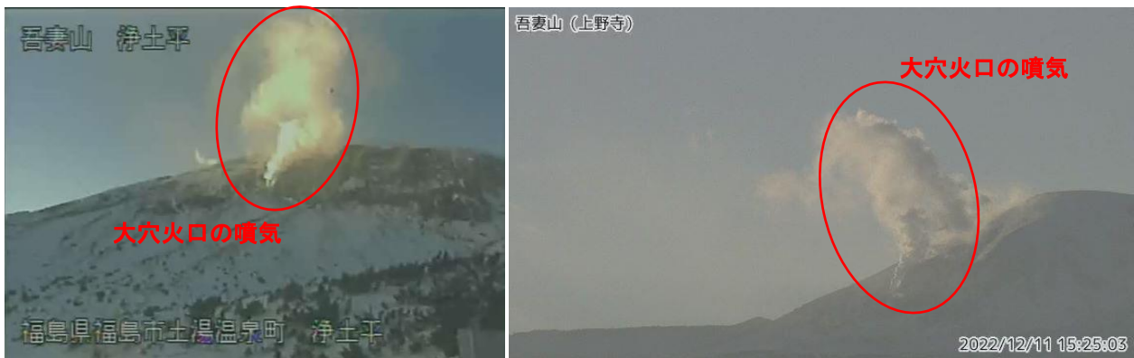
図9 吾妻山 大穴火口周辺の噴気の状態（12月11日）
