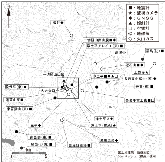
図14 吾妻山 観測点配置図
