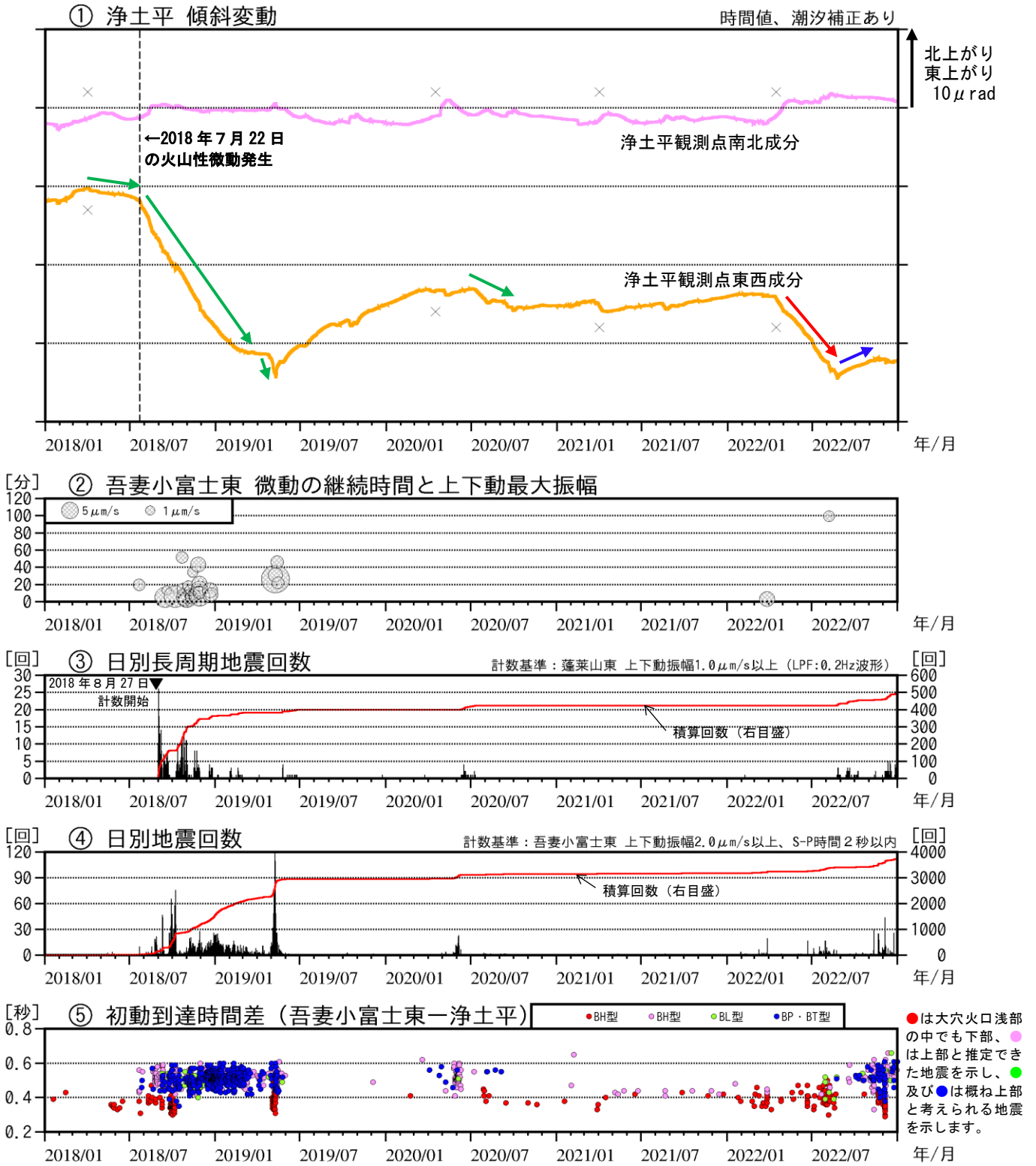
図3 吾妻山 火山活動経過図 (2018年1月～2022年12月)
